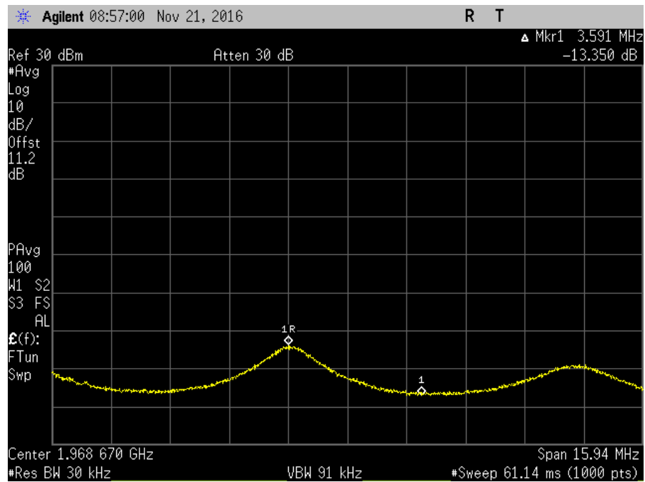
7.11.3_Osc_DL_1930-1995MHz+2_AWGNL
