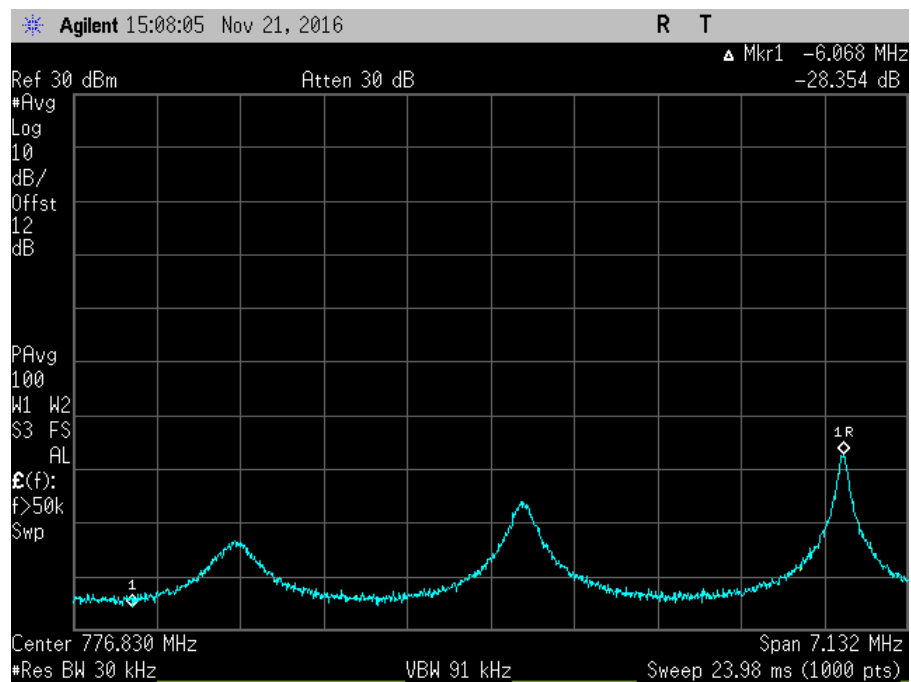
7.11.3_Osc_UL_776-787MHz-2_AWGNR
