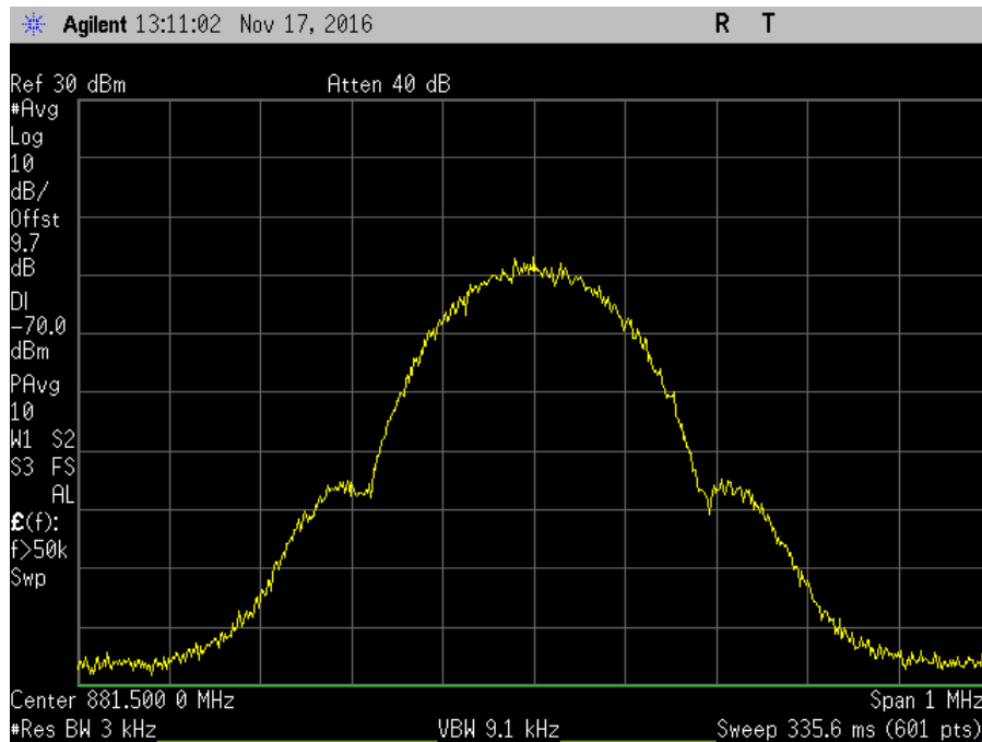
7.10_OBW_DL_869-894MHz_GSM_Out
