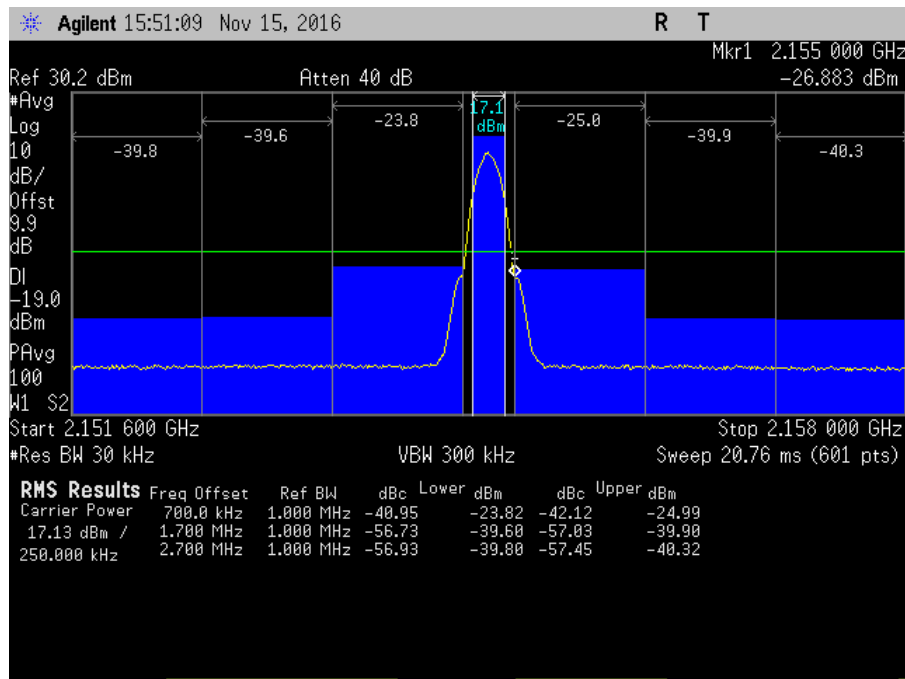
7.5_OBE_DL_2110-2155MHz_H_PreAGC_GSM
