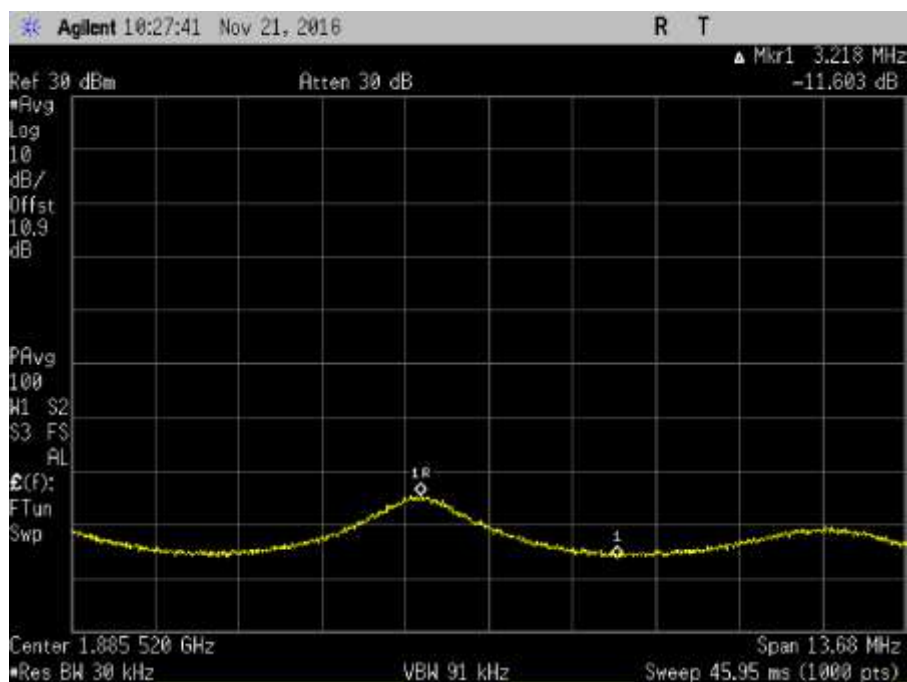
7.11.3_Osc_UL_1850-1915MHz+5_AWGNL
