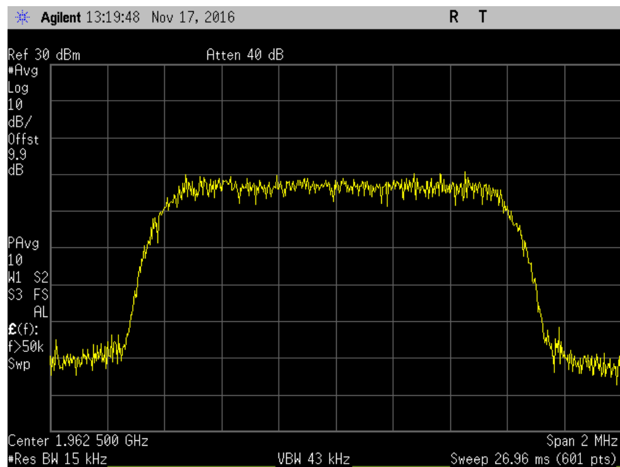
7.10_OBW_DL_1930-1995MHz_CDMA_Out
