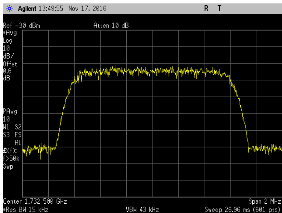
7.10_OBW_UL_1710-1755MHz_CDMA_In
