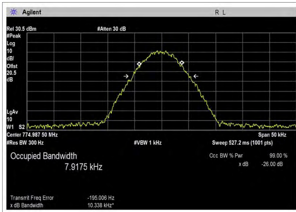
DL_775H-Out+10dB
