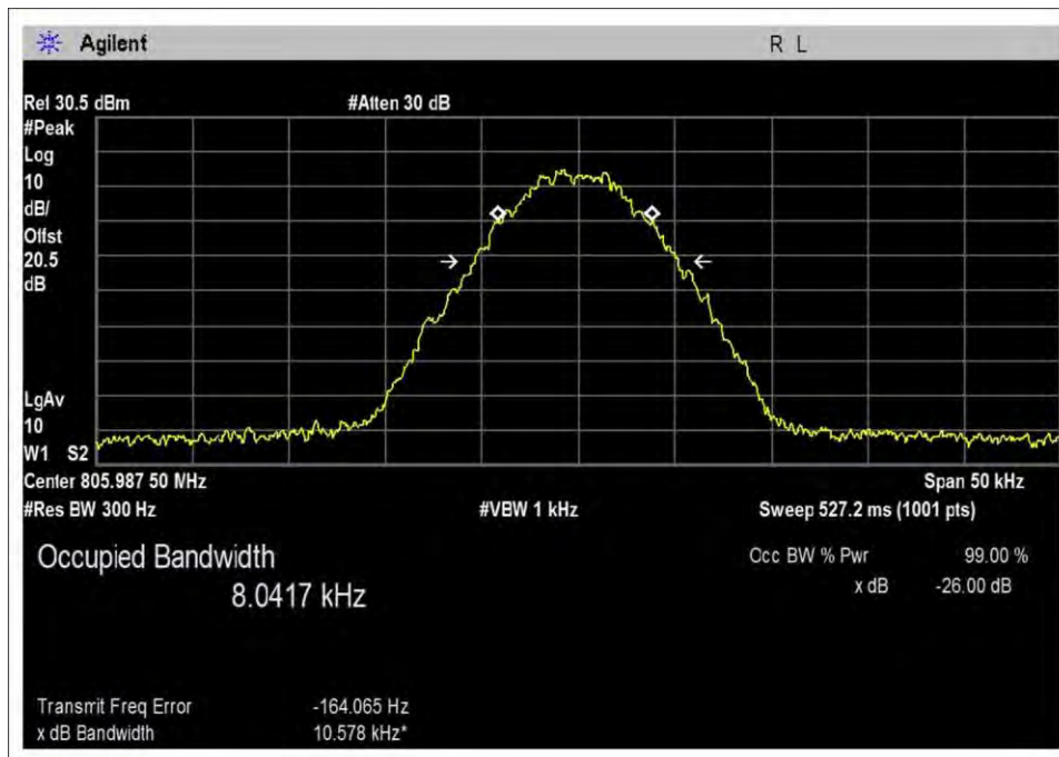
UL_805H-Out+10dB
