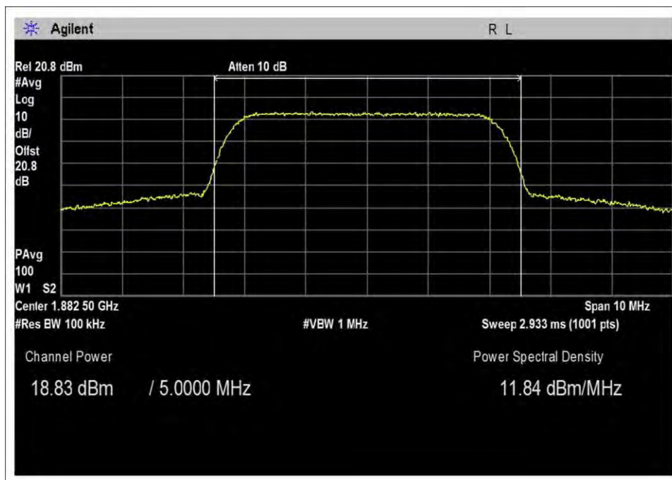
UL-1850-1915MHz-Out-AGC+3
