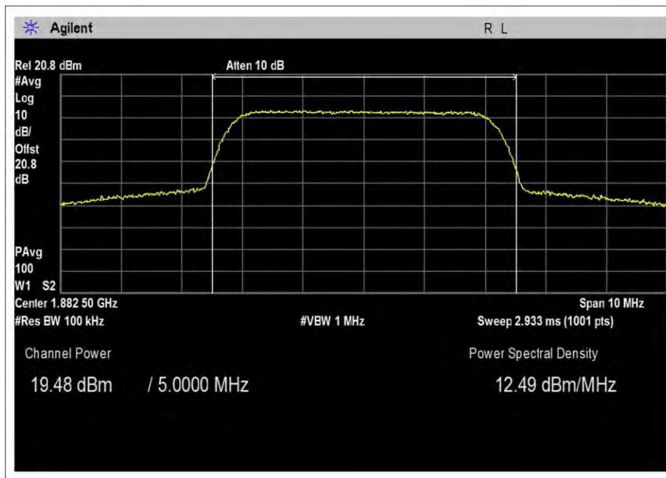
UL-1850-1915MHz-Out-41.8
