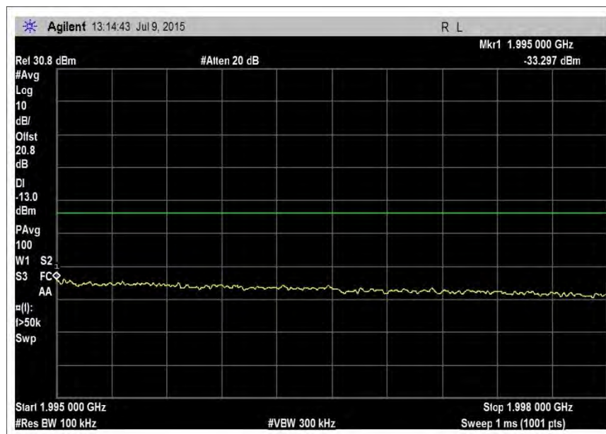
DL-1930-1995H-Cm-AGC+3
