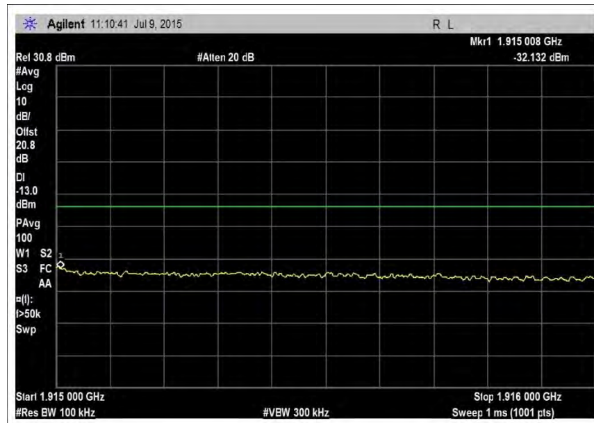
UL-1850-1915H-Cm-preAGC
