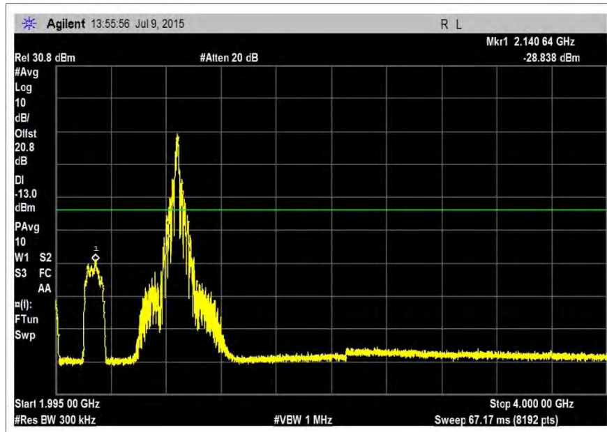
DL-1930-1995R-AWGN-L
