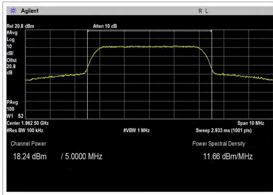
DL-1930-1995MHz-Out-AGC+3
