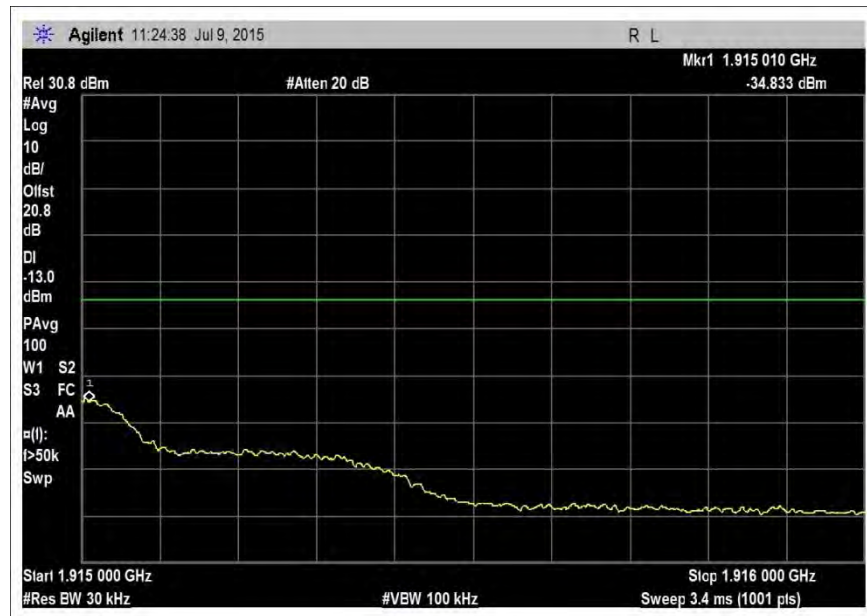
UL-1850-1915H-Cm-preAGC
