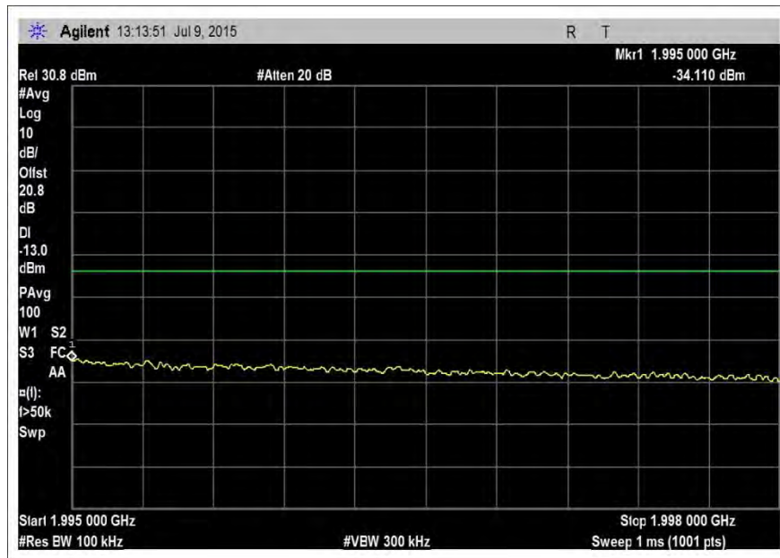
DL-1930-1995H-Cm-preAGC
