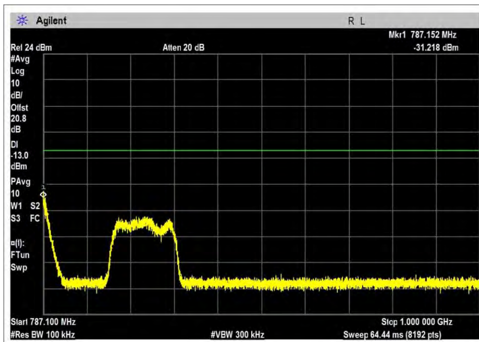
UL-776-787R-AWGN-H
