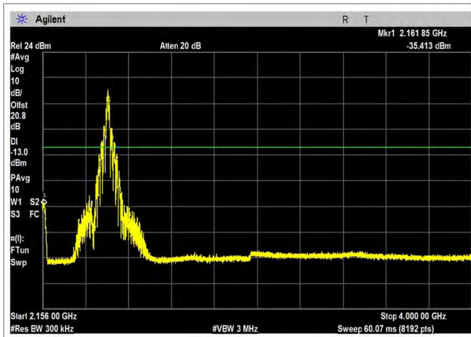
DL-2110-2155R-GSM-M
