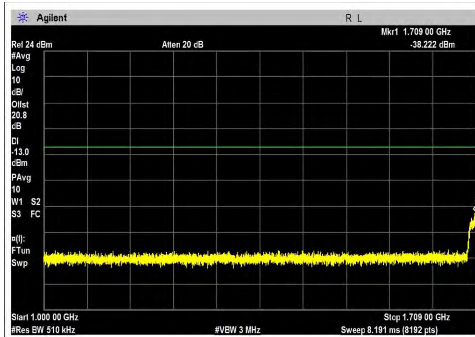
UL-1710-1755L-GSM-M
