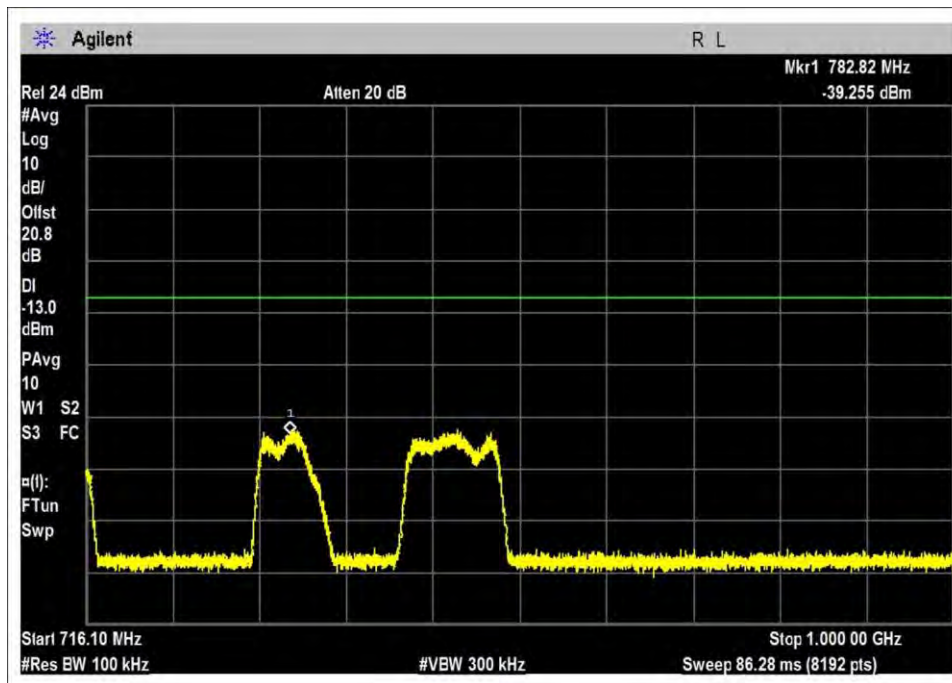
UL-698-716R-GSM-L
