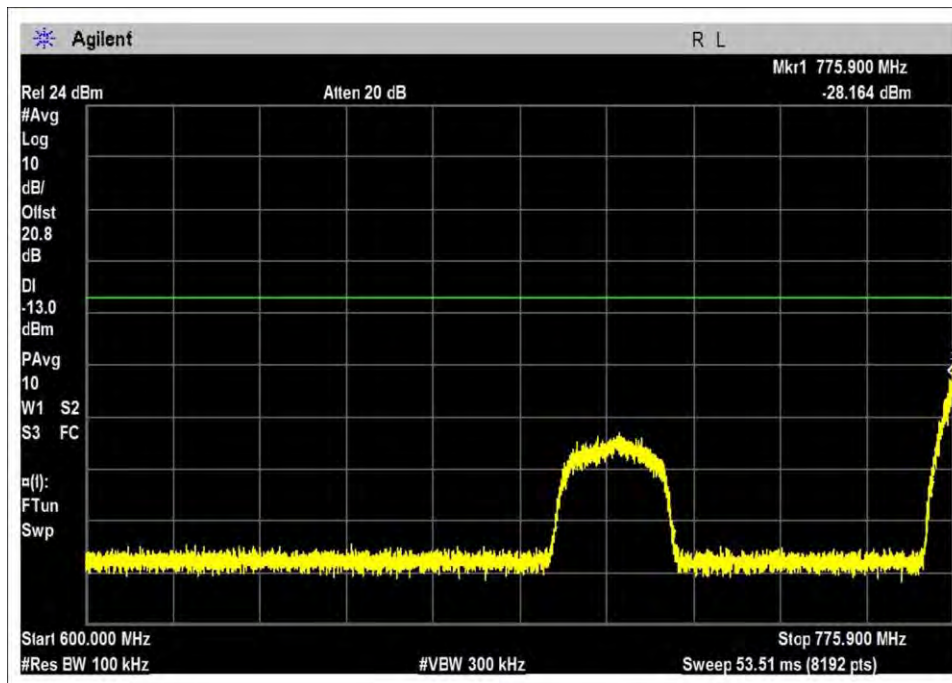
UL-776-787L-AWGN-L
