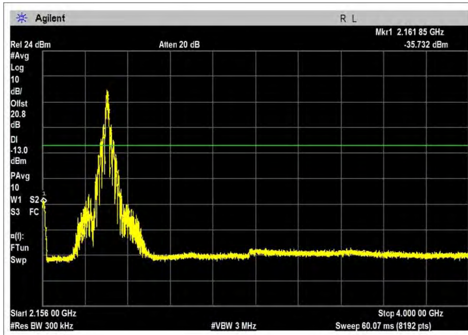
DL-2110-2155R-GSM-L
