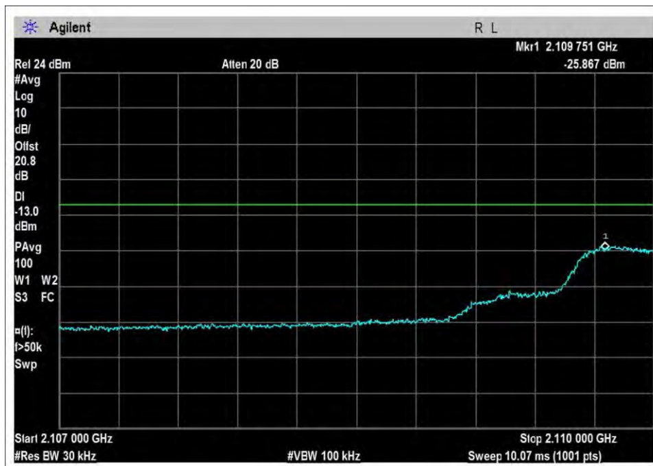
DL-2110-2155L-Cm-preAGC
