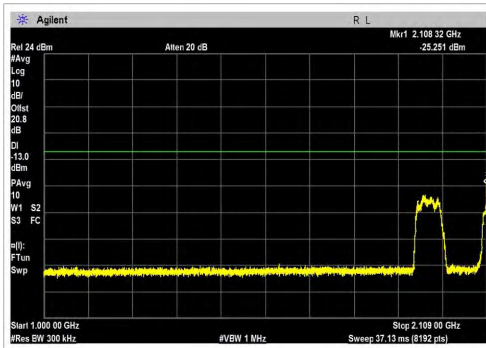
DL-2110-2155L-AWGN-L
