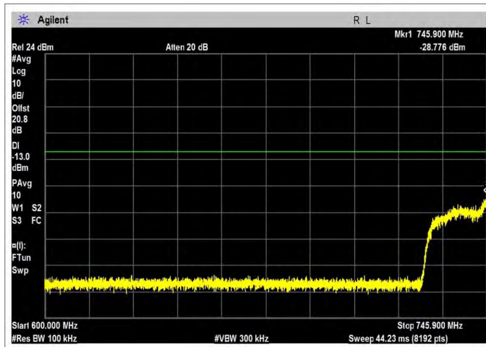
DL-746-757L-AWGN-L
