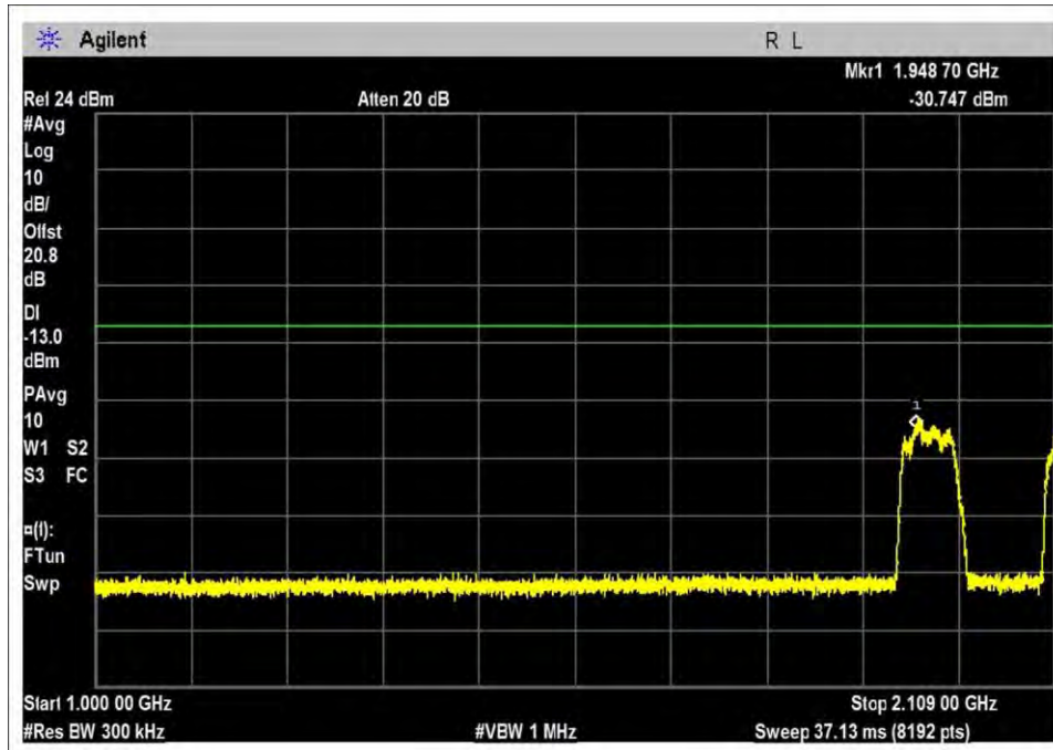
DL-2110-2155L-AWGN-M
