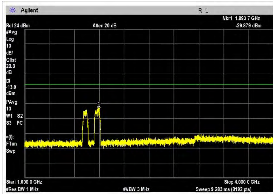
UL-776-787-AWGN-M
