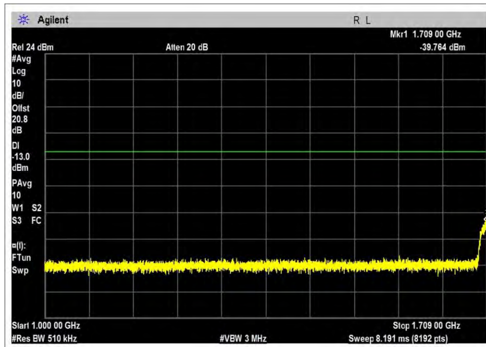
UL-1710-1755L-GSM-L
