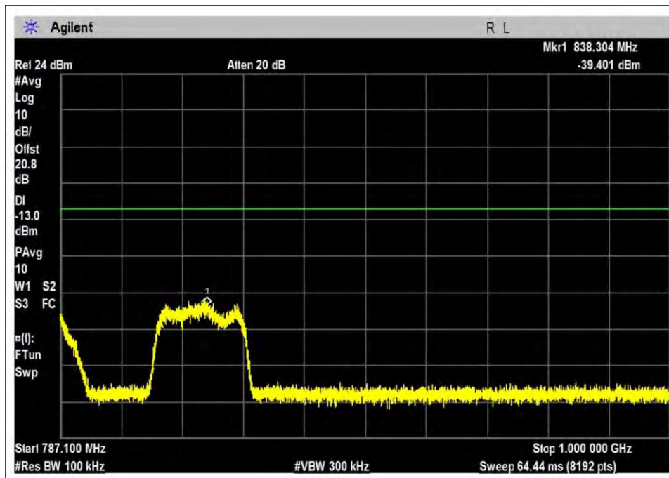
UL-776-787R-AWGN-L
