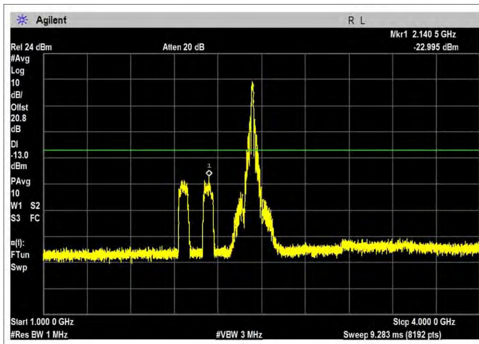
DL-728-746-AWGN-M
