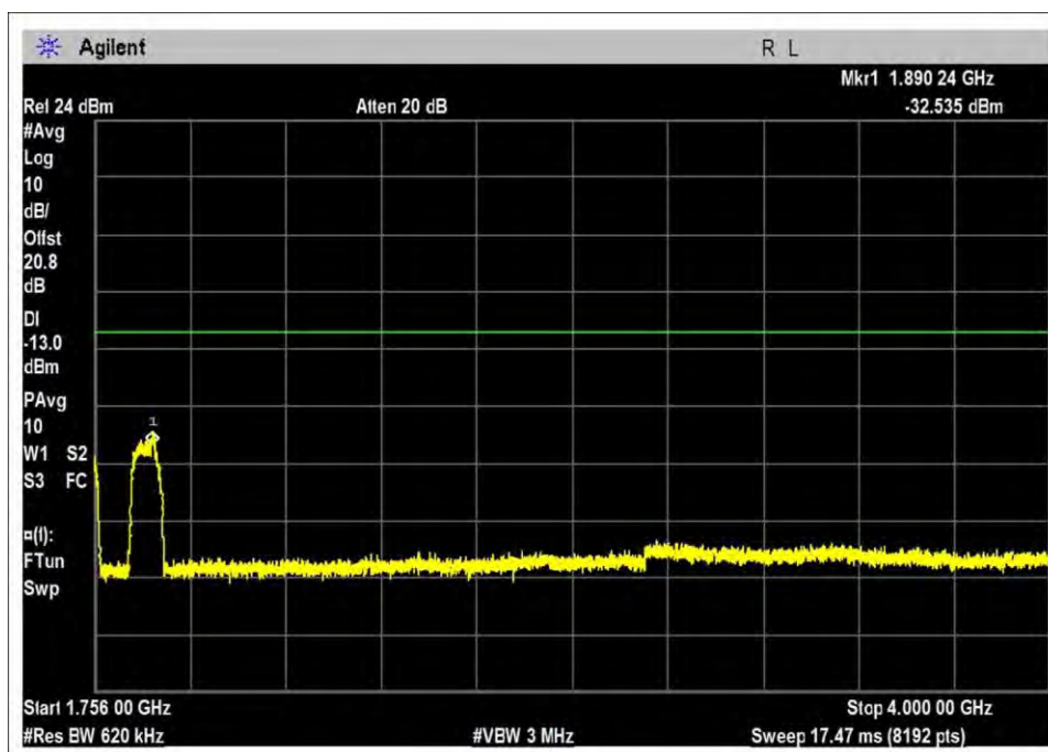
UL-1710-1755R-AWGN-M
