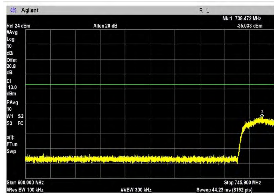
DL-746-757L-AWGN-M
