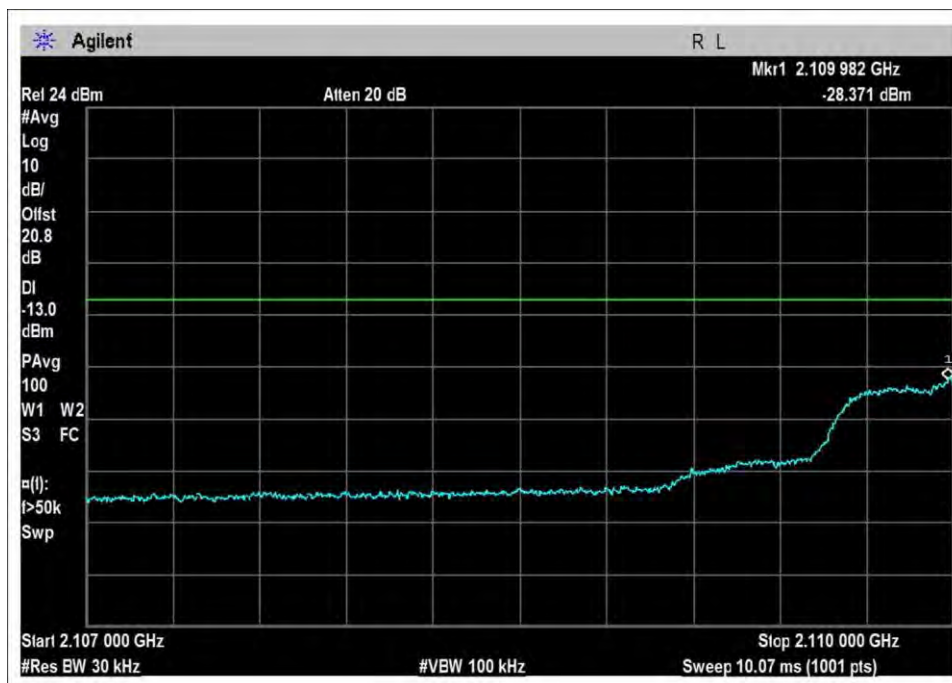
DL-2110-2155L-Cm-AGC+3
