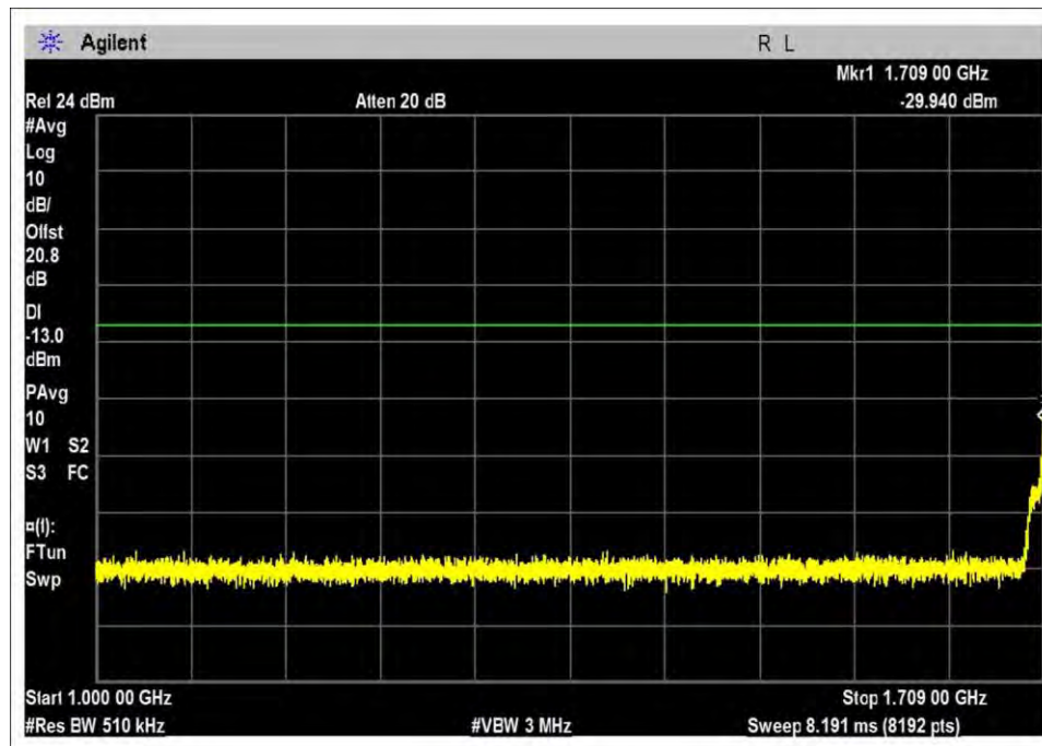
UL-1710-1755L-AWGN-L
