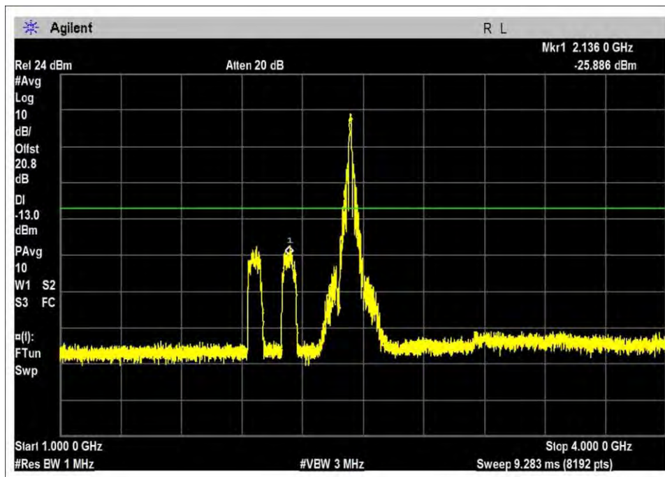
DL-728-746-AWGN-L
