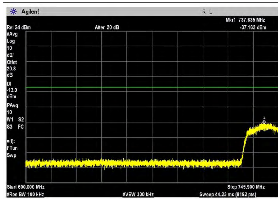
DL-746-757L-GSM-M
