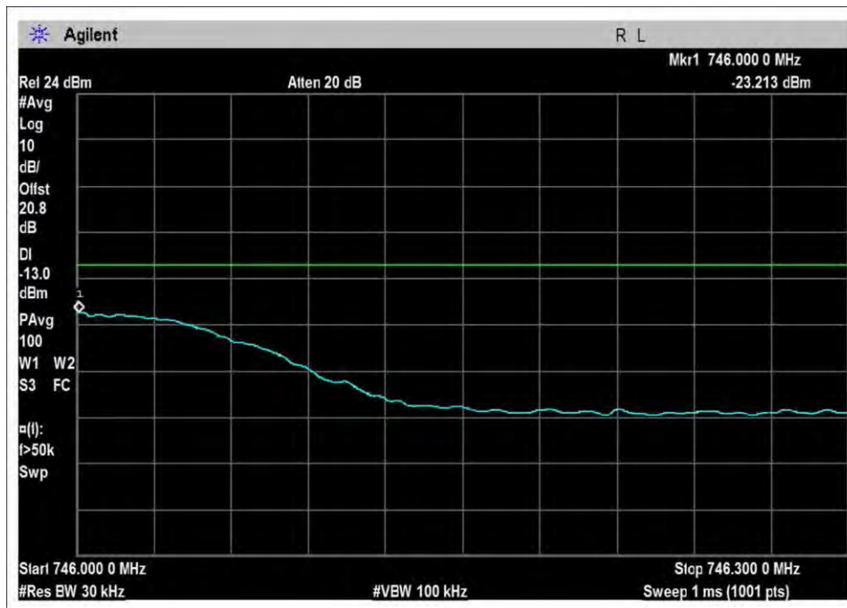
DL-728-746H-Sn-AGC+3
