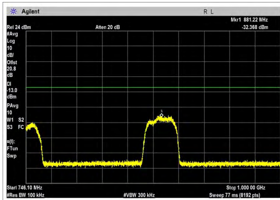
DL-728-746R-AWGN-L
