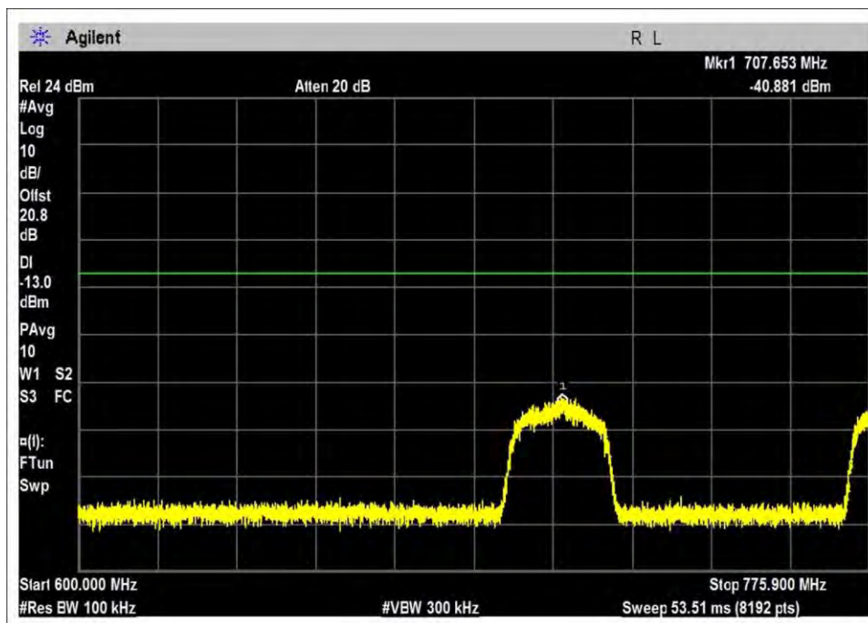
UL-776-787L-AWGN-H
