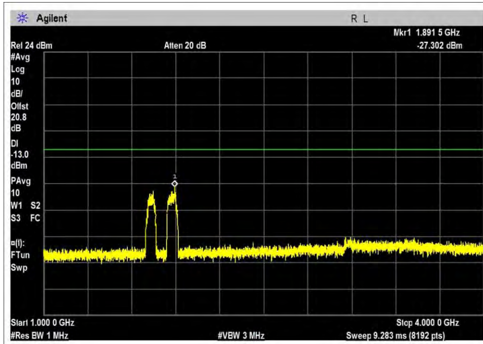
UL-776-787-GSM-M
