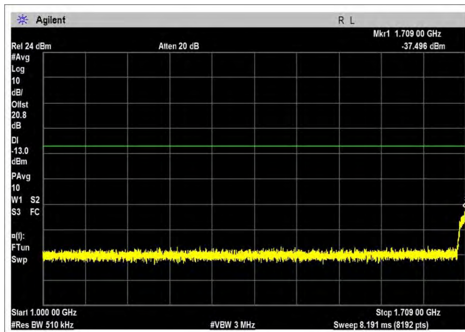
UL-1710-1755L-AWGN-M
