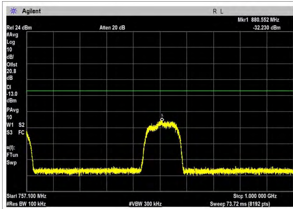
DL-746-757R-AWGN-M
