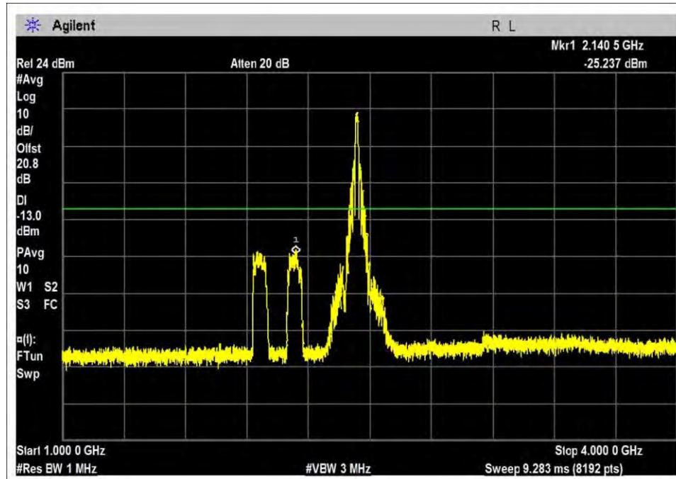
DL-746-757-GSM-M
