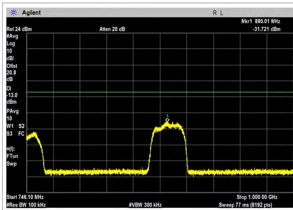
DL-728-746R-GSM-M
