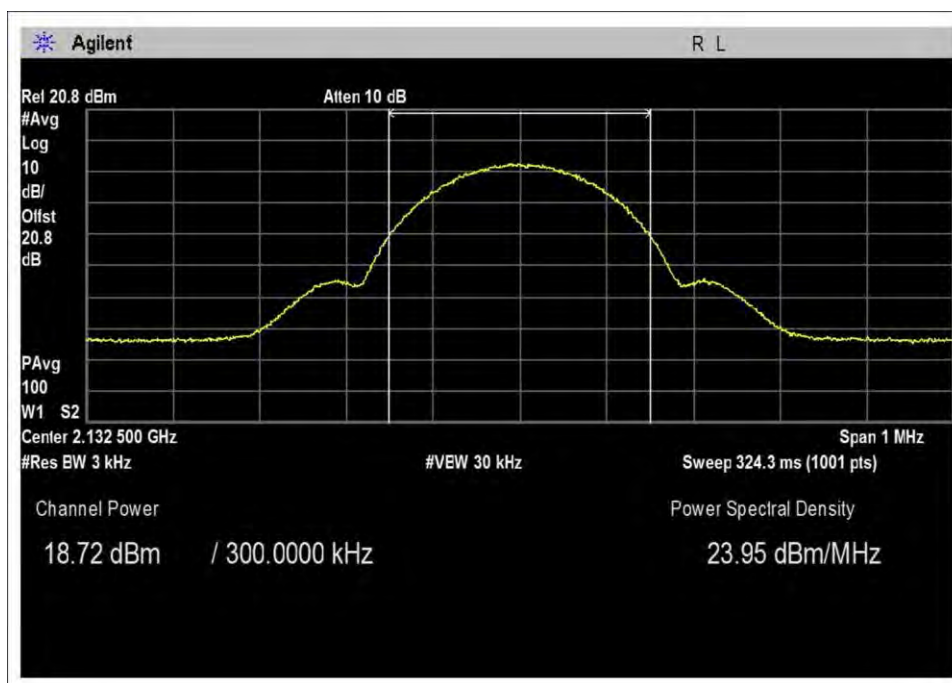
DL-2110-2155M-Out-46.2
