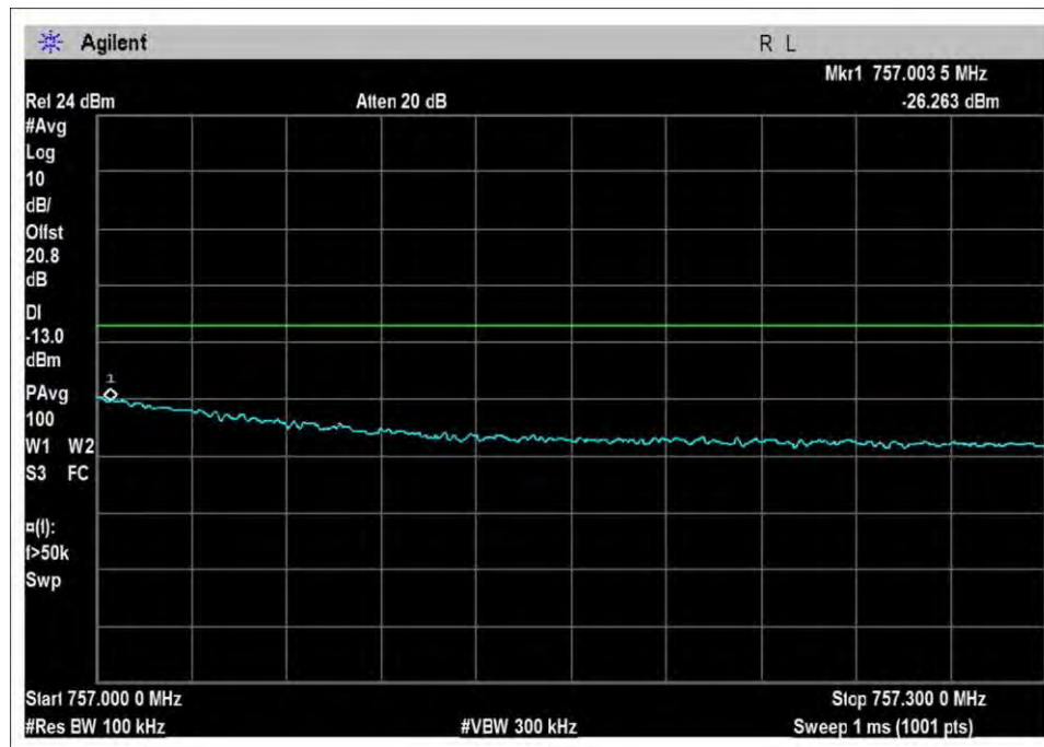
DL-746-757H-Sn-AGC+3
