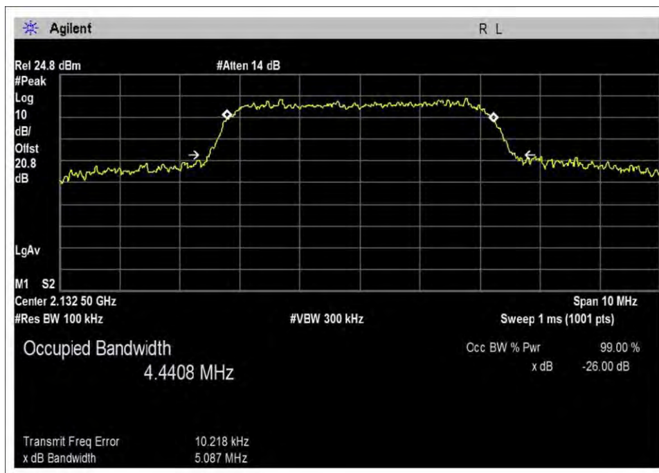
DL-2110-2155M-Out-46.8
