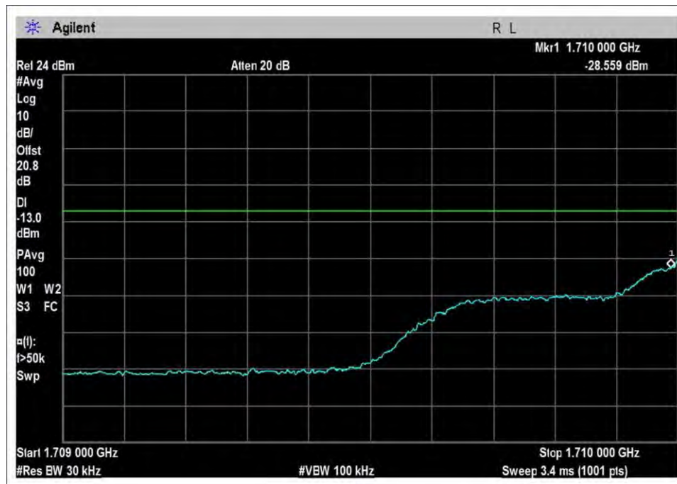
UL-1710-1755L-Cm-AGC+3
