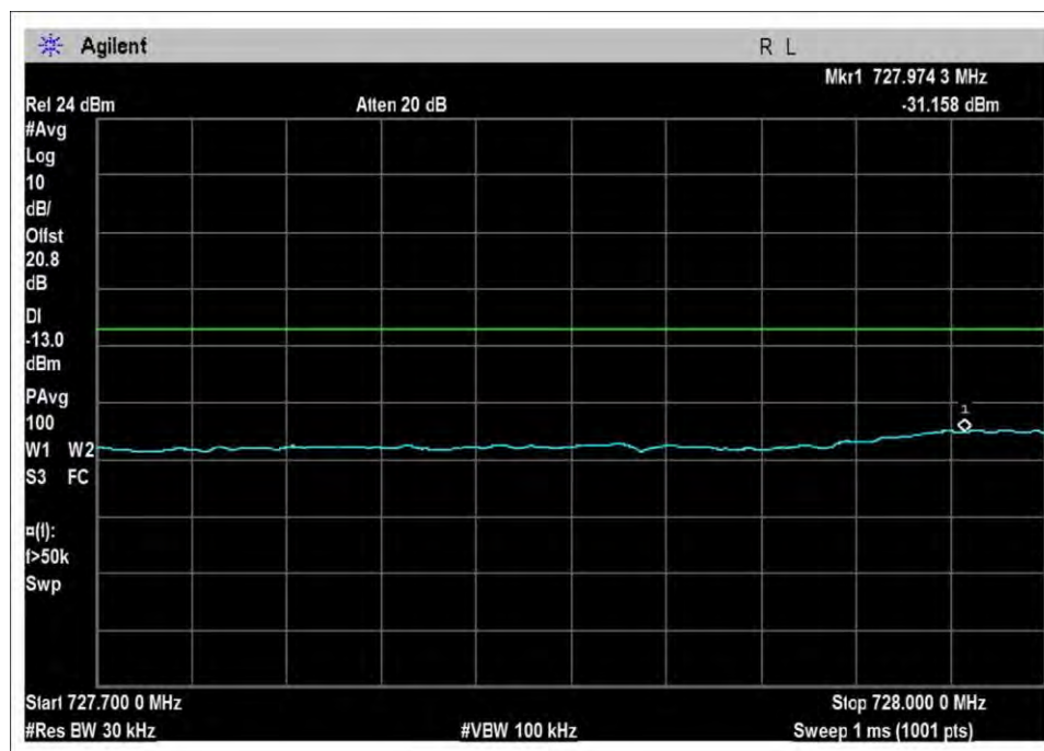
DL-728-746L-Cm-preAGC
