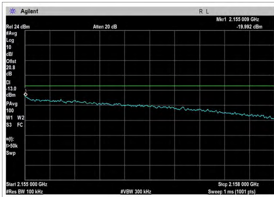
DL-2110-2155H-Sn-AGC+3
