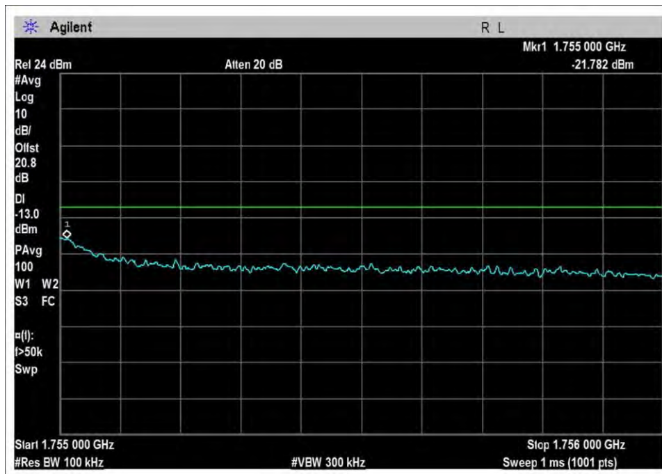
UL-1710-1755H-Sn-AGC+3
