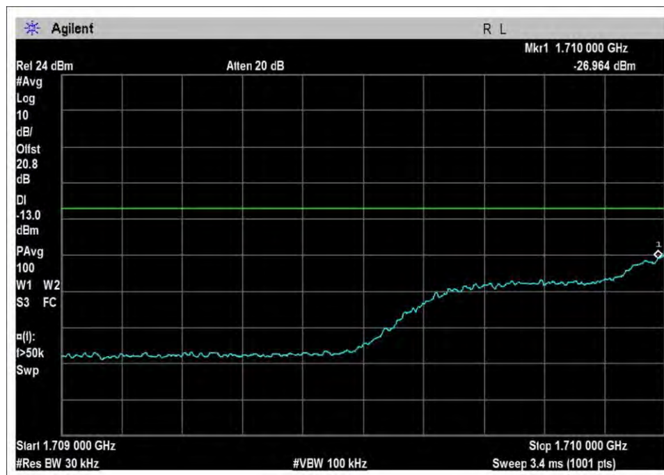
UL-1710-1755L-Cm-preAGC
