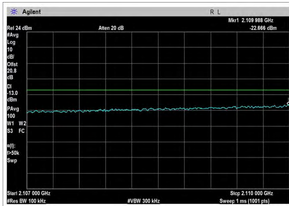
DL-2110-2155L-Cm-AGC+3
