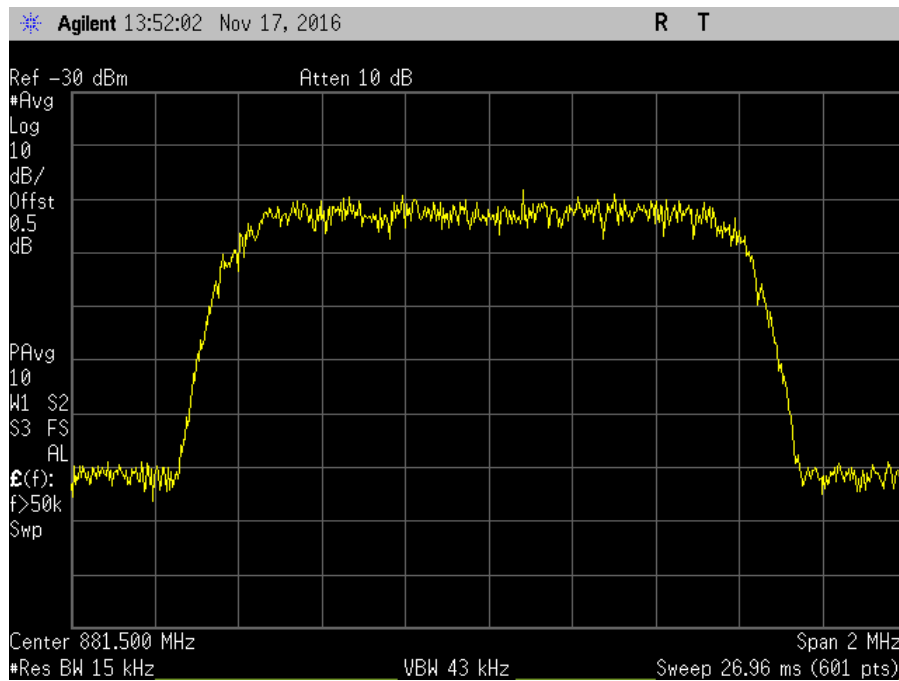
7.10_OBW_DL_869-894MHz_CDMA_In
