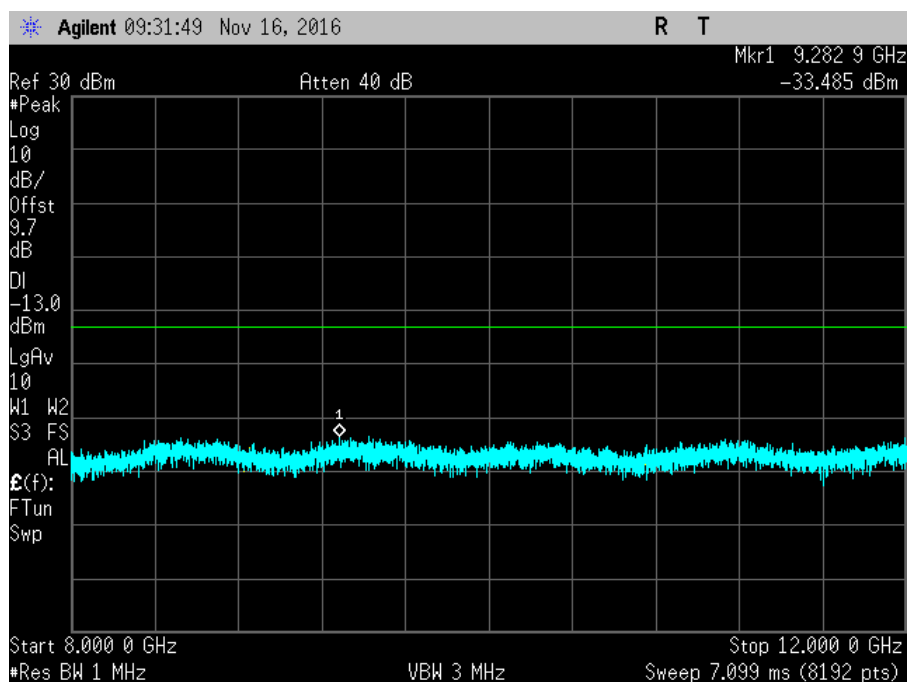
7.6_CSE_UL_824-849MHz_R3
