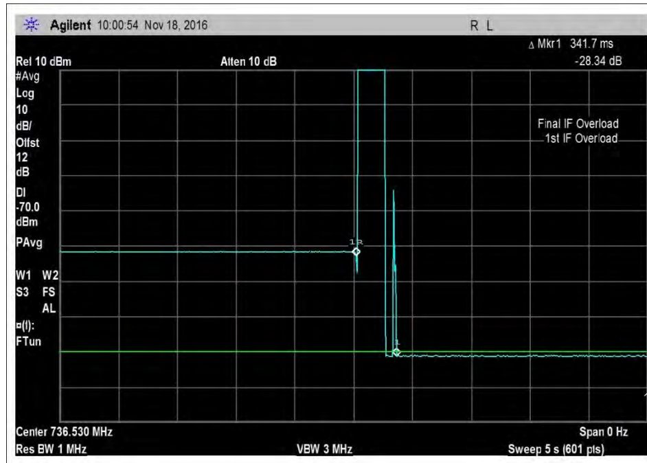
7.11_osc_DL-728-746MHz
