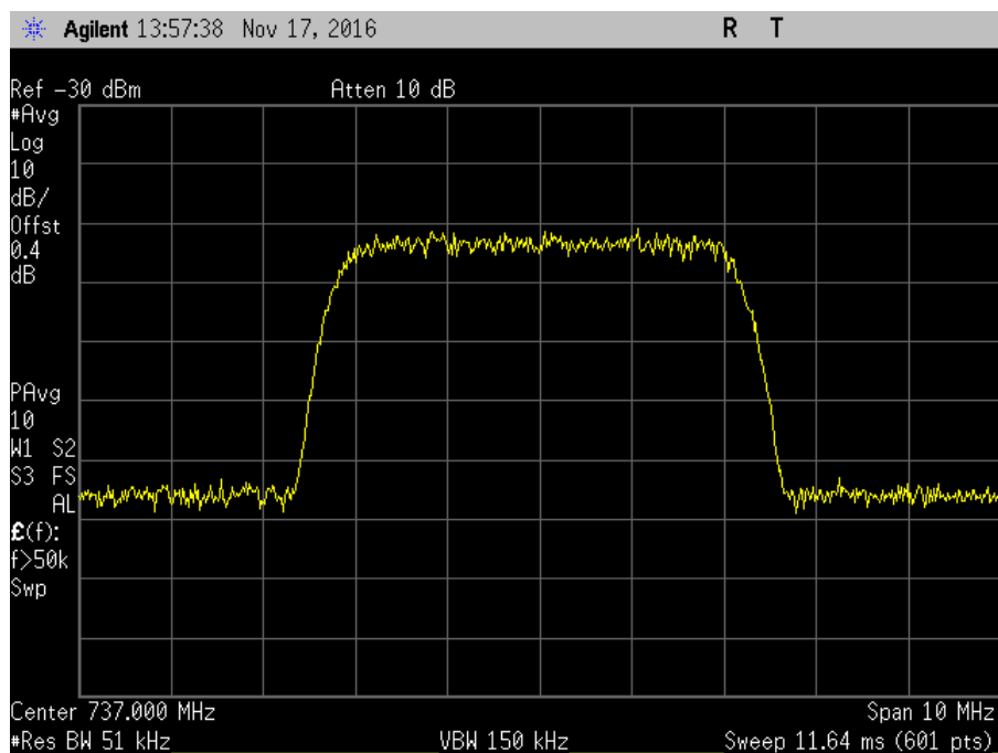
7.10_OBW_DL_728-746MHz_WCDMA_In
