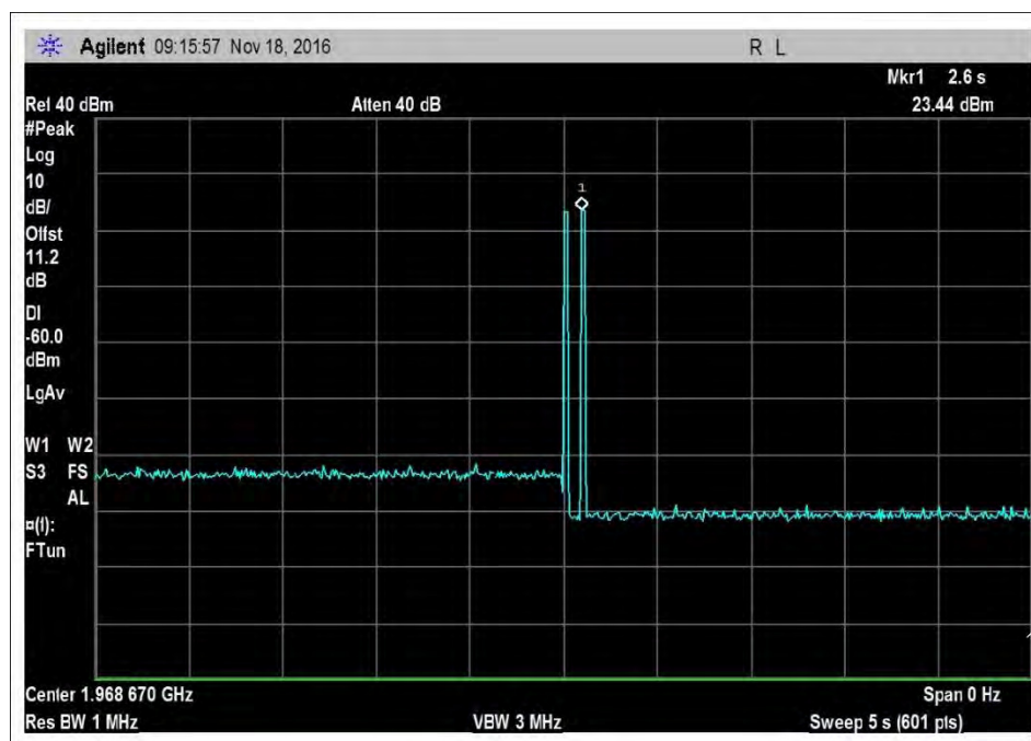
7.11_osc_DL-1930-1995MHz-Pk
