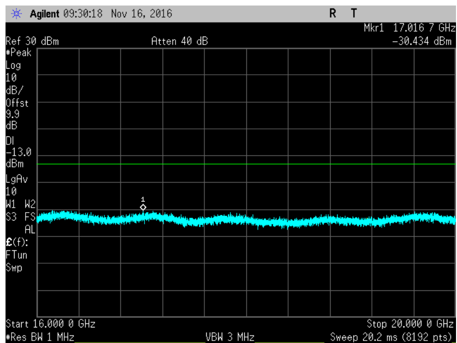
7.6_CSE_UL_1710-1755MHz_R5
