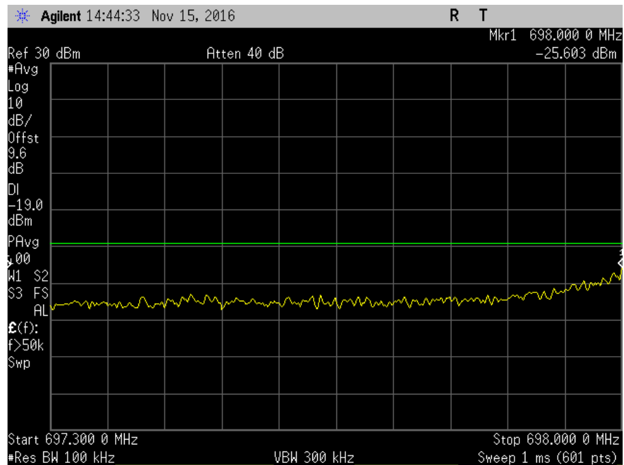
7.5_OBE_UL_698-716MHz_L_PreAGC_LTE
