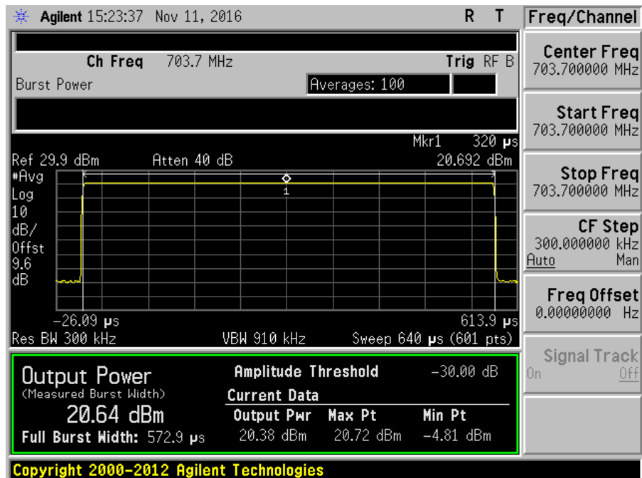
7.2_Power_UL_698-716MHz_GSM_Max
