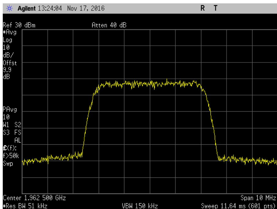
7.10_OBW_DL_1930-1995MHz_WCDMA_Out
