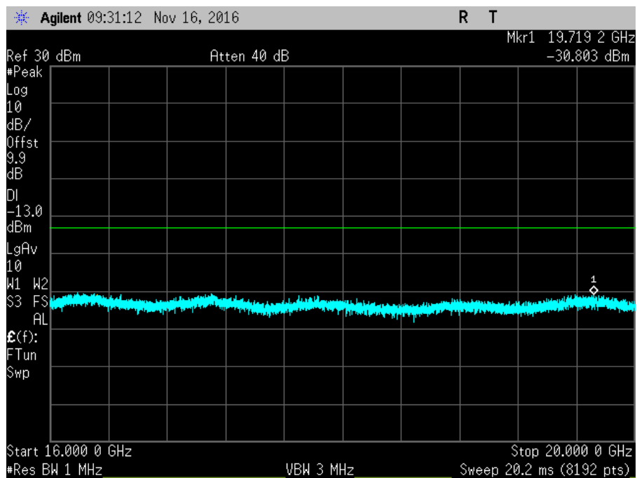
7.6_CSE_UL_1850-1915MHz_R5
