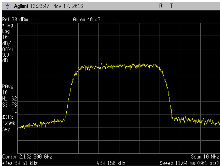
7.10_OBW_DL_2110-2155MHz_WCDMA_Out
