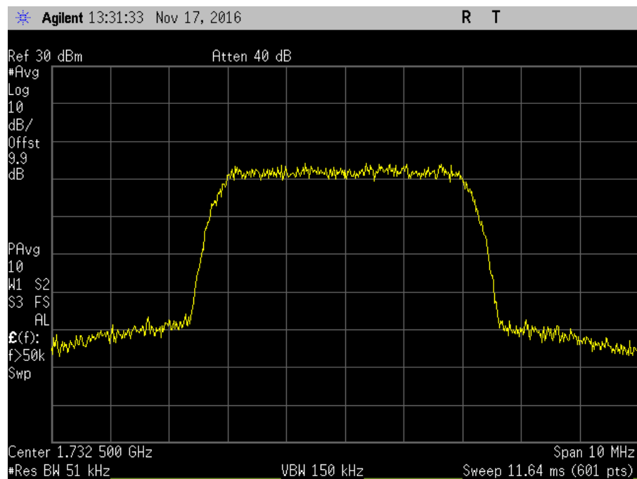
7.10_OBW_UL_1710-1755MHz_WCDMA_Out
