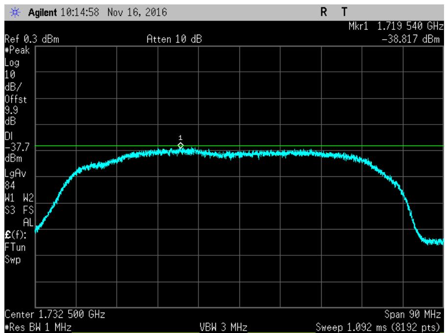
7.7.1_Noise_UL_1710-1755MHz
