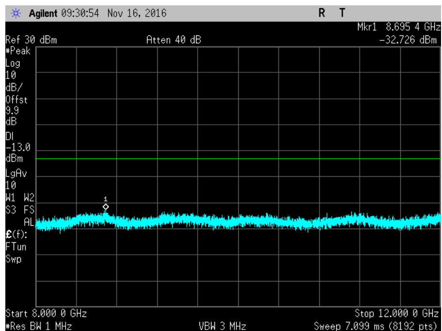
7.6_CSE_UL_1850-1915MHz_R3
