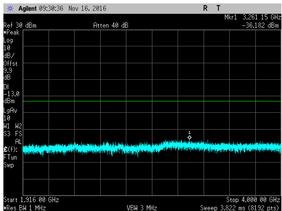
7.6_CSE_UL_1850-1915MHz_R1
