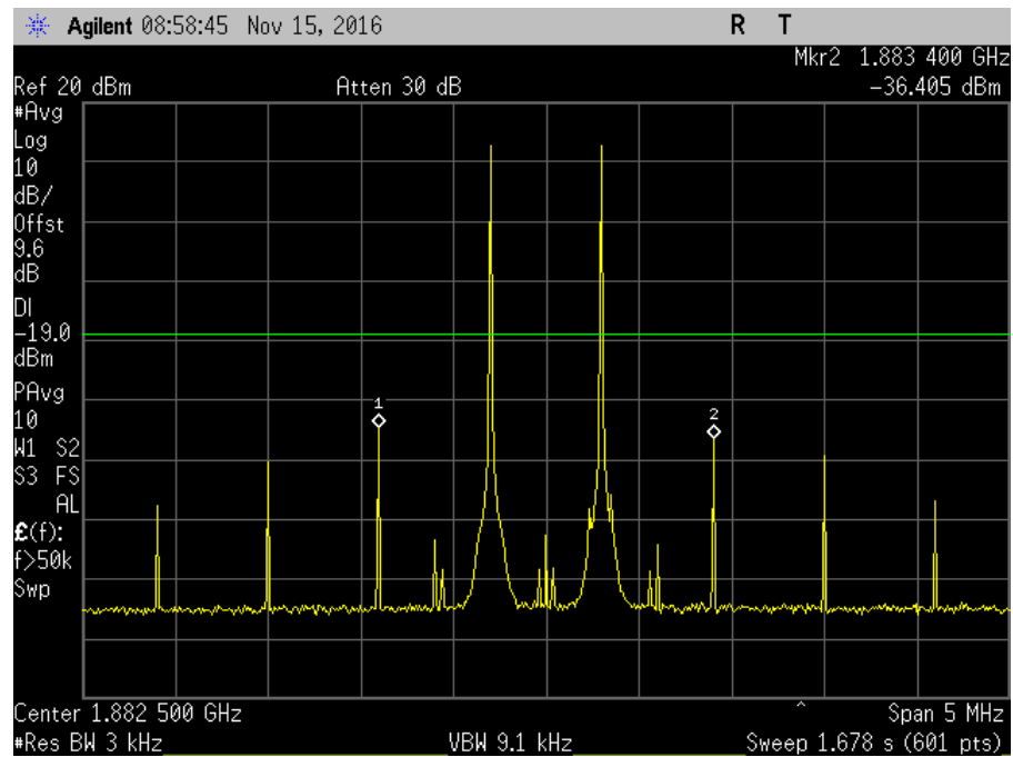
7.4_Intermod_UL_1850-1915MHz
