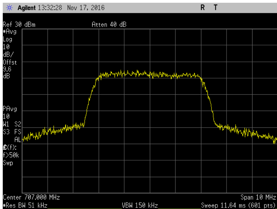
7.10_OBW_UL_698-716MHz_WCDMA_Out
