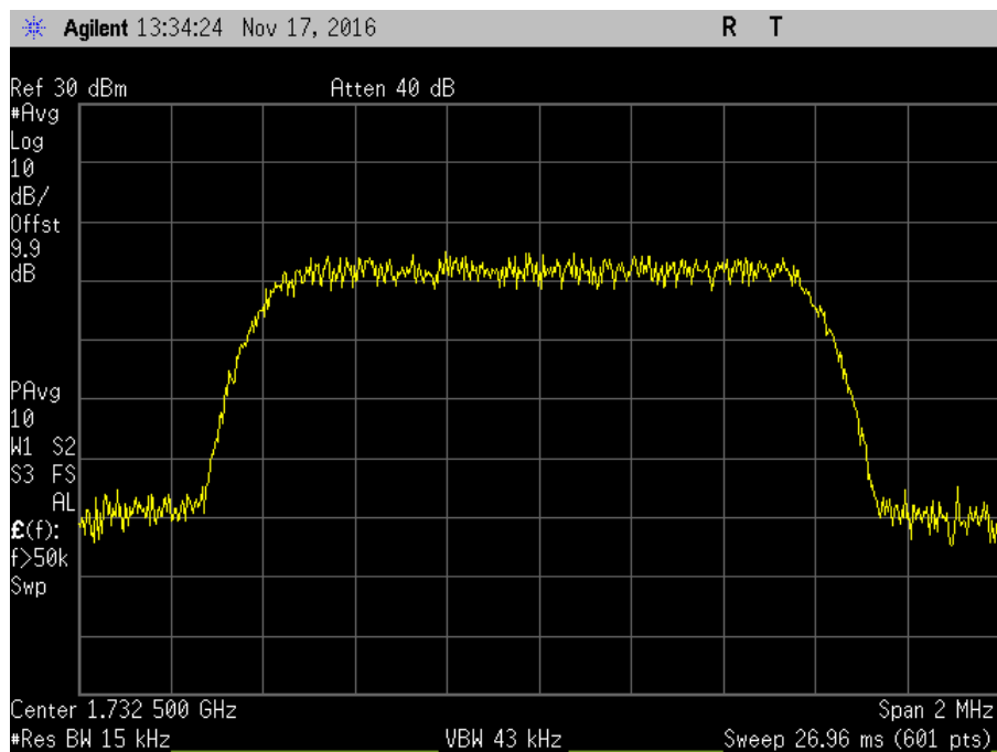
7.10_OBW_UL_1710-1755MHz_CDMA_Out
