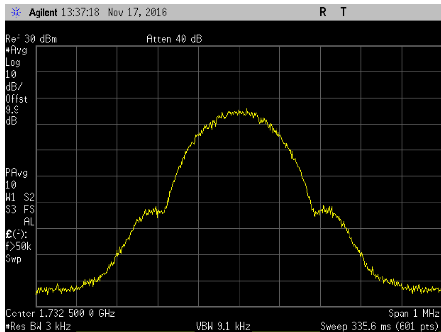
7.10_OBW_UL_1710-1755MHz_GSM_Out
