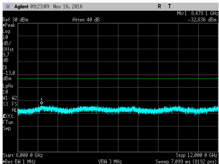
7.6_CSE_DL_869-894MHz_R3
