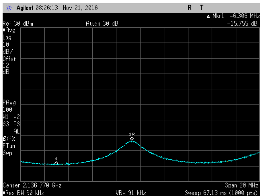
7.11.3_Osc_DL_2110-2155MHz+0_AWGNL
