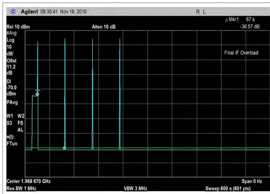
7.11_osc_DL-1930-1995MHz-600sec
