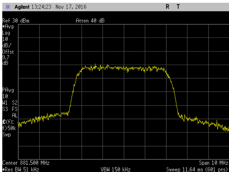
7.10_OBW_DL_869-894MHz_WCDMA_Out
