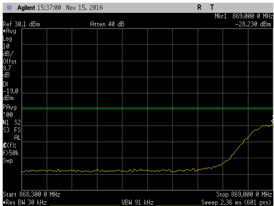
7.5_OBE_DL_869-894MHz_L_PreAGC_CDMA
