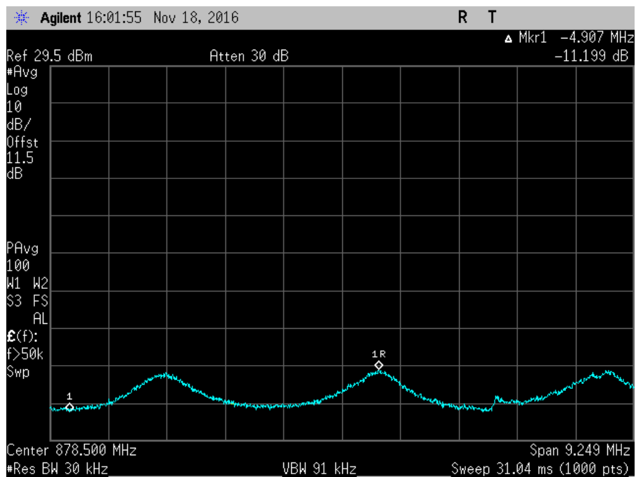
7.11.3_Osc_DL_869-894MHz+3_AWGNR
