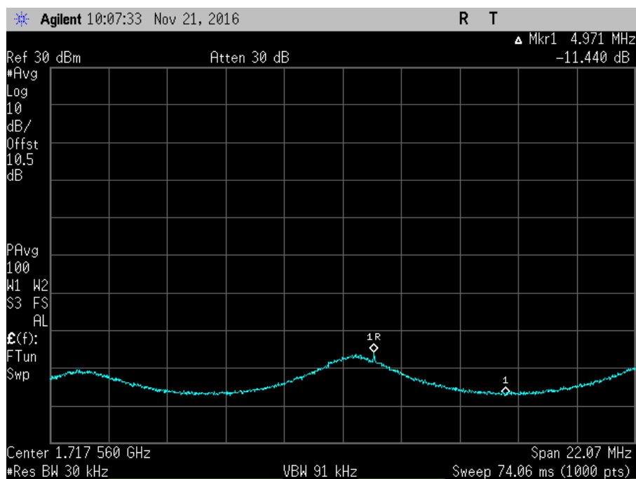
7.11.3_Osc_UL_1710-1755MHz+4_AWG NR
