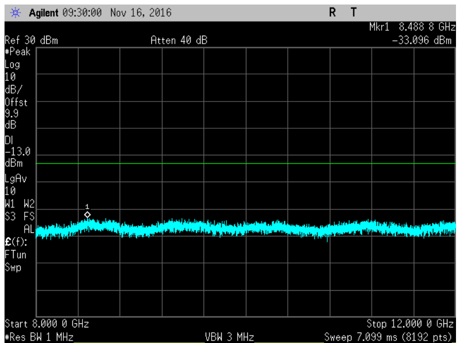
7.6_CSE_UL_1710-1755MHz_R3
