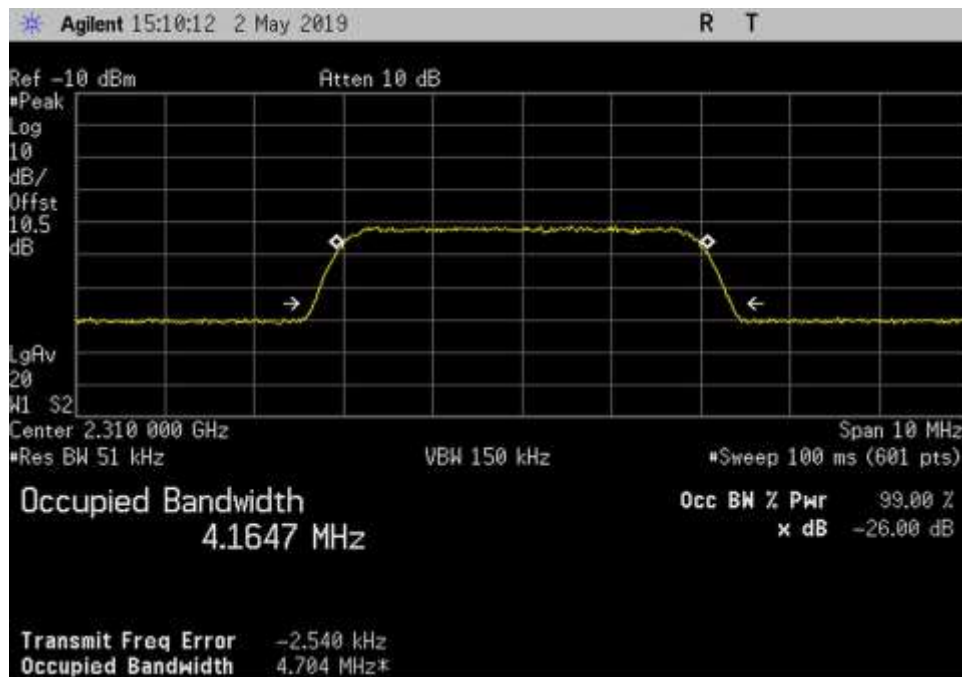
In_UL_2305-2315_AWGN_ 2310MHz
