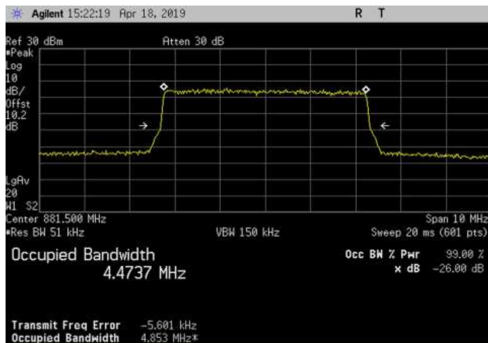
Out_DL_869-894_LTE_ 881.5MHz_3dB
