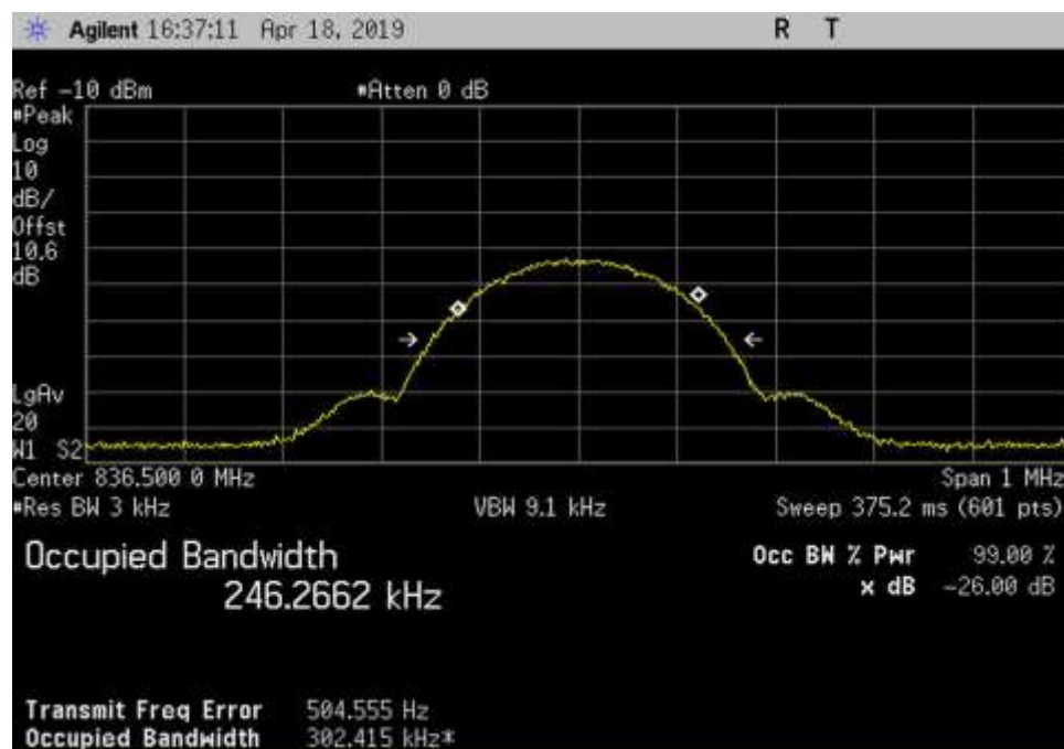
In_UL_824-849_GSM_ 836.5MHz
