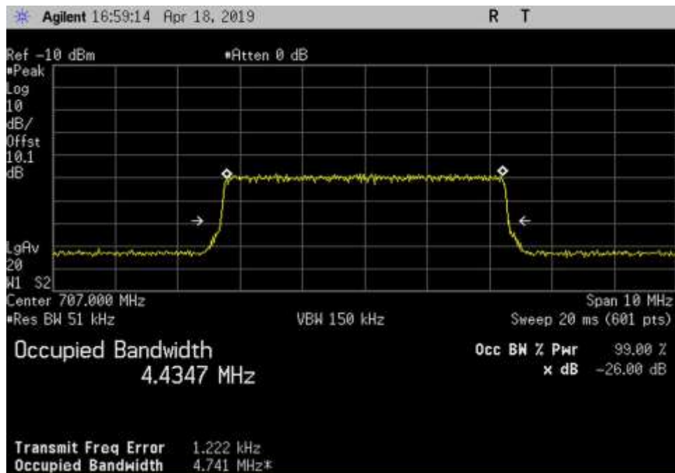
In_UL_698-716_LTE_707MHz
