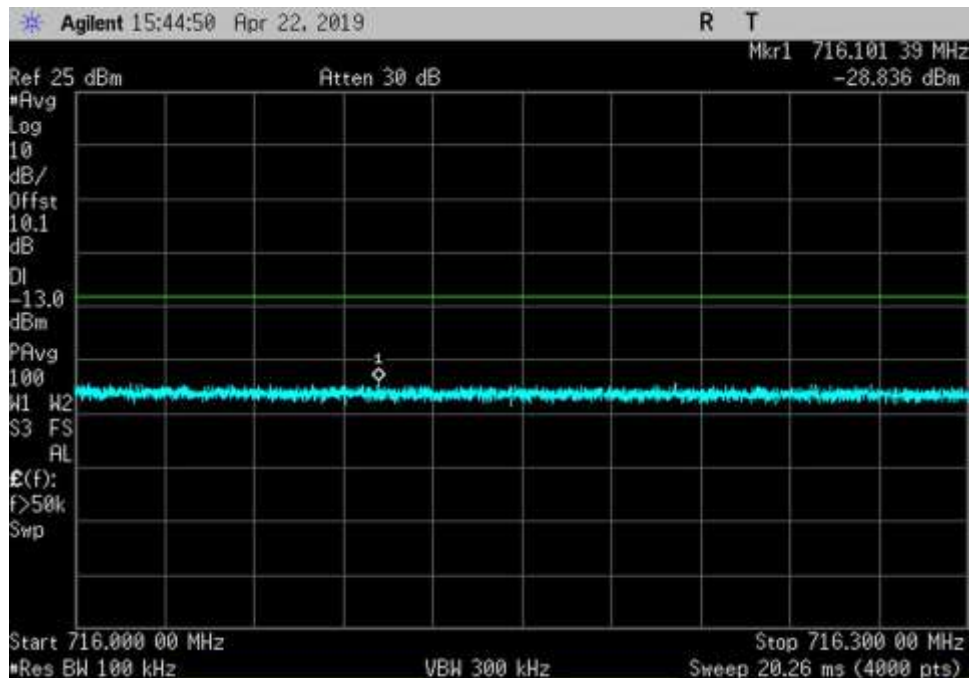
UL_698-716_AWGN_ 716- 716.3MHz_Cm-H+3dB
