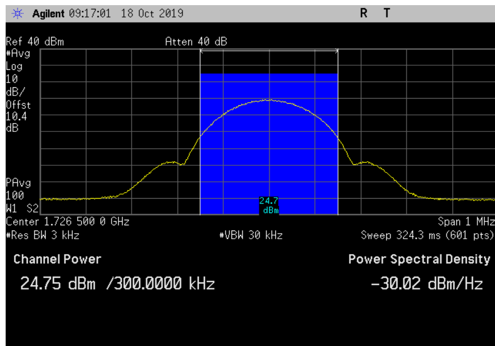
UL_1710-1755_GSM_ 1726.5MHz_3dB
