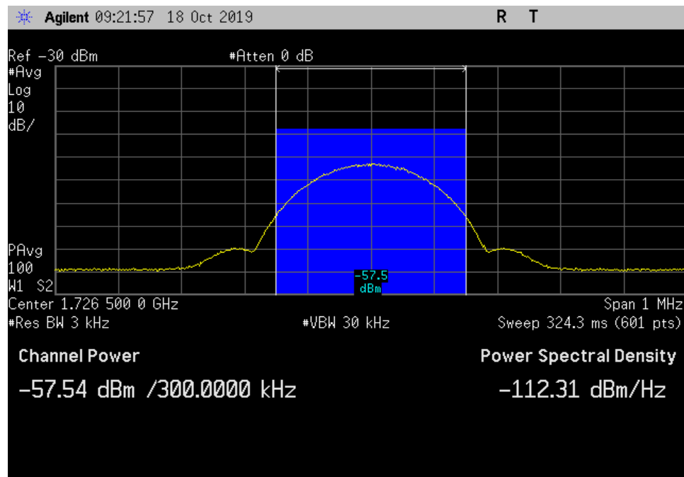
UL_1710-1755_GSM_ 1726.5MHz_Input
