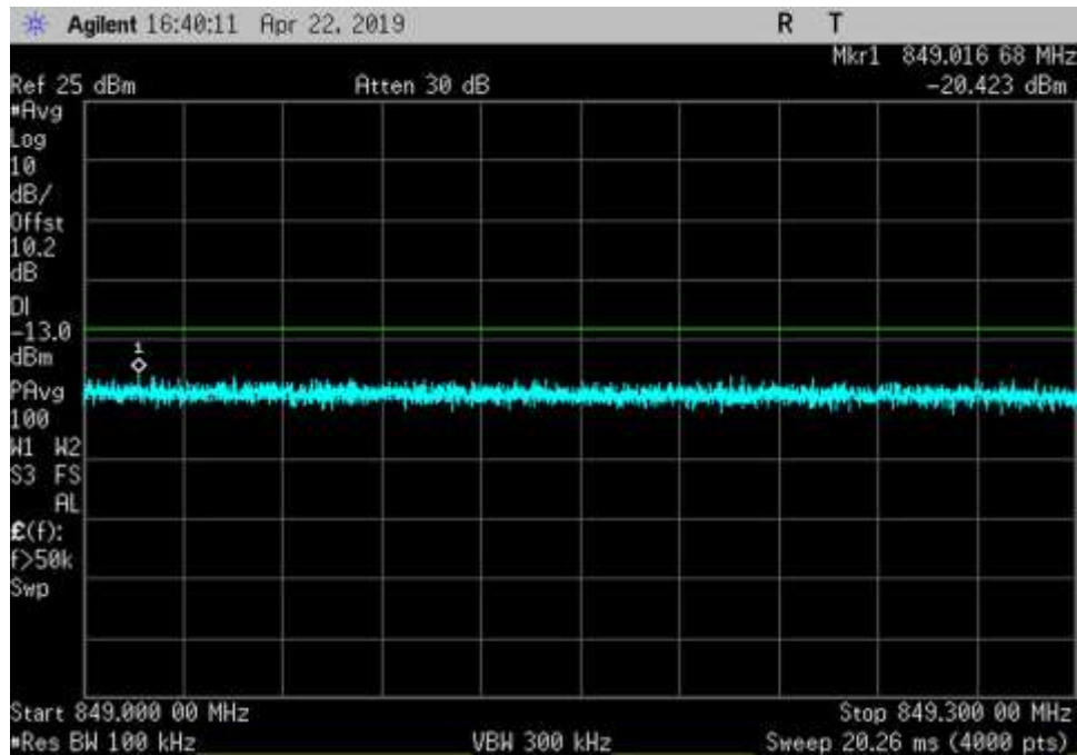
UL_824-849_AWGN_ 849- 849.3MHz_Sn-H
