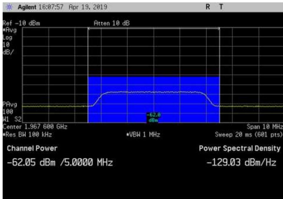
DL_1930-1995_AWGN_ 1967.6MHz_Input
