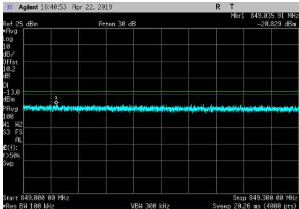
UL_824-849_AWGN_ 849- 849.3MHz_Sn-H+3dB
