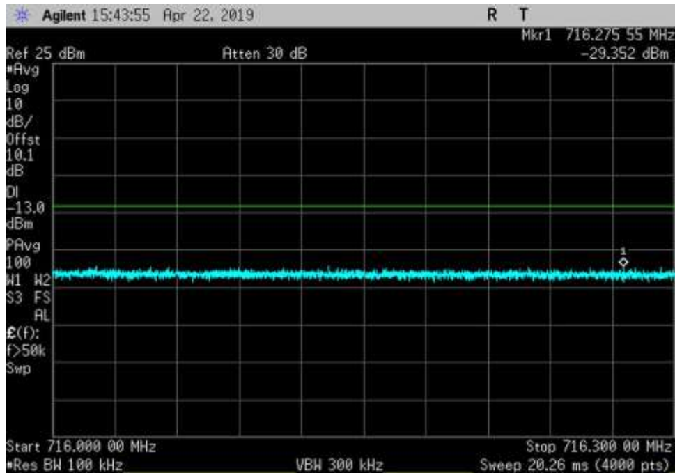
UL_698-716_AWGN_ 716- 716.3MHz_Cm-H
