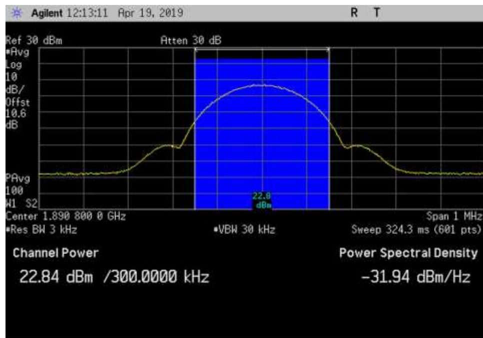
UL_1850-1915_GSM_ 1890.8MHz
