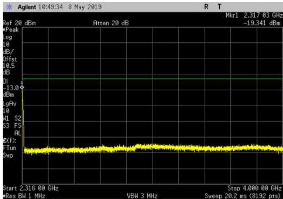
UL_2305-2315_GSM_2316- 4000MHz_LC
