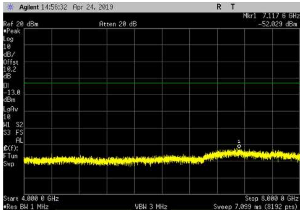
DL_746-757_GSM_4000- 8000MHz_HC
