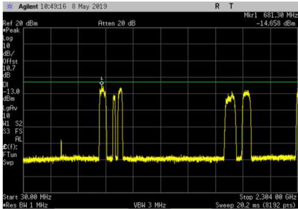
UL_2305-2315_GSM_30- 2304MHz_LC
