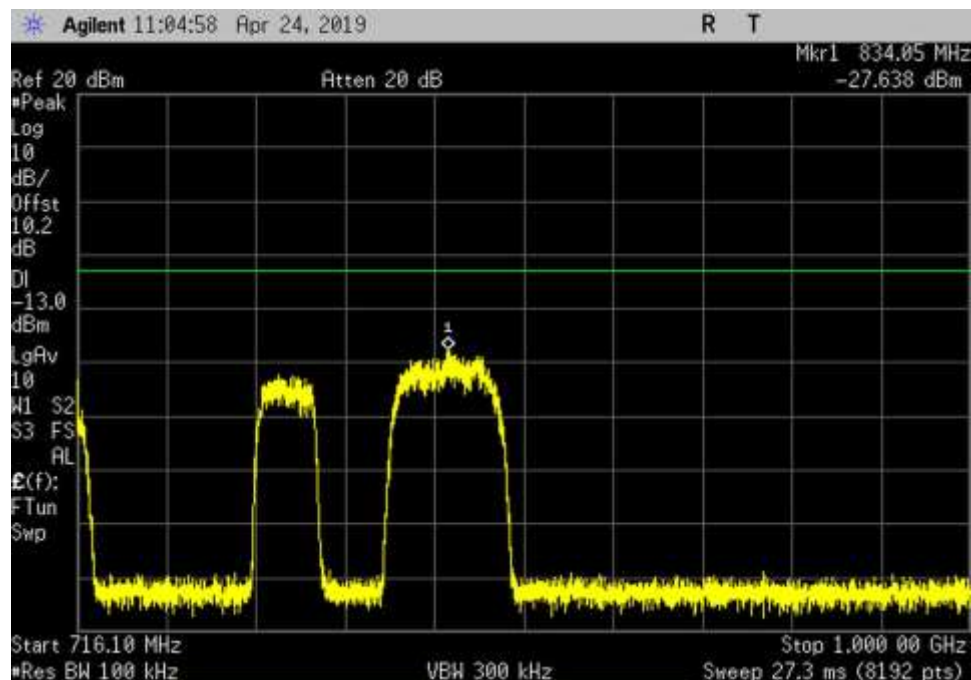
UL_698-716_GSM_716.1- 1000MHz_HC
