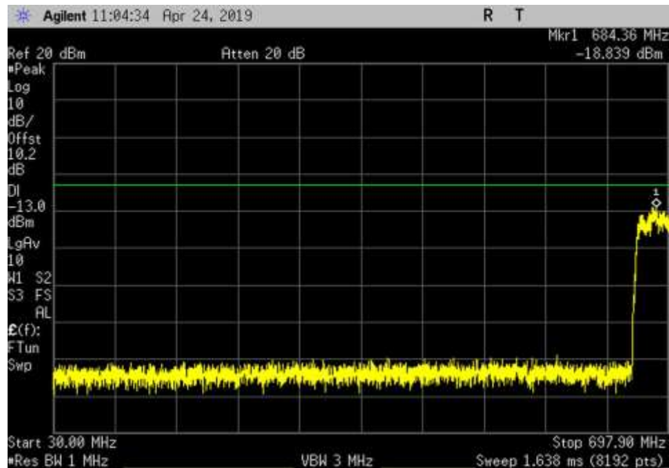
UL_698-716_GSM_30- 697.9MHz_HC
