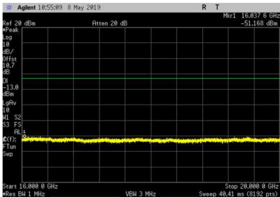
UL_2305-2315_GSM_16000-20000MHz_HC
