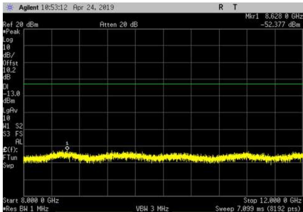
UL_824-849_GSM_8000- 12000MHz_LC
