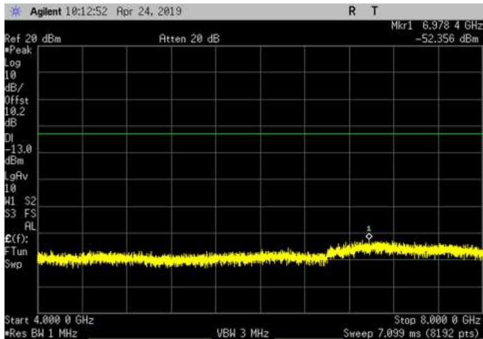
UL_663-698_GSM_4000-8000MHz_MC
