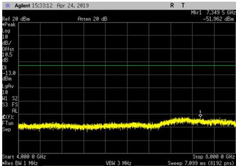
DL_1930-1995_AWGN_4000- 8000MHz_MC
