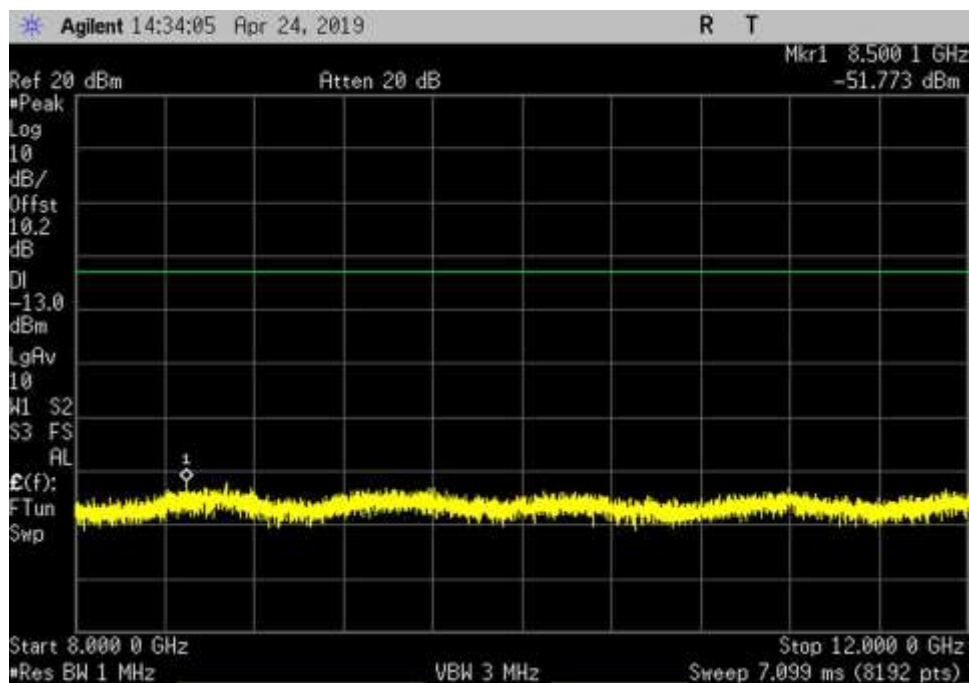
DL_869-894_GSM_8000-12000MHz_HC
