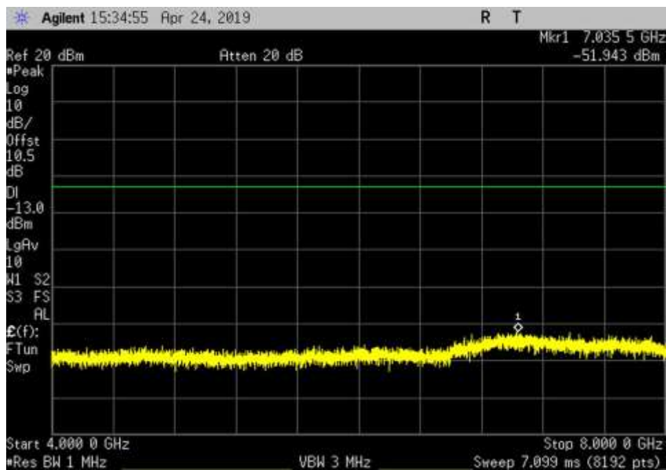
DL_1930-1995_AWGN_4000- 8000MHz_HC
