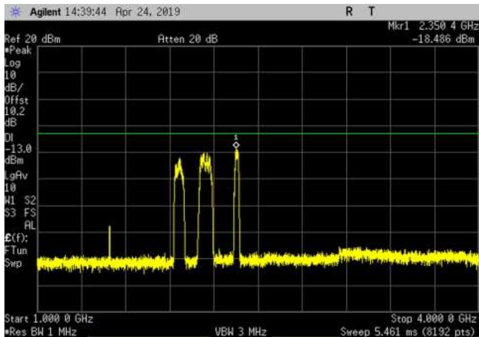
DL_728-746_GSM_1000- 4000MHz_HC
