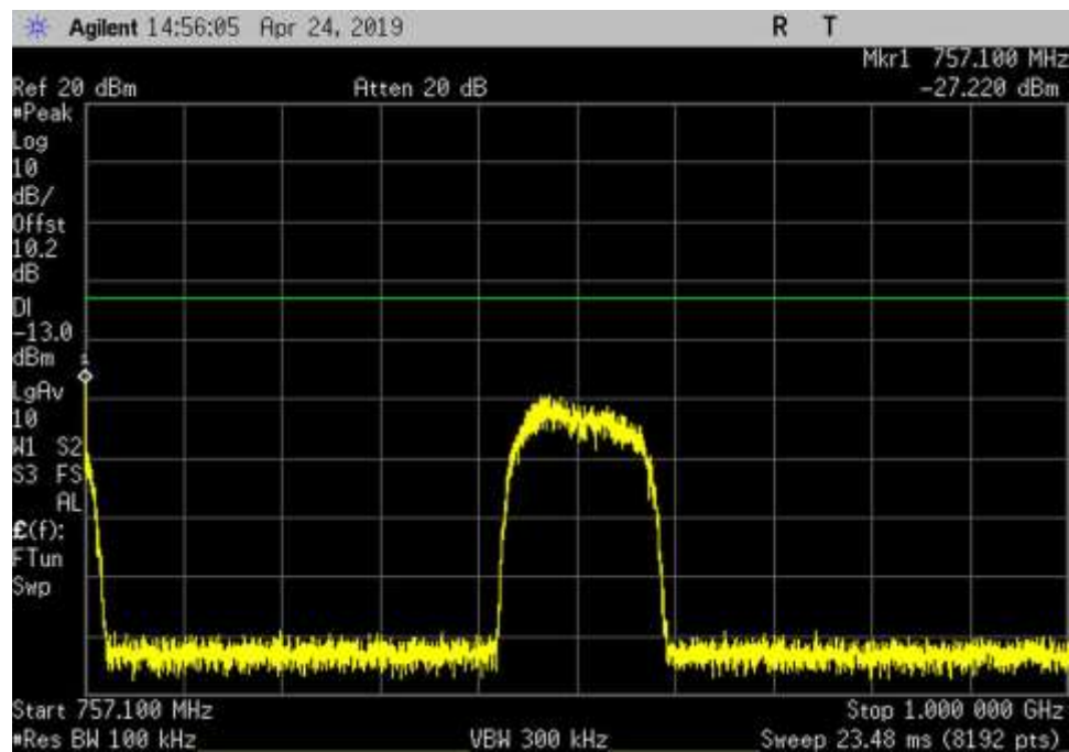
DL_746-757_GSM_757.1- 1000MHz_HC
