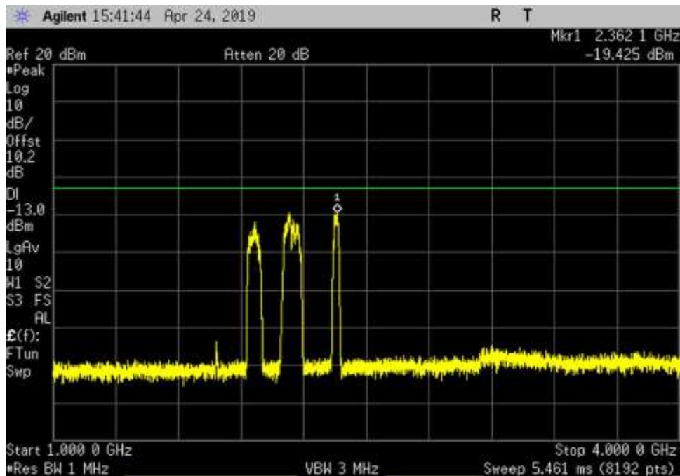
DL_869-894_AWGN_1000- 4000MHz_HC
