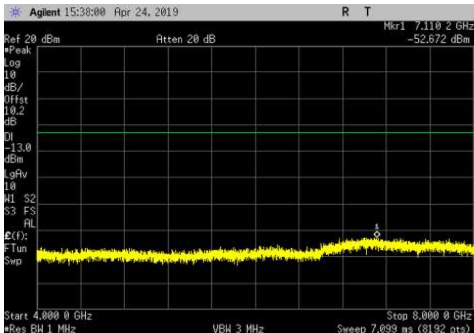
DL_869-894_AWGN_4000- 8000MHz_LC
