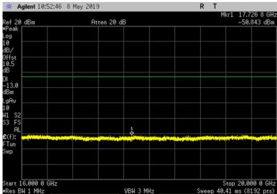
UL_2305-2315_GSM_16000-20000MHz_MC
