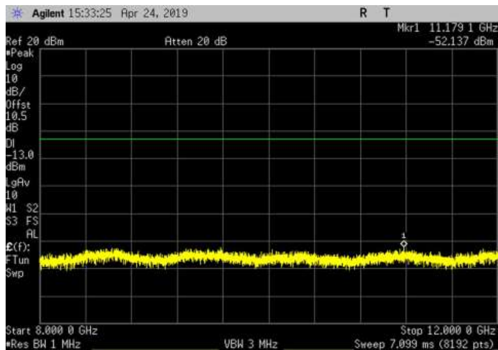
DL_1930-1995_AWGN_ 8000- 12000MHz_MC
