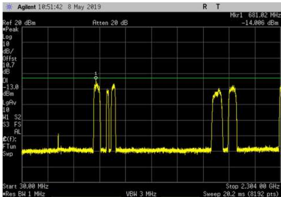
UL_2305-2315_GSM_30- 2304MHz_MC
