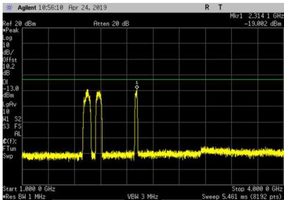
UL_824-849_GSM_1000- 4000MHz_HC
