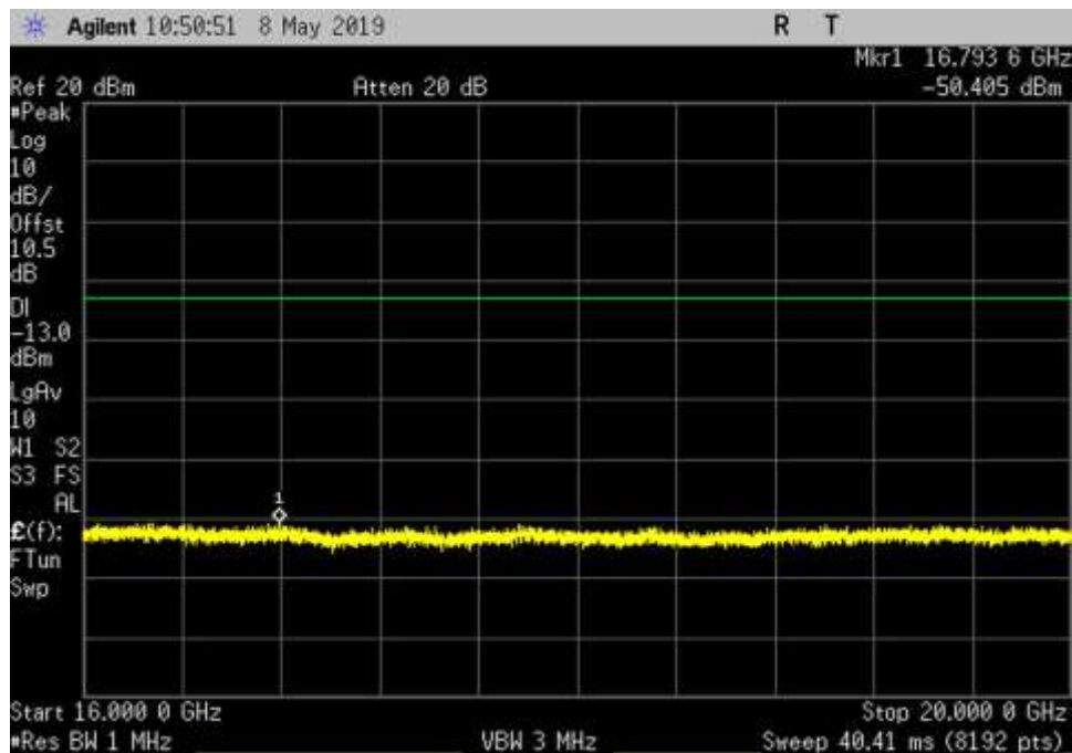
UL_2305-2315_GSM_16000- 20000MHz_LC
