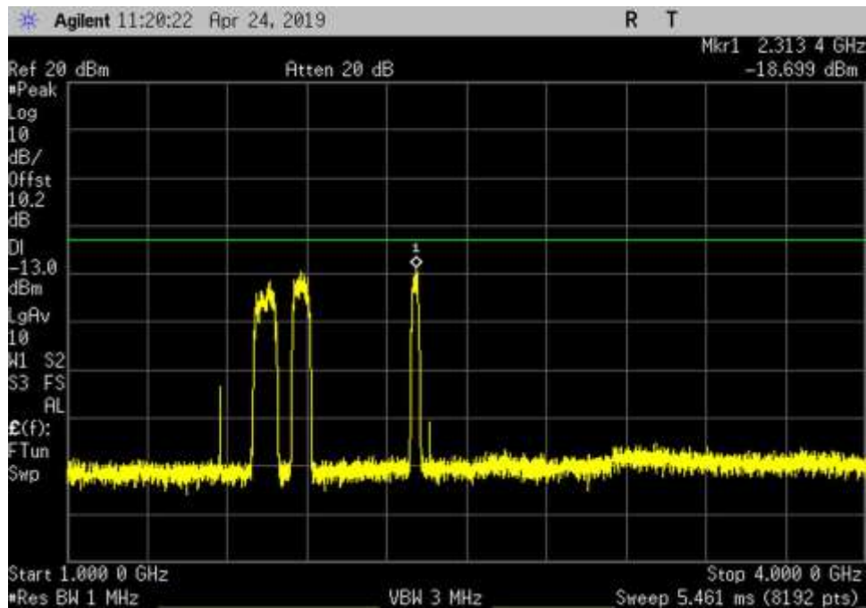
UL_776-787_GSM_1000- 4000MHz_HC
