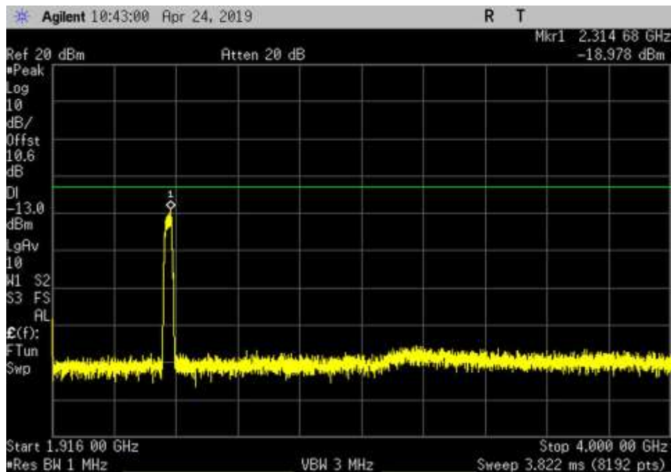
UL_1850-1915_GSM_1916-4000MHz_LC
