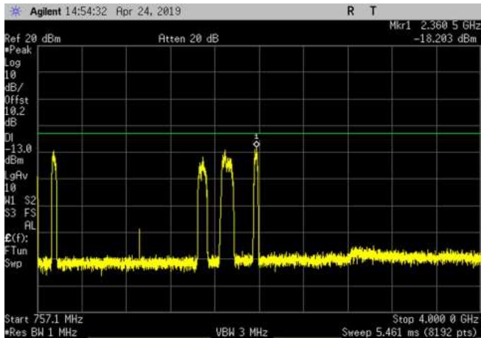
DL_746-757_GSM_757.1-4000MHz_MC
