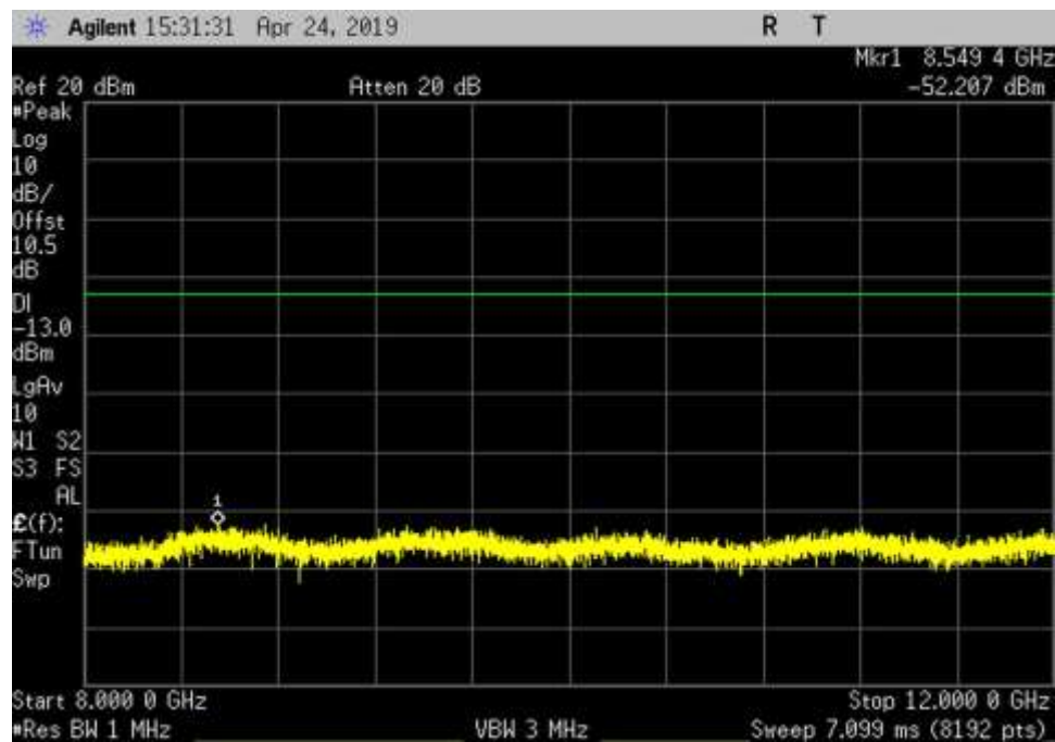
DL_1930-1995_AWGN_ 8000- 12000MHz_LC
