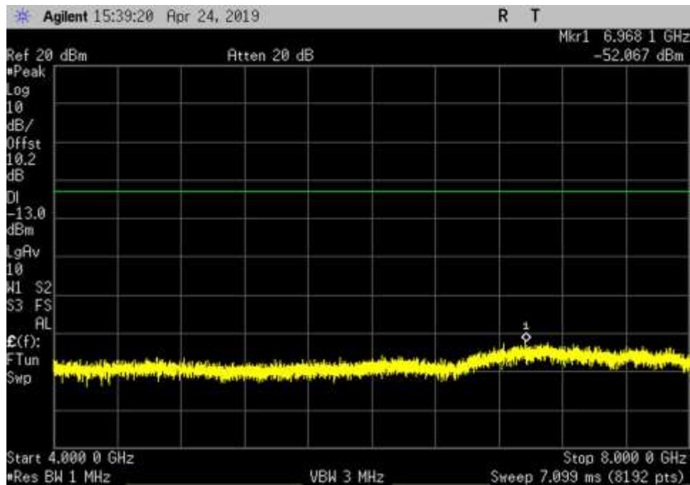
DL_869-894_AWGN_4000- 8000MHz_MC
