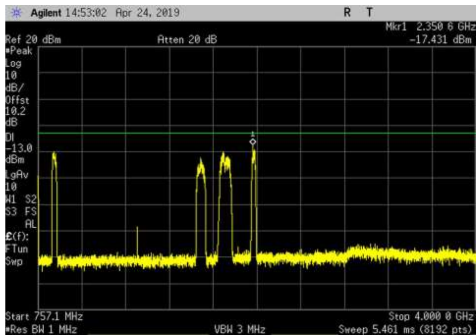
DL_746-757_GSM_757.1- 4000MHz_LC
