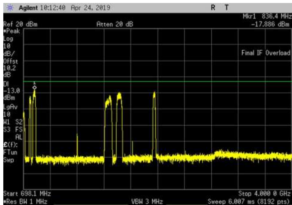
UL_663-698_GSM_698.1- 4000MHz_MC
