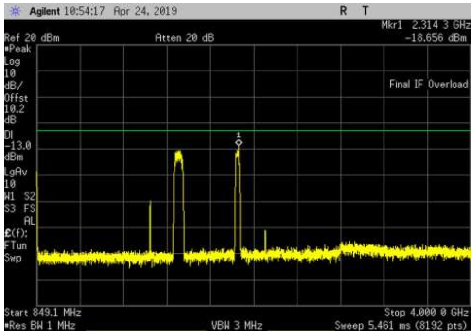
UL_824-849_GSM_849.1- 4000MHz_MC
