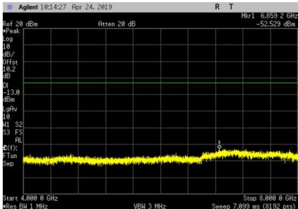
UL_663-698_GSM_4000-8000MHz_HC
