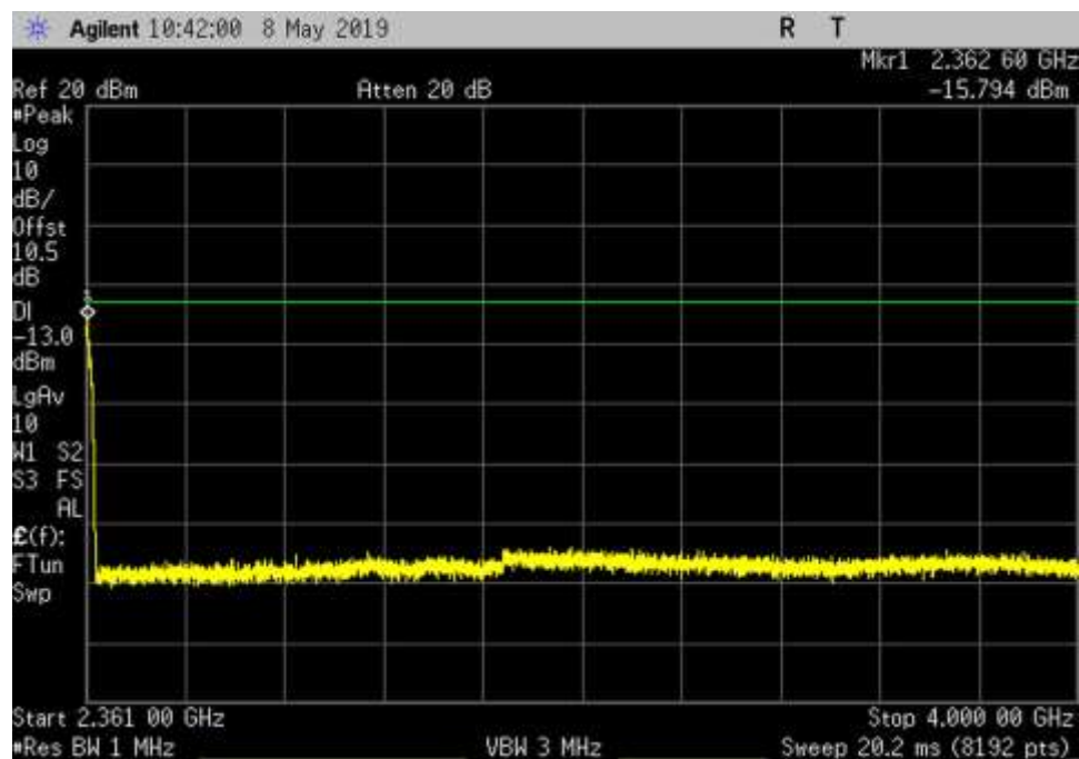
DL_2350-2360_GSM_2361- 4000MHz_MC
