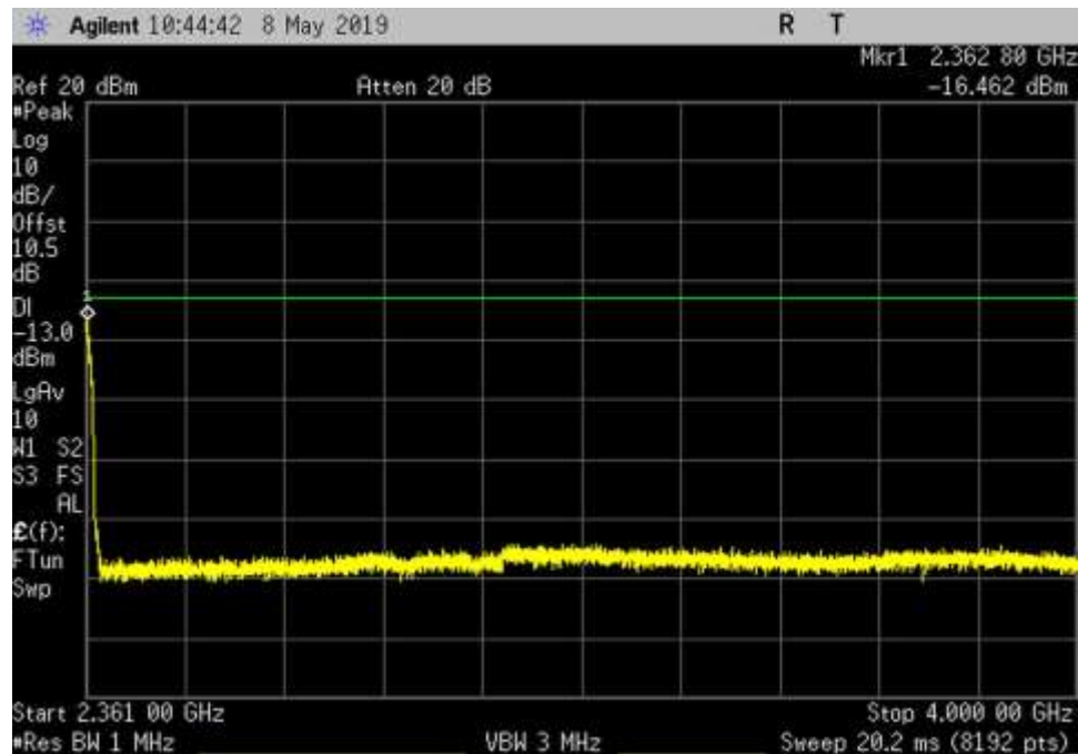
DL_2350-2360_GSM_2361- 4000MHz_HC
