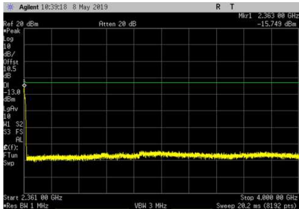
DL_2350-2360_GSM_2361- 4000MHz_LC
