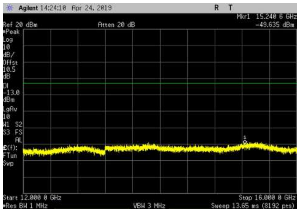
DL_1930-1995_GSM_12000- 16000MHz_MC
