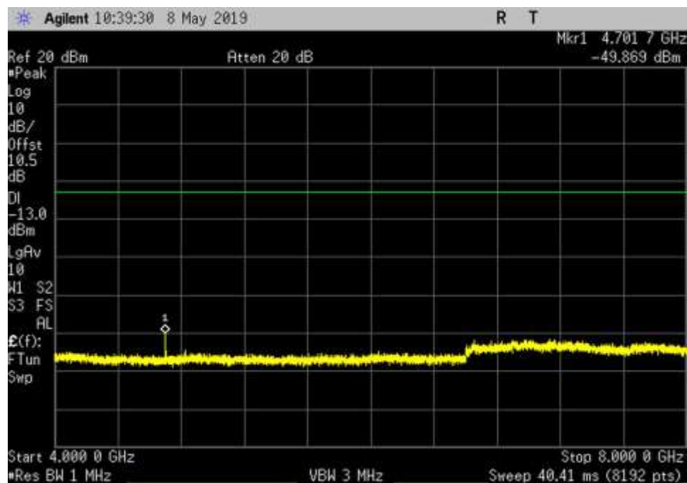
DL_2350-2360_GSM_4000- 8000MHz_LC
