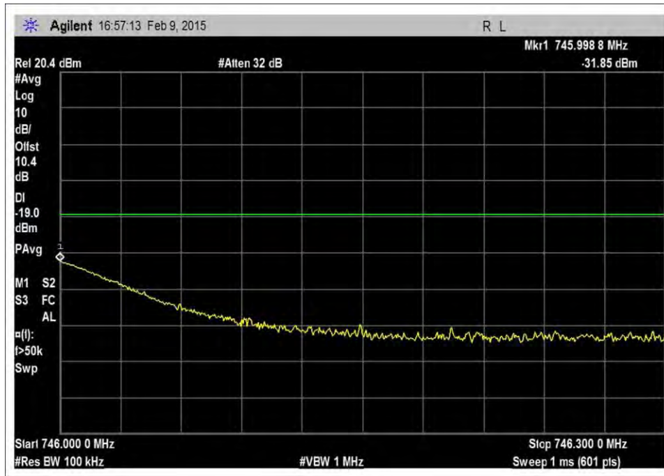
7.5_OBE_DL_728-746MHz_GSM_H_-54dBm
