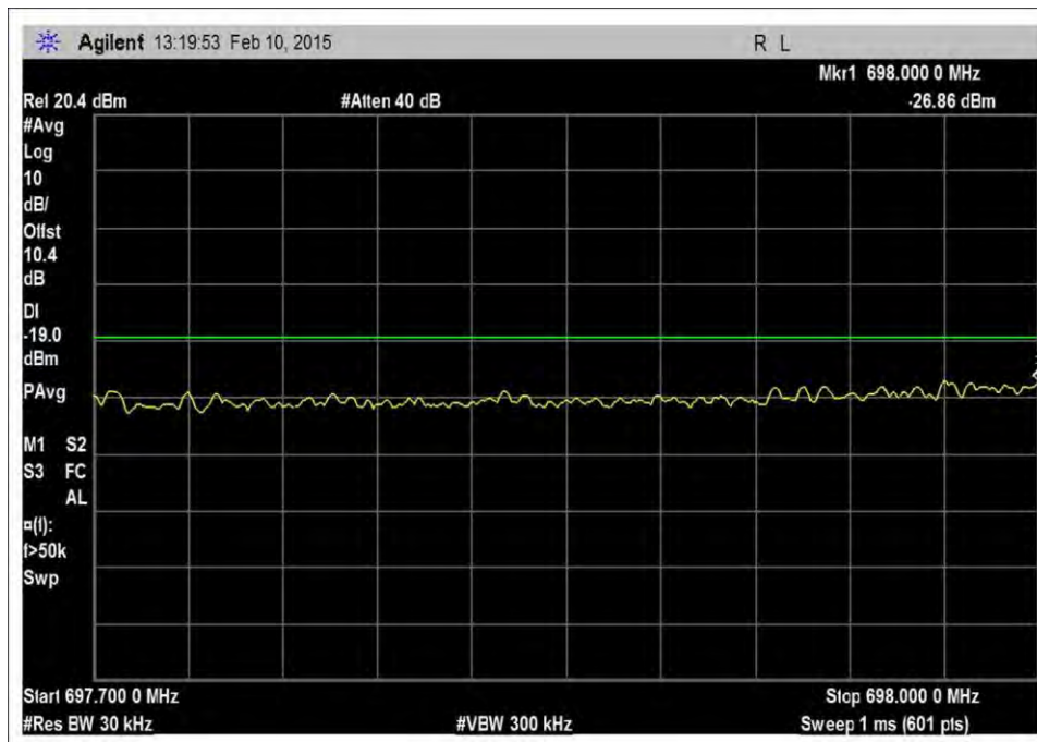
7.5_OBE_UL_698-716MHz_LTE_L_-22dBm
