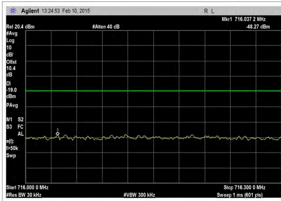
7.5_OBE_UL_698-716MHz_LTE_H_+10dBm
