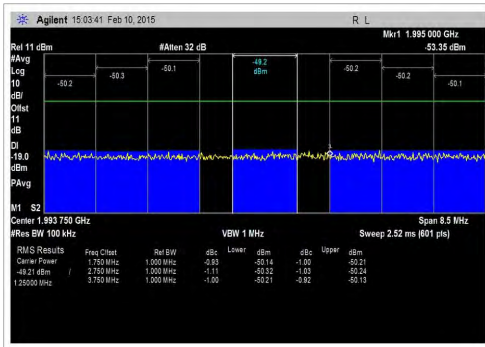
7.5_OBE_DL_1930-1995MHz_CDMA_H_-20dBm
