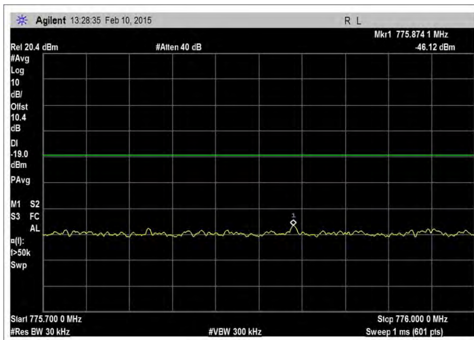
7.5_OBE_UL_776-787MHz_LTE_L_+10dBm
