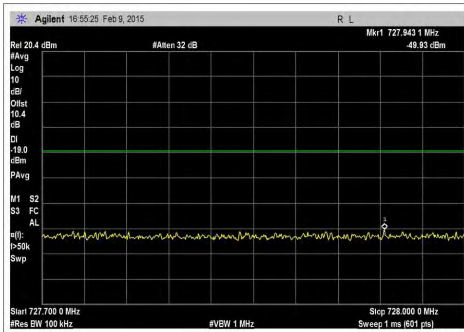
7.5_OBE_DL_728-746MHz_GSM_L_-20dBm
