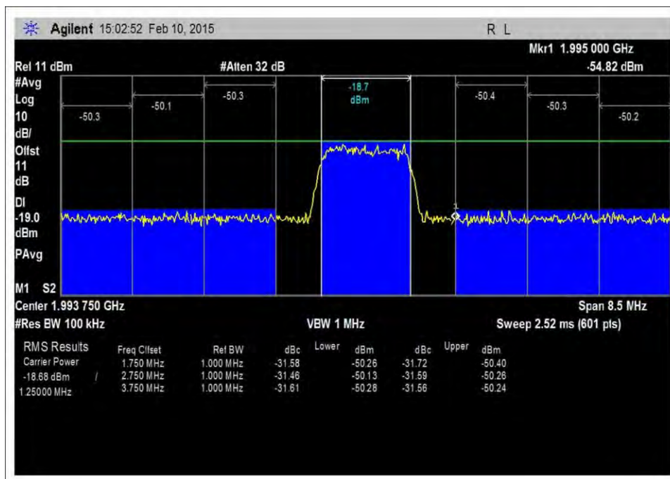
7.5_OBE_DL_1930-1995MHz_CDMA_H_-46dBm
