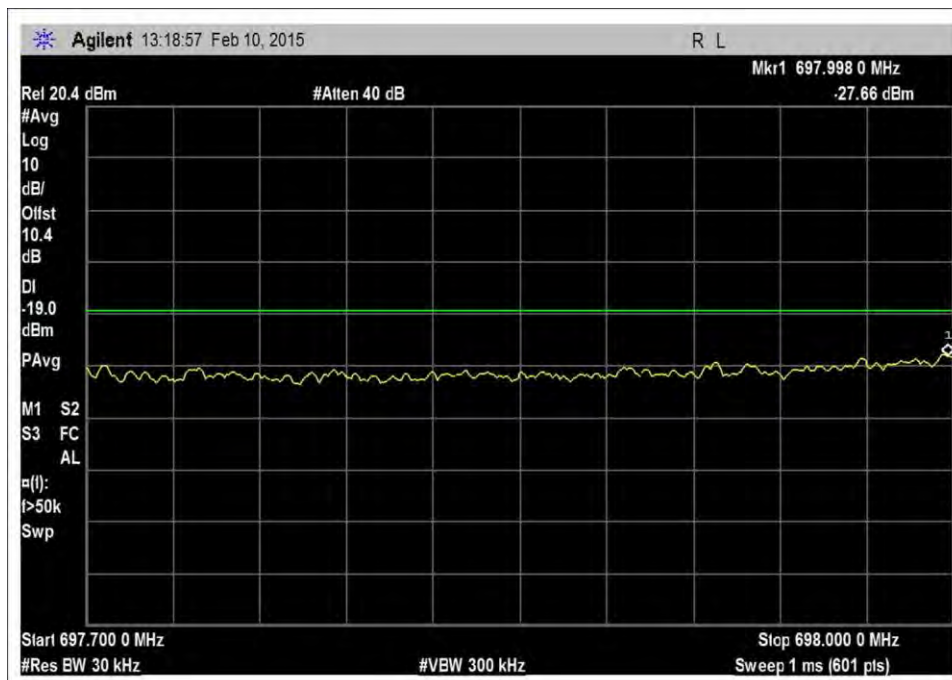
7.5_OBE_UL_698-716MHz_LTE_L_-27dBm
