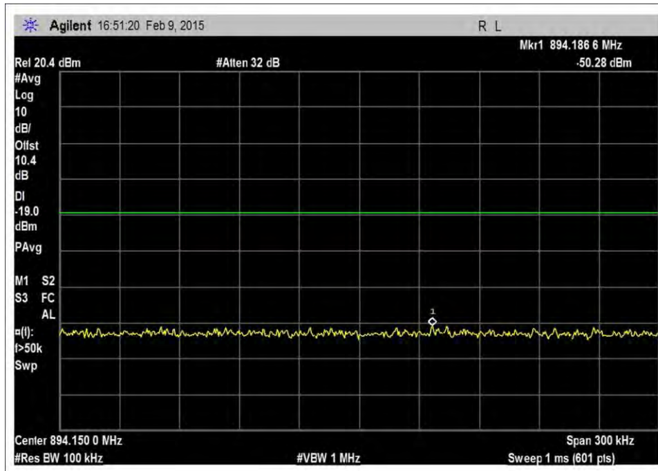
7.5_OBE_DL_869-894MHz_GSM_H_-20dBm
