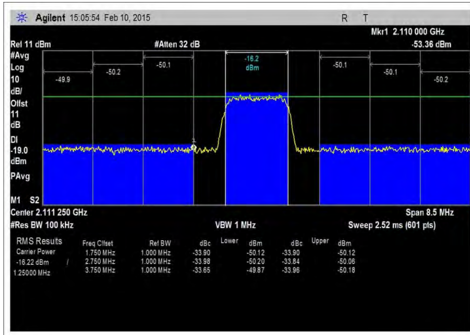
7.5_OBE_DL_2110-2155MHz_CDMA_L_-54dBm
