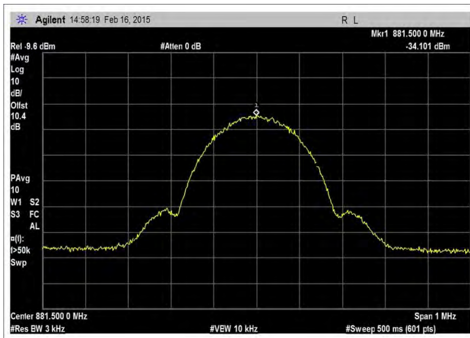
7.10_OBW_DL_869-894MHz_GSM_Output
