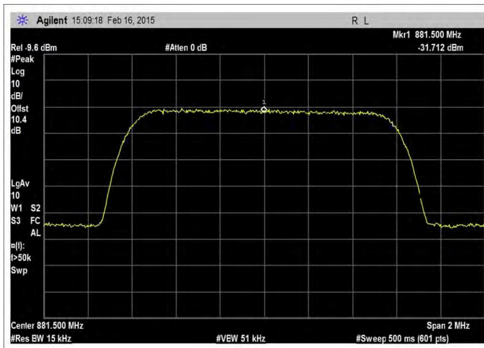
7.10_OBW_DL_869-894MHz_CDMA_Output
