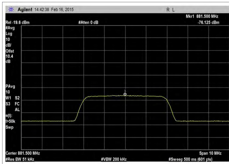
7.10_OBW_DL_869-894MHz_WCDMA_Input
