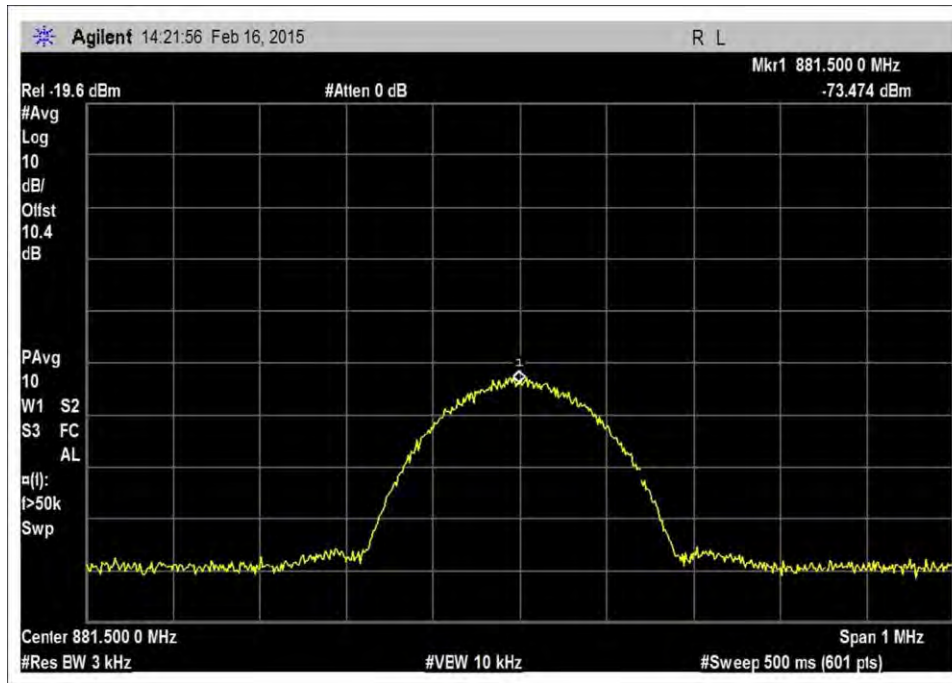
7.10_OBW_DL_869-894MHz_GSM__Input
