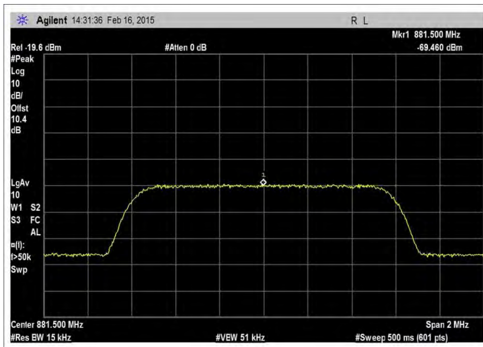
7.10_OBW_DL_869-894MHz_CDMA_Input
