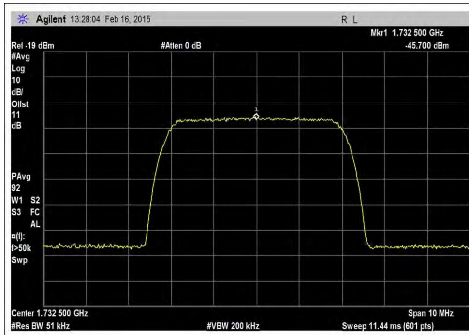
7.10_OBW_UL_1710-1755MHz_WCDMA_Input
