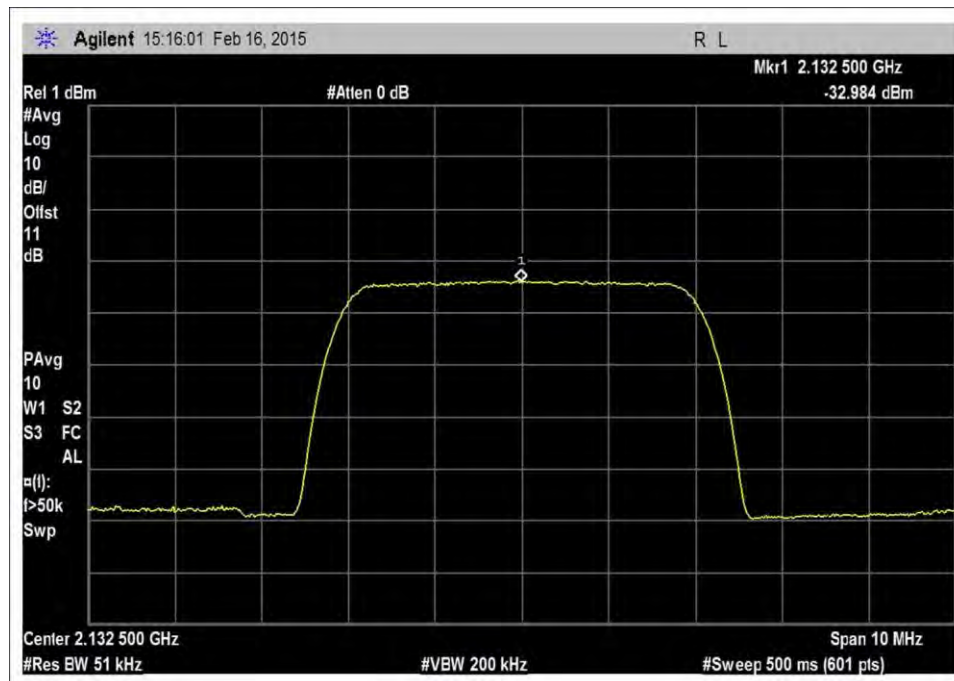
7.10_OBW_DL_2110-2155MHz_WCDMA_Output
