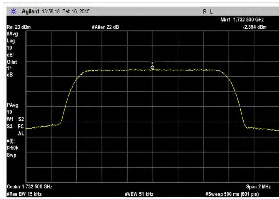
7.10_OBW_UL_1710-1755MHz_CDMA_Output
