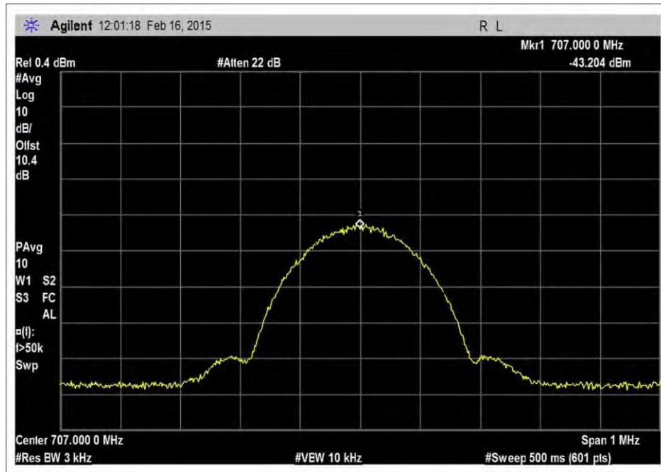
7.10_OBW_UL_698-716MHz_GSM__Input
