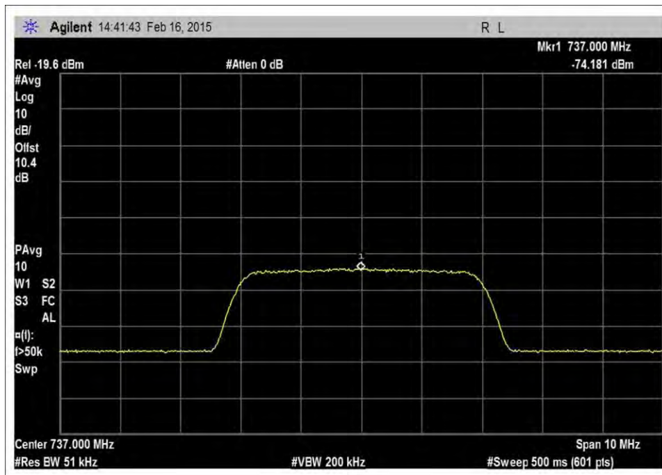
7.10_OBW_DL_728-746MHz_WCDMA_Input
