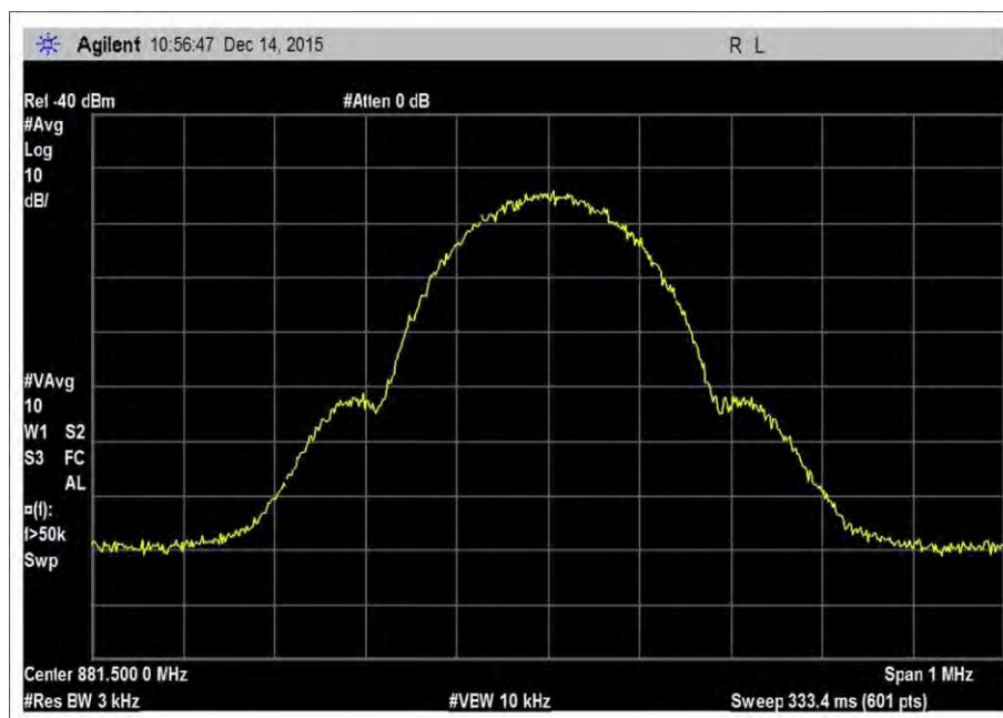
7.10_OBW_DL_869-894MHz_GSM
