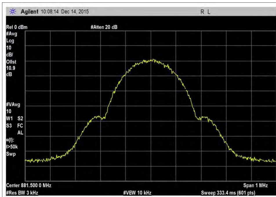
7.10_OBW_DL_869-894MHz_GSM
