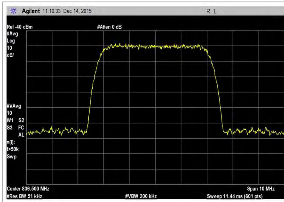
7.10_OBW_UL_824-849MHz_WCDMA
