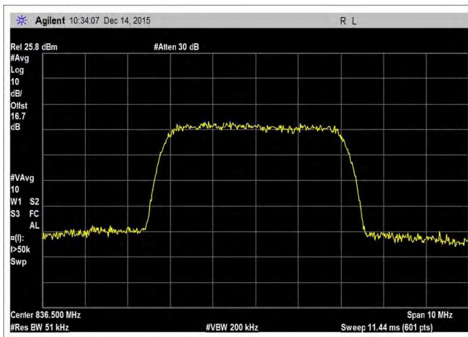
7.10_OBW_UL_824-849MHz_WCDMA
