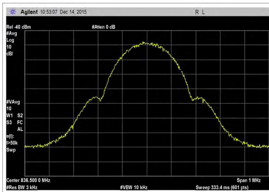
7.10_OBW_UL_824-849MHz_GSM
