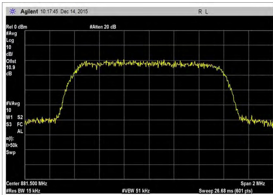
7.10_OBW_DL_869-894MHz_CDMA
