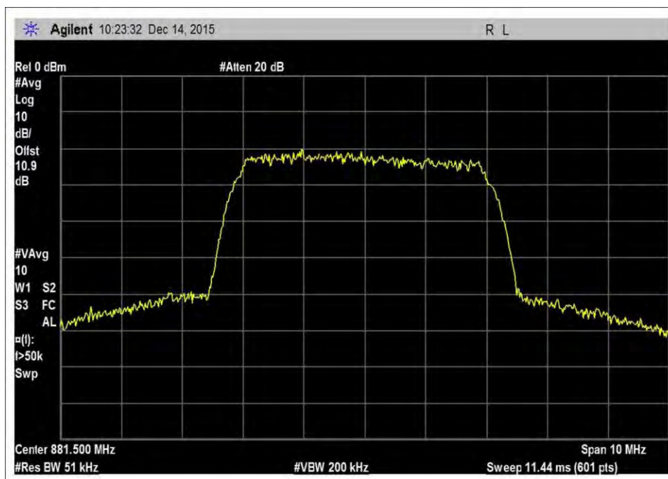
7.10_OBW_DL_869-894MHz_WCDMA
