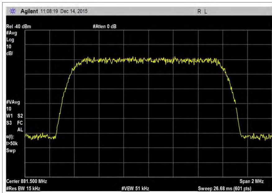
7.10_OBW_DL_869-894MHz_CDMA
