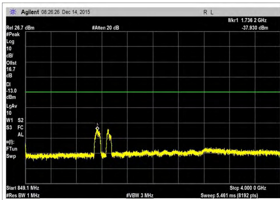
UL_824-849R1
