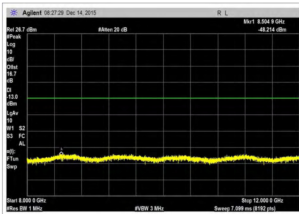
UL_824-849R3
