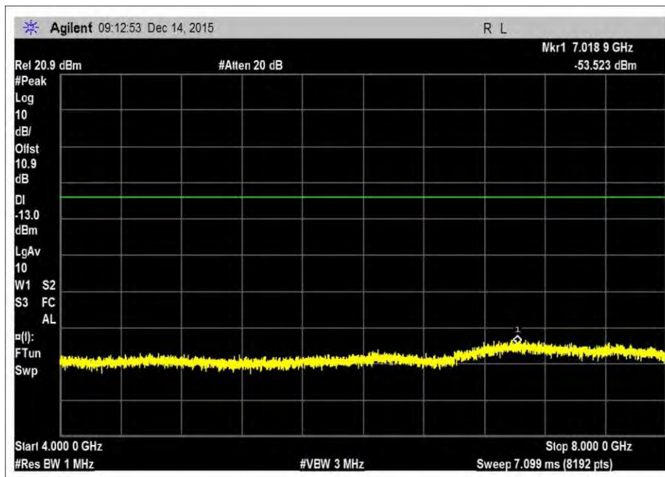
DL_869-894R2
