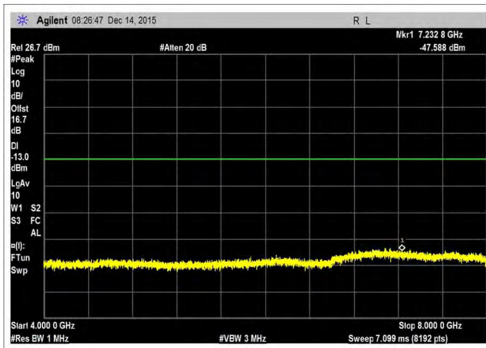
UL_824-849R2
