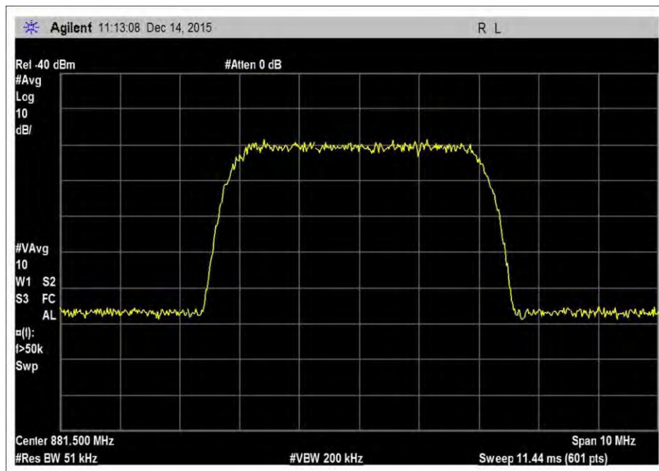
7.10_OBW_DL_869-894MHz_WCDMA
