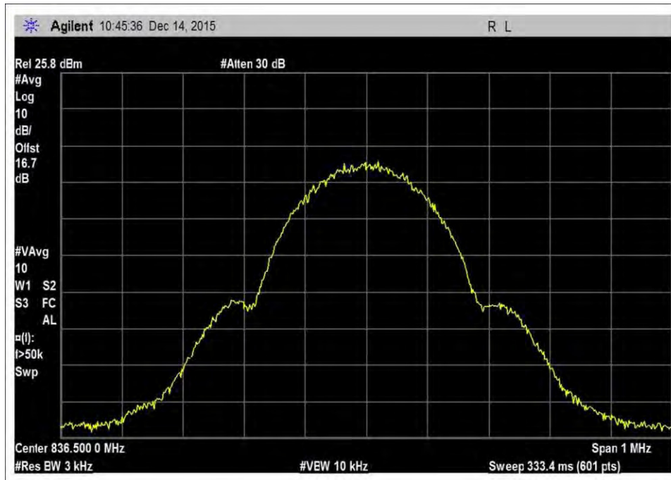
7.10_OBW_UL_824-849MHz_GSM
