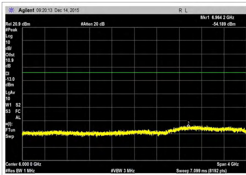
DL_746-757R2
