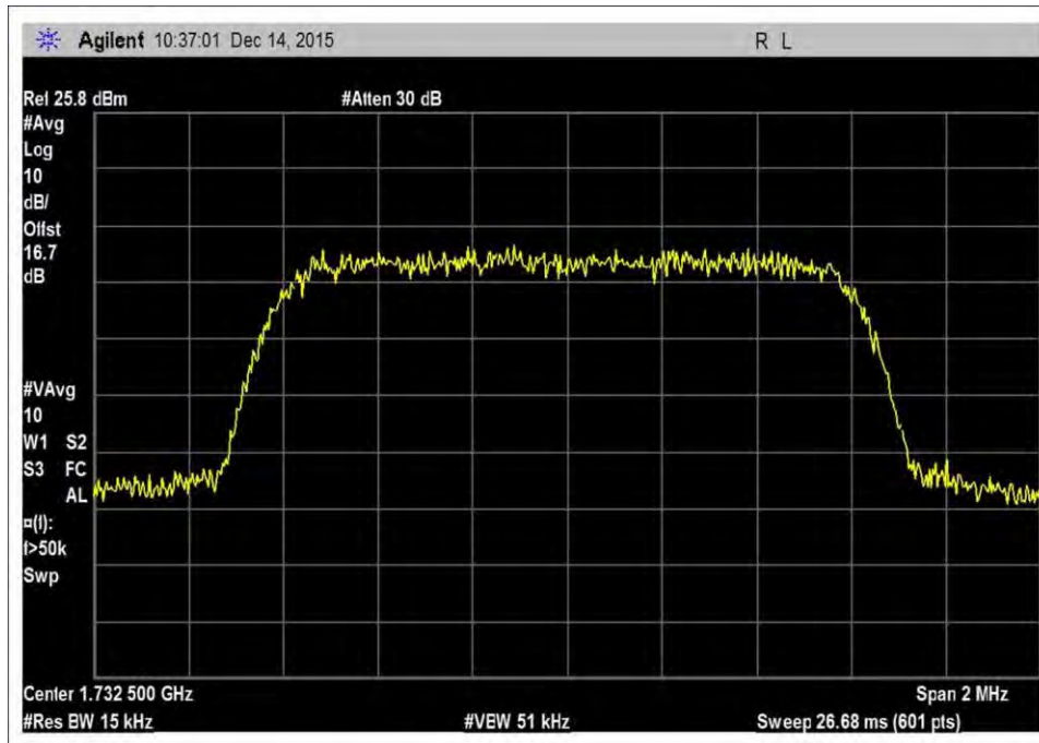
7.10_OBW_UL_1710-1755MHz_CDMA
