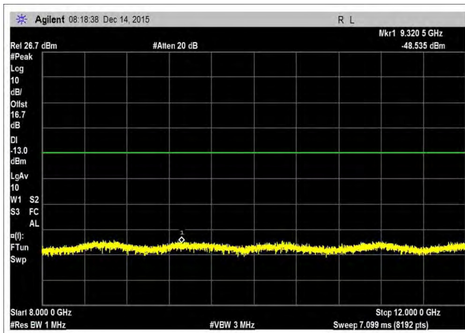
UL_1710-1755R3
