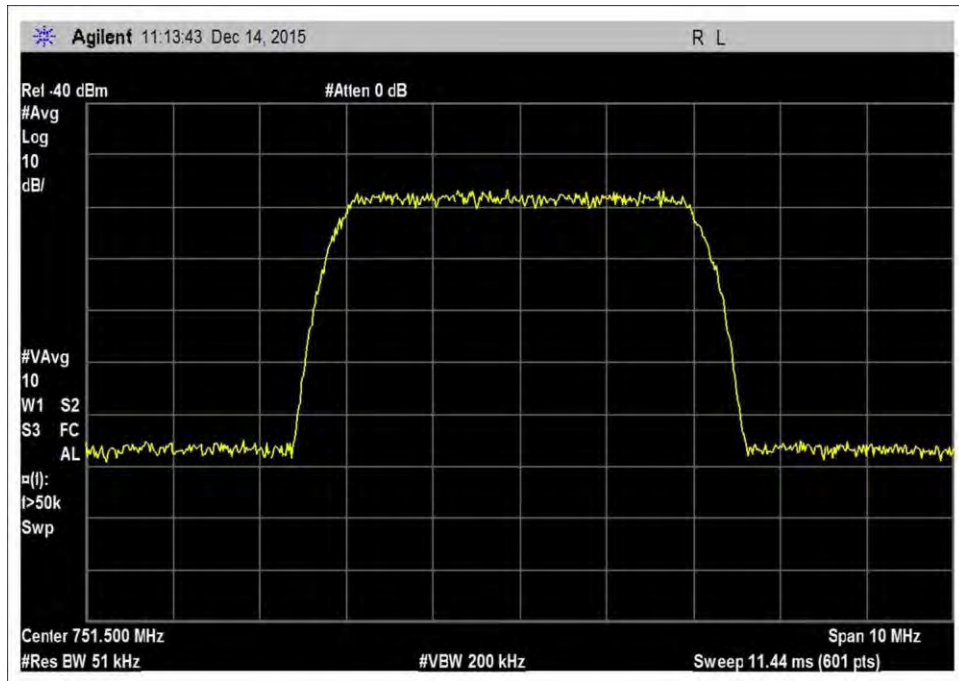
7.10_OBW_DL_746-757MHz_WCDMA
