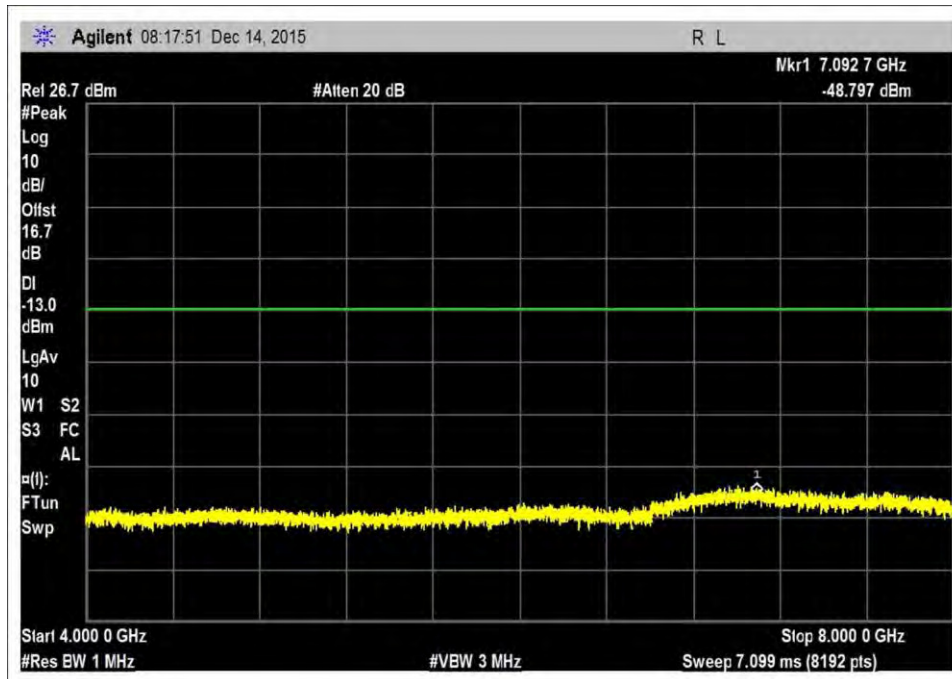
UL_1710-1755R2
