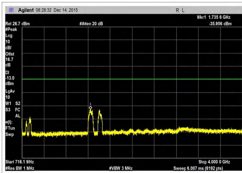
UL_698-716R1
