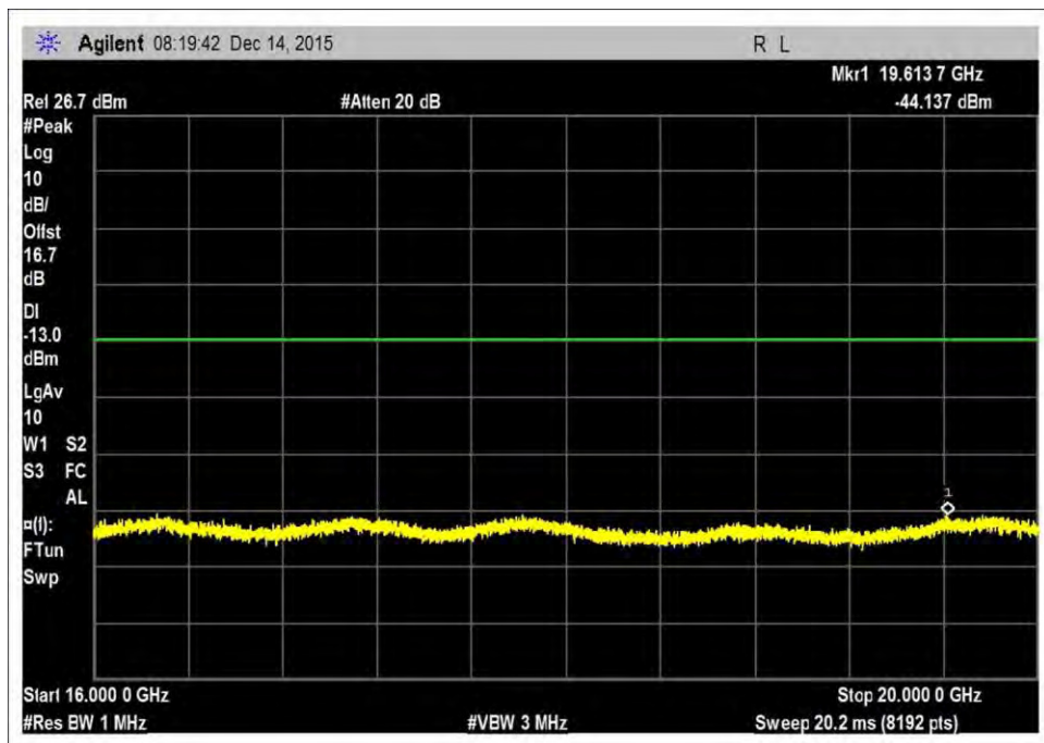
UL_1710-1755R5
