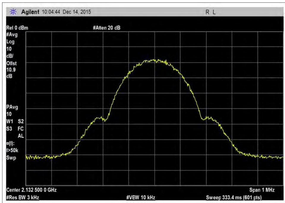
7.10_OBW_DL_2110-2155MHz_GSM
