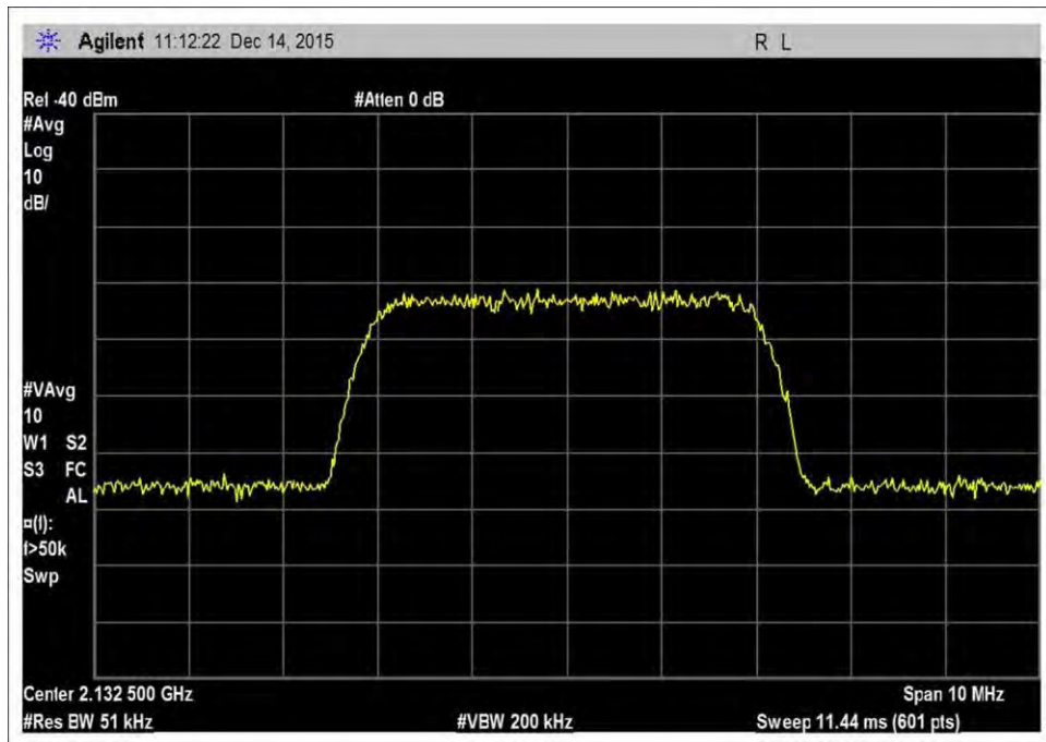
7.10_OBW_DL_2110-2155MHz_WCDMA
