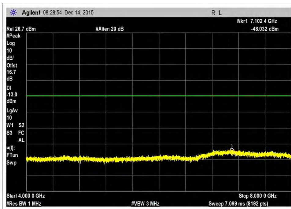
UL_698-716R2
