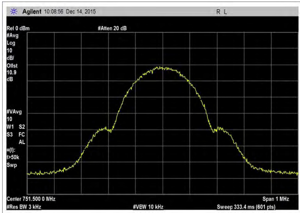
7.10_OBW_DL_746-757MHz_GSM
