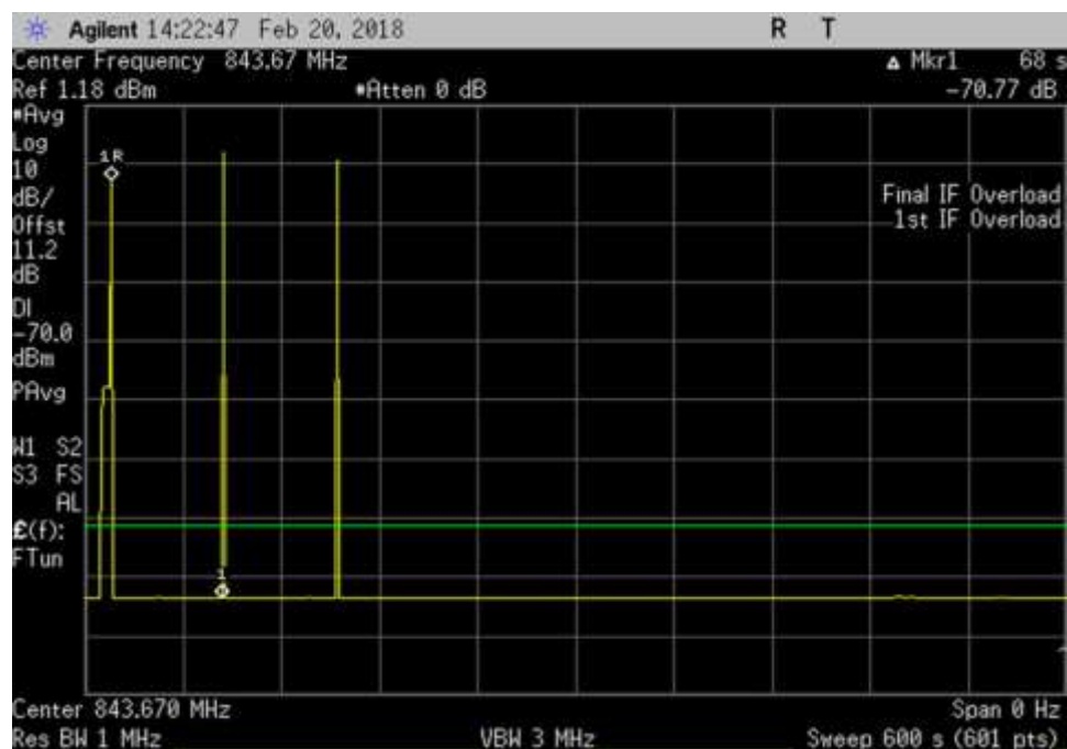
UL_824-849_600sec_ 843.67MHz
