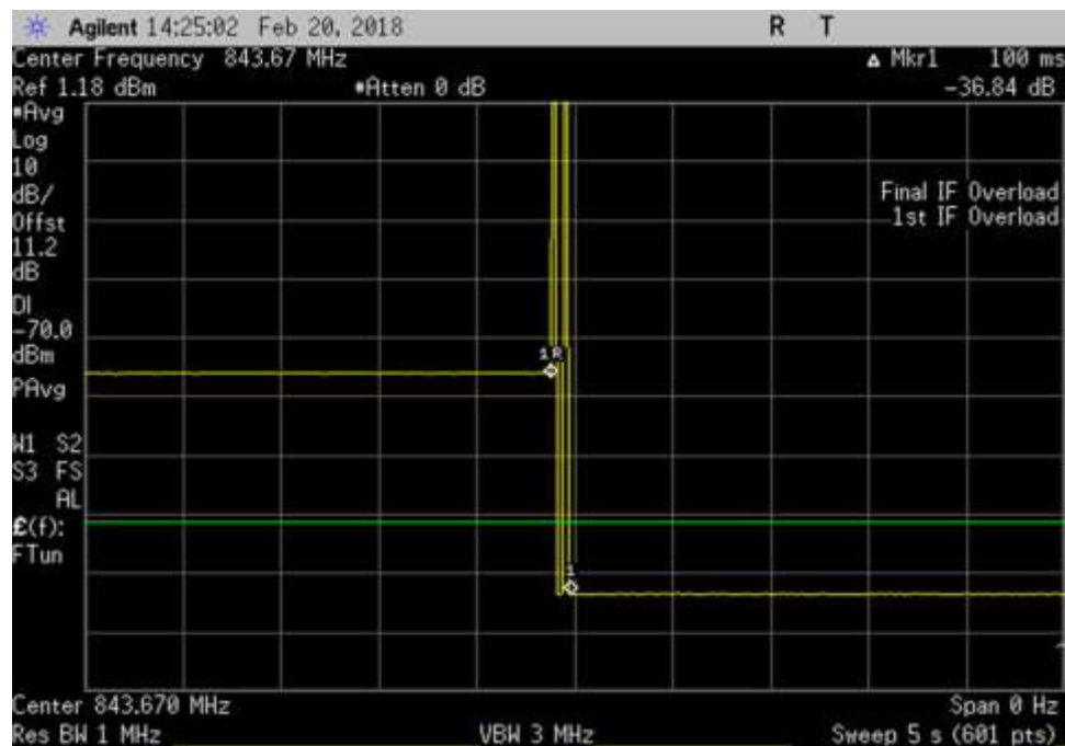
UL_824-849_ 843.67MHz_Time
