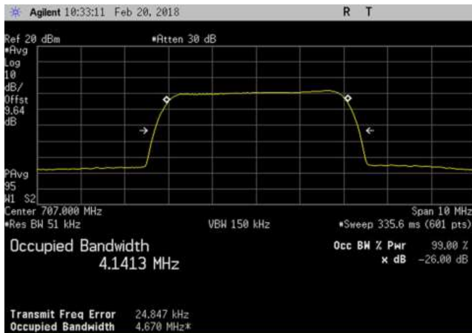
UL_698-716_AWGN_707MHz
