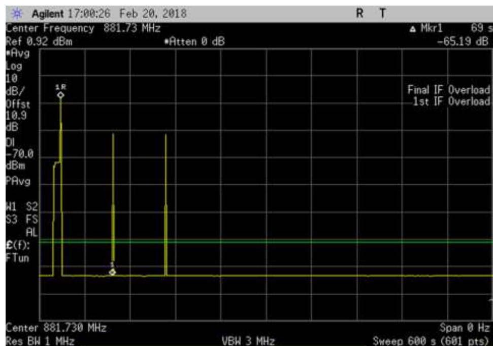
DL_869-894_600sec_ 881.73MHz
