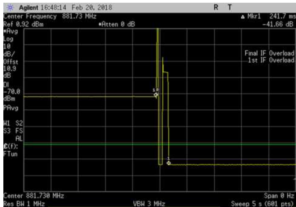
DL_869-894_ 881.73MHz_Tlme
