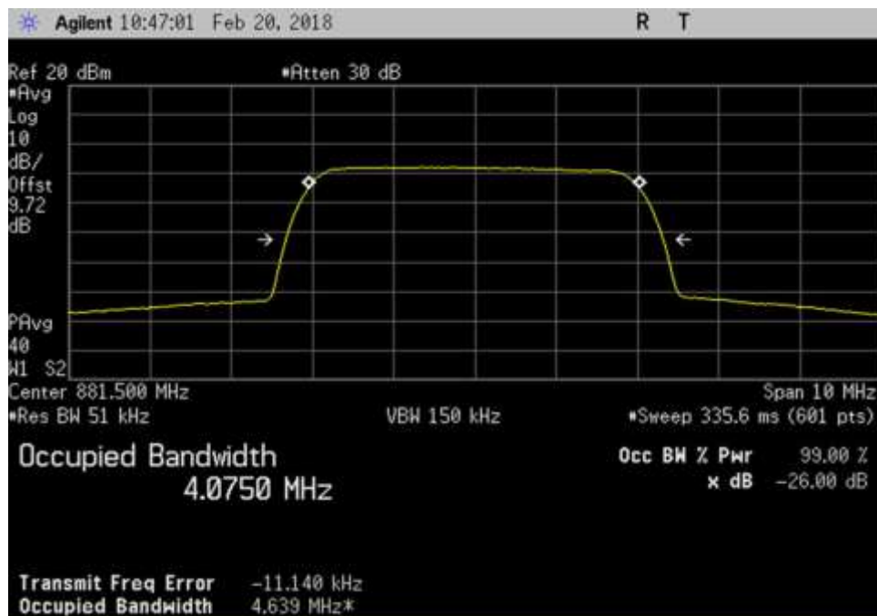
DL_869-894_AWGN_881.5MHz
