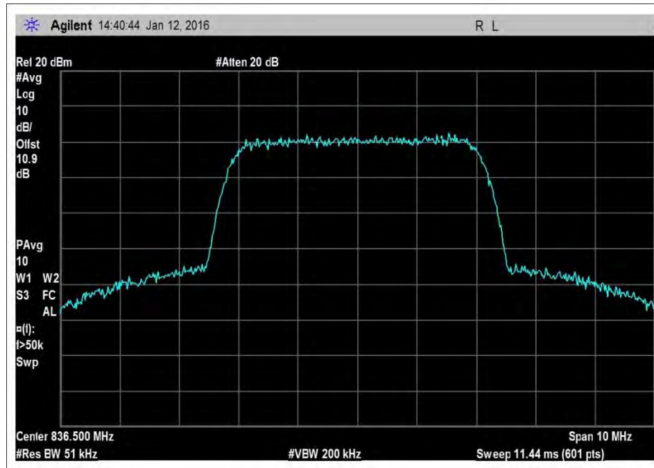
7.10_OBW_UL_824-849MHz_WCDMA
