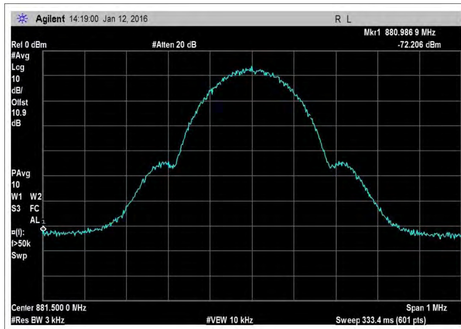
7.10_OBW_DL_869-894MHz_GSM
