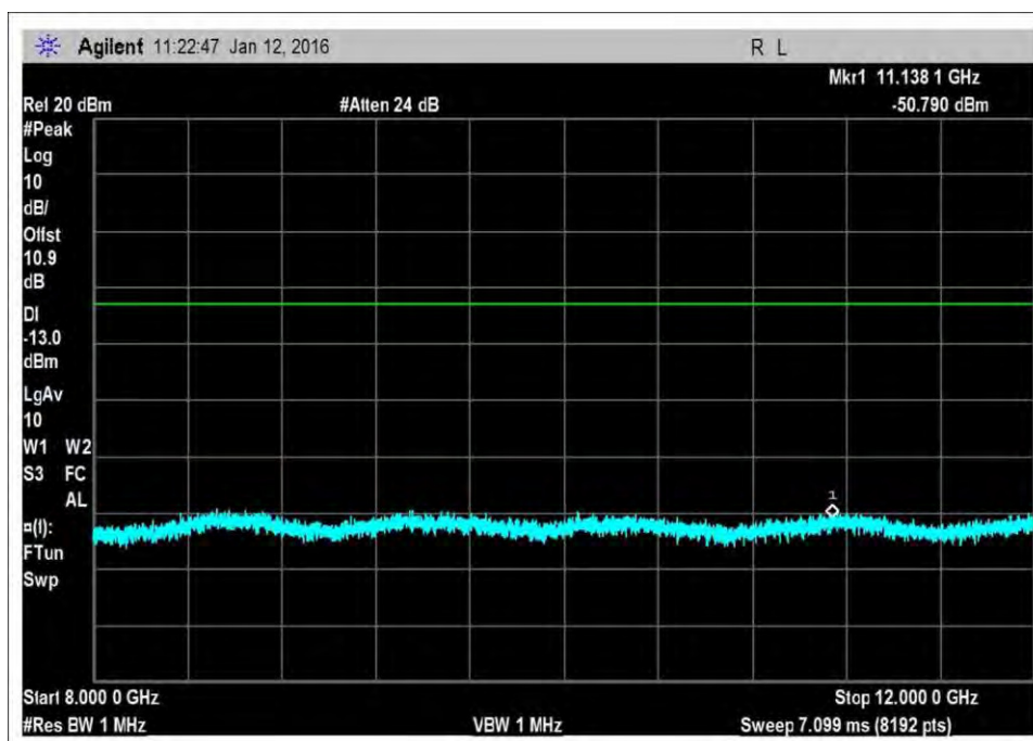
DL_869-894R3
