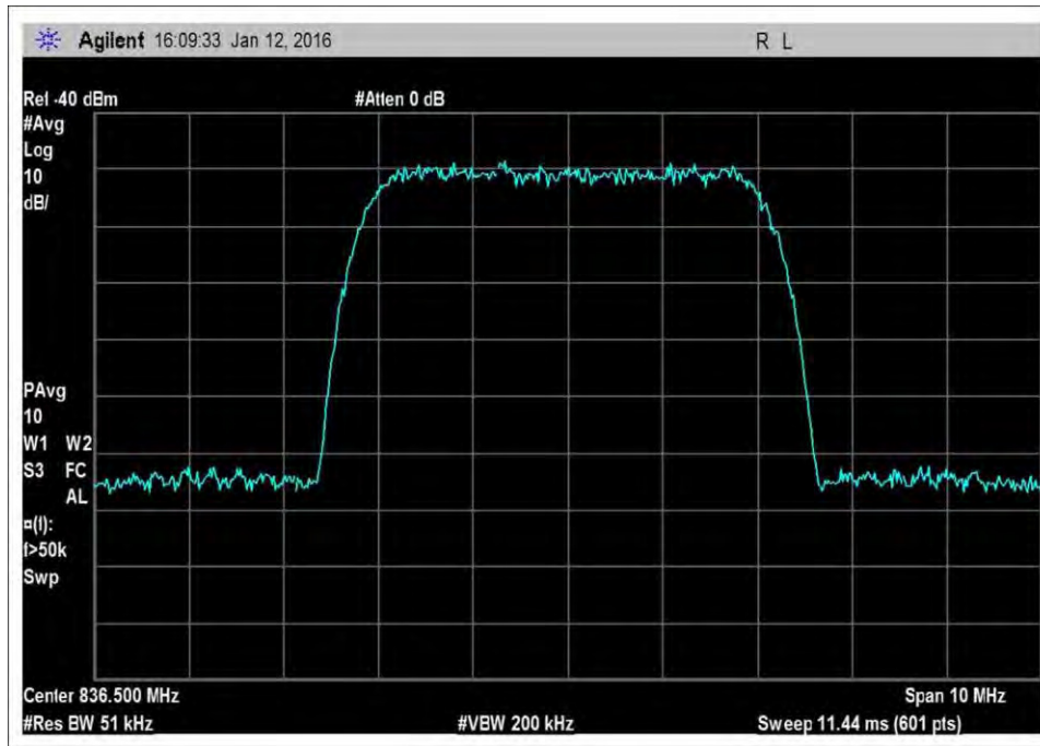
7.10_OBW_UL_824-849MHz_WCDMA
