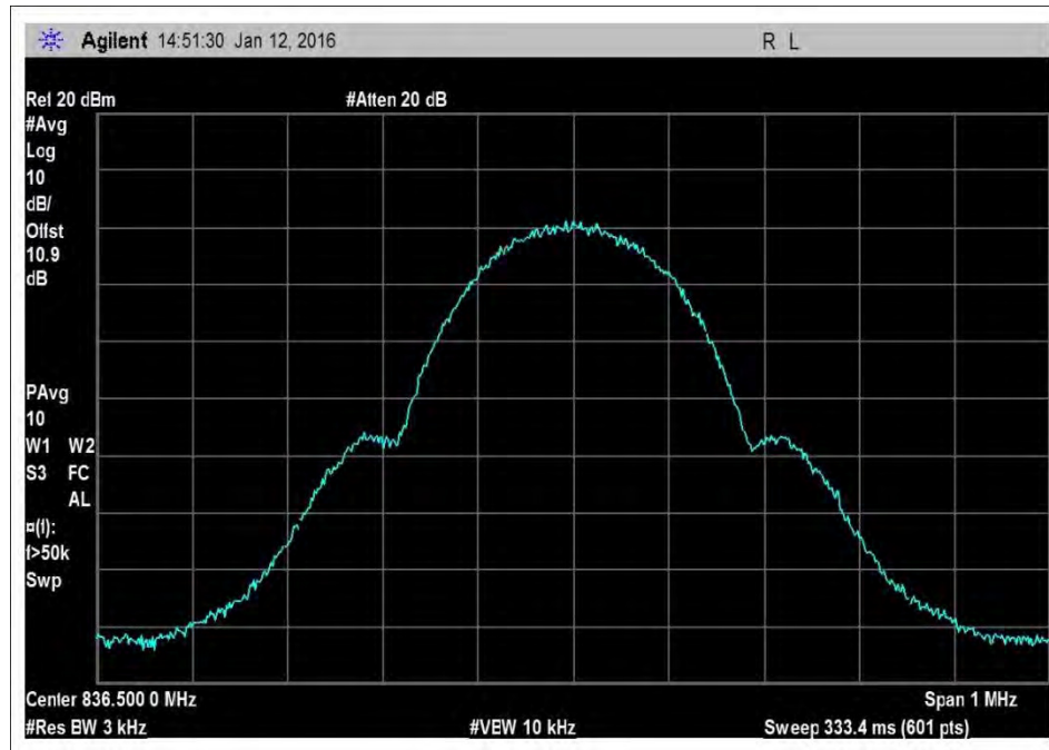
7.10_OBW_UL_824-849MHz_GSM
