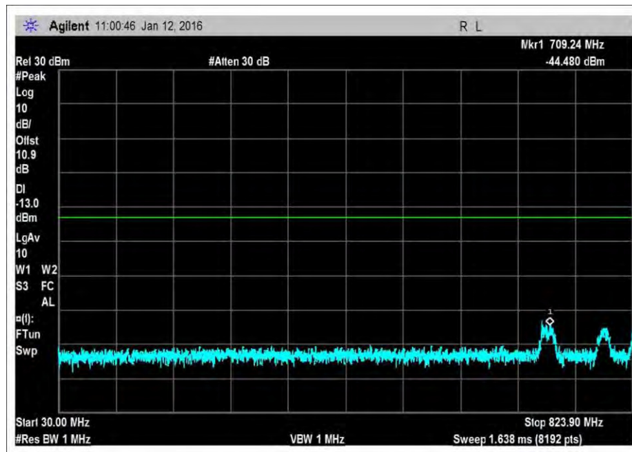
UL_824-849L
