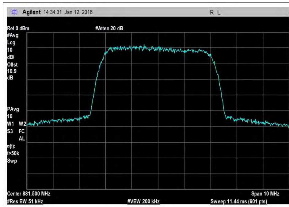
7.10_OBW_DL_869-894MHz_WCDMA
