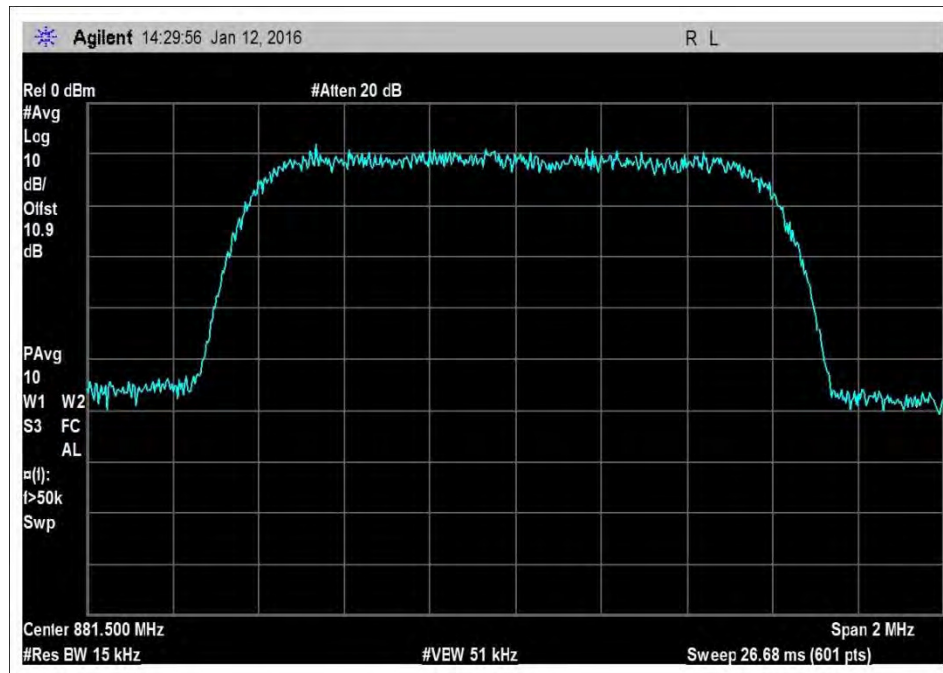
7.10_OBW_DL_869-894MHz_CDMA
