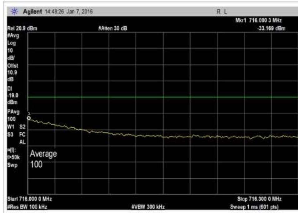
7.5_OBE_UL_698-716MHz_H_Max
