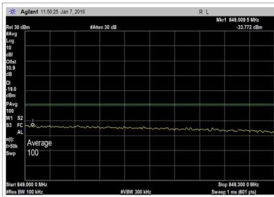
7.5_OBE_UL_824-849MHz_H_Max
