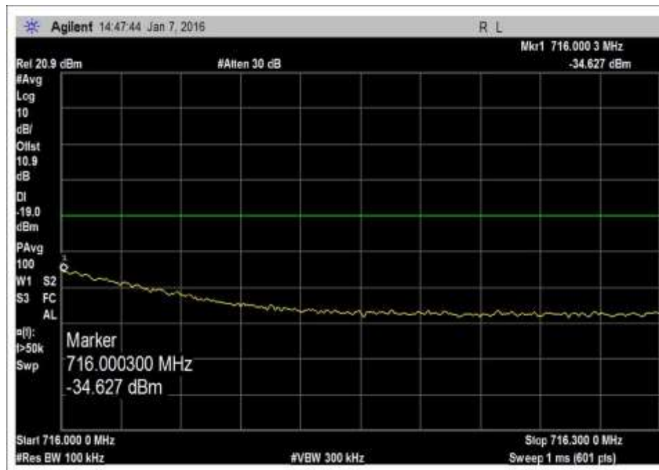
7.5_OBE_UL_698-716MHz_H_PreAGC
