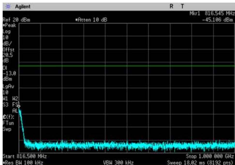
CSE_UL_806-816_816.5- 1000MHz_HC
