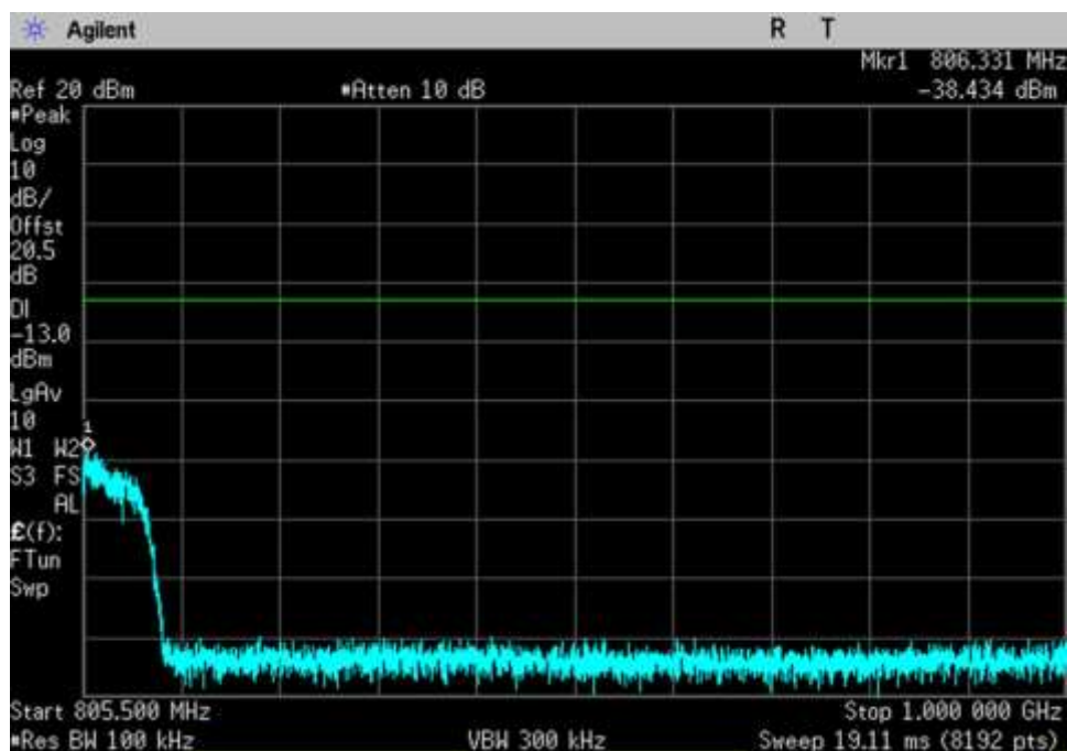
CSE_UL_799-805_ 805.5- 1000MHz_MC
