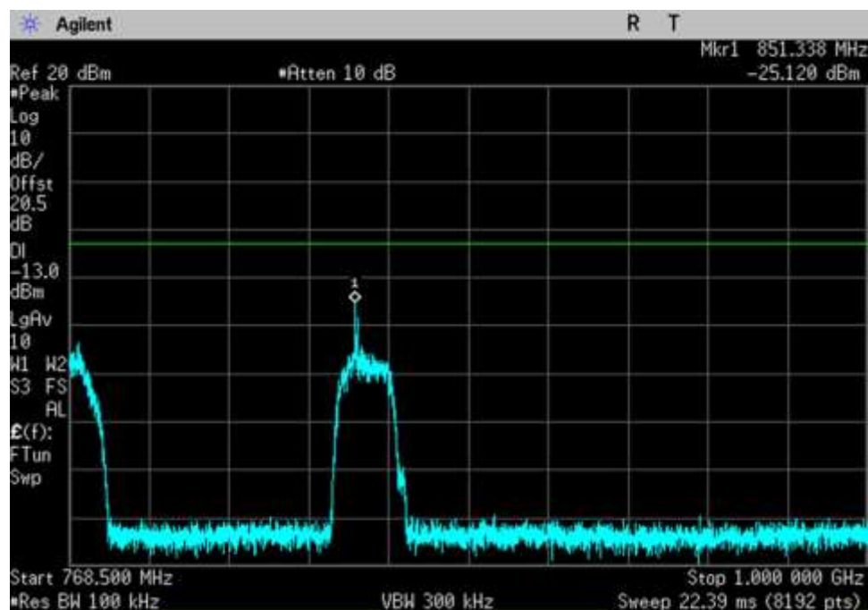
CSE_DL_758-768_ 768.5- 1000MHz_MC
