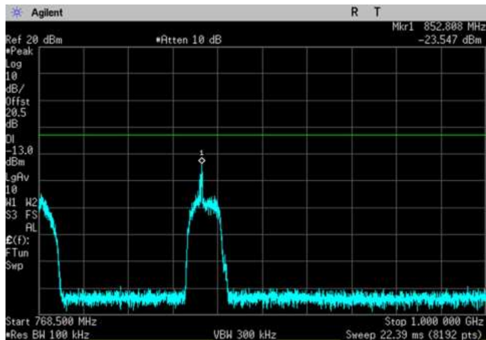
CSE_DL_758-768_ 768.5- 1000MHz_LC
