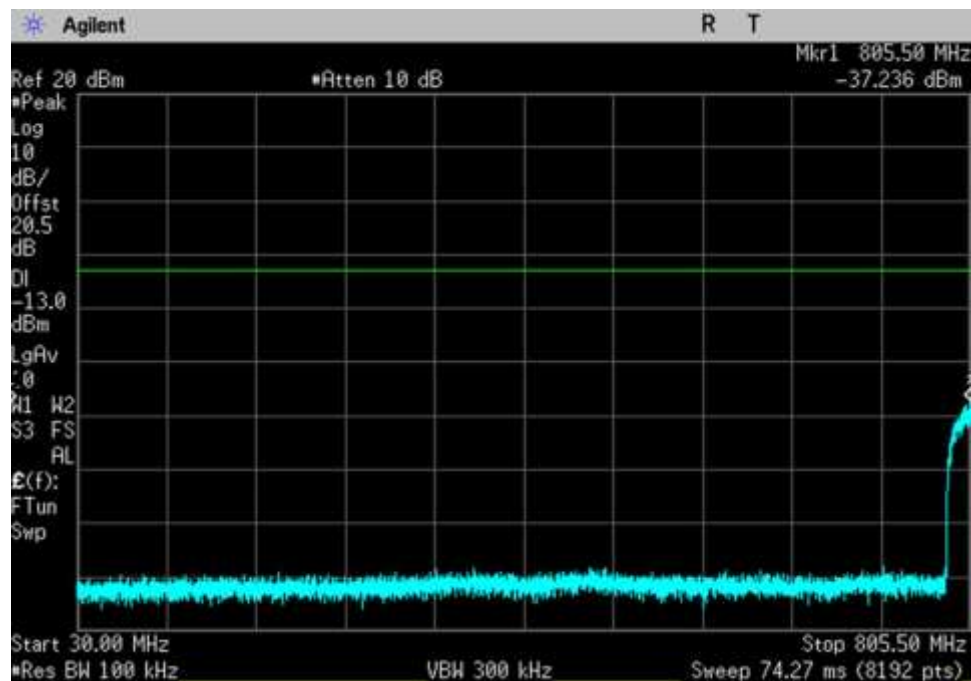
CSE_UL_806-816_30- 805.5MHz_MC
