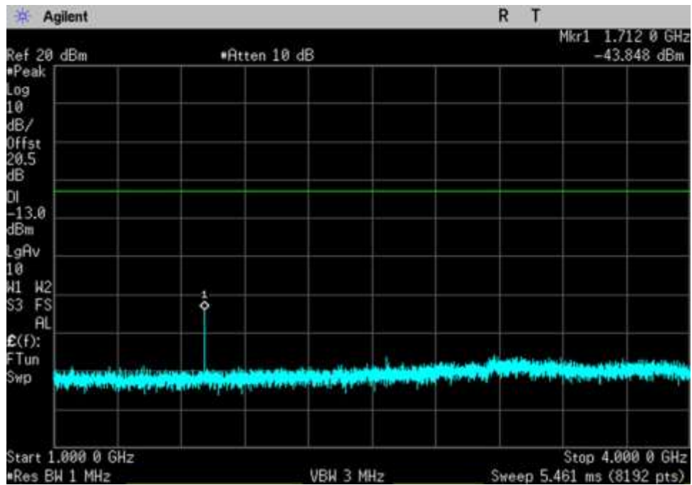
CSE_DL_851-861_ 1000- 4000MHz_MC
