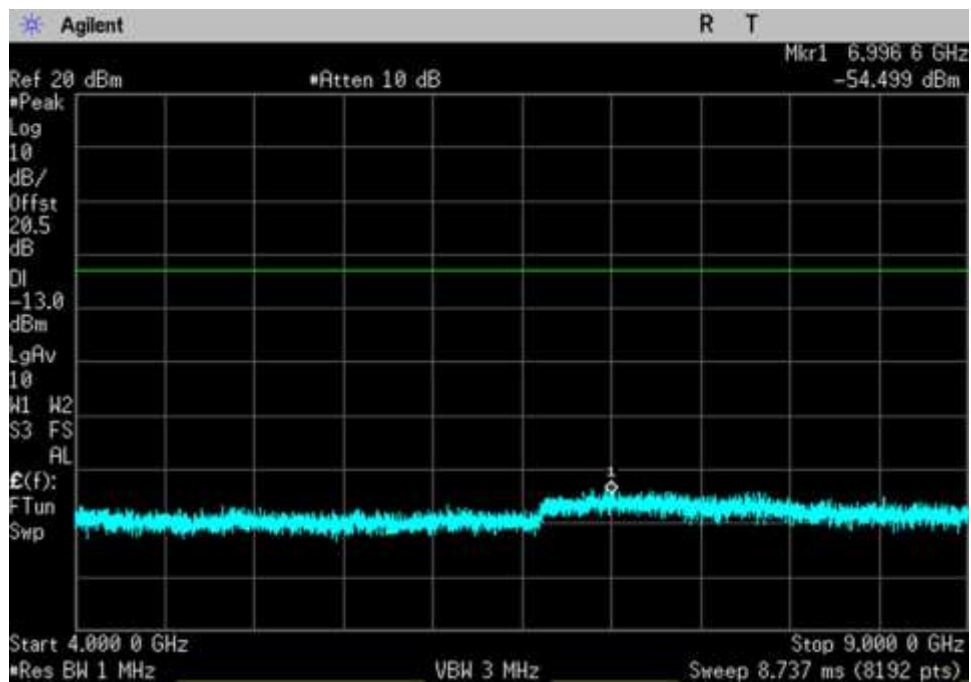
CSE_DL_851-861_ 4000- 9000MHz_HC
