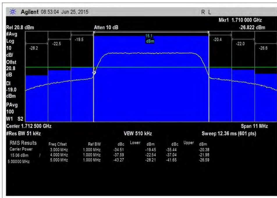
UL_1710-1755MHz_L_Max
