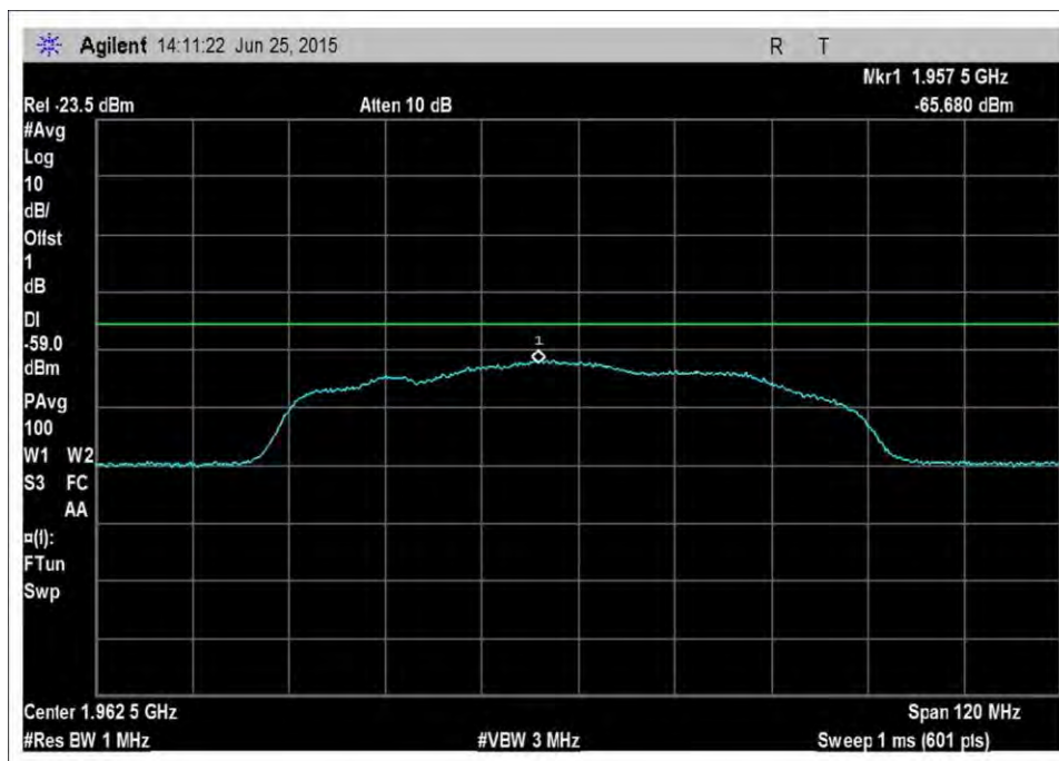
DL_1930-1995MHz_a-g_Noise_50
