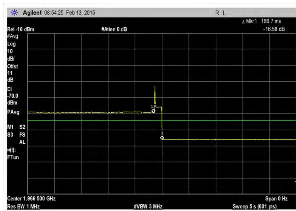
DL_1930-1995MHz_a-g_timing
