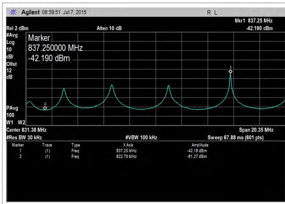
UL_824-849MHz-AWGNR+1
