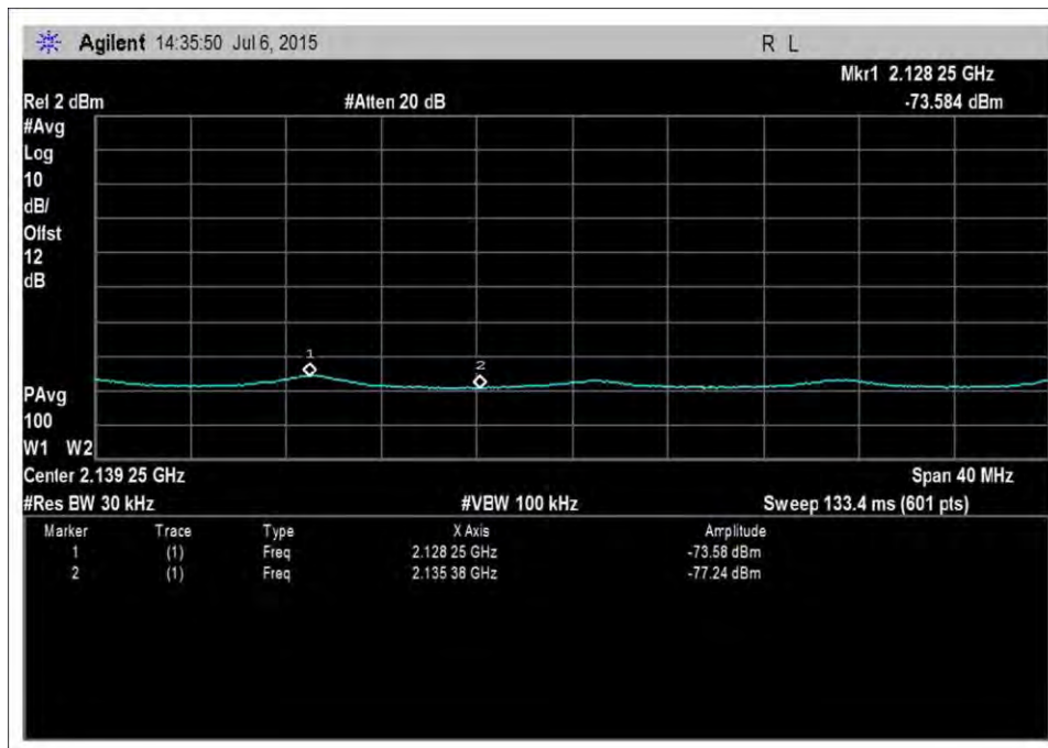
DL_2110-2155MHz-AWGNL+5
