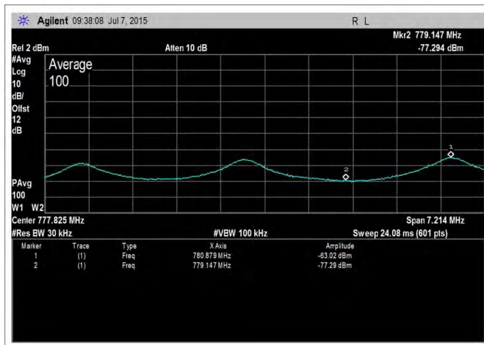
UL_776-787MHz-AWGNR+3
