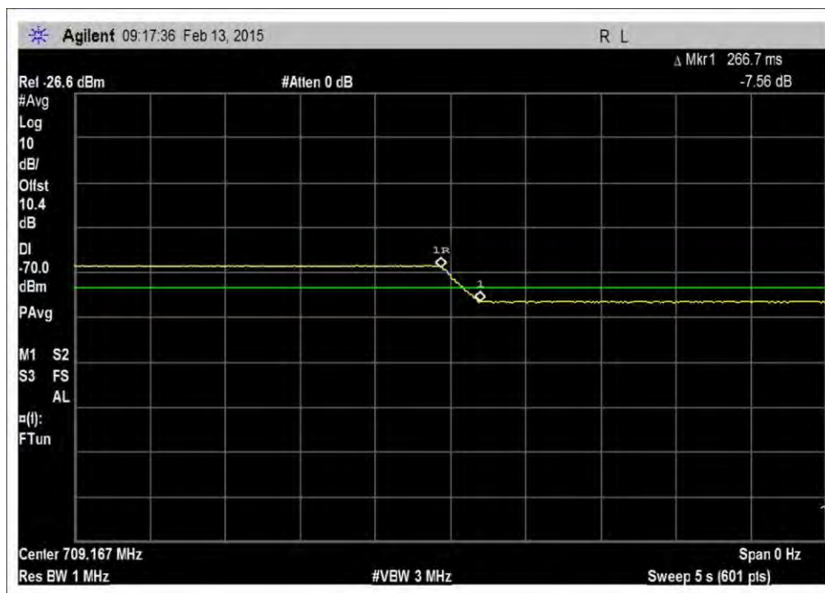
UL_698-716MHz_a-g_timing
