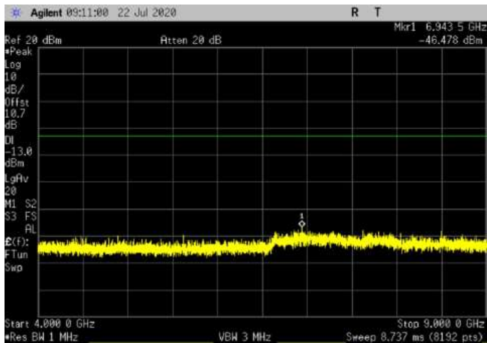
UL_809-816_4000-9000MHz_MC
