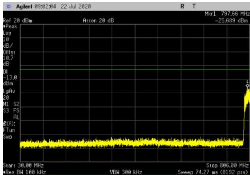
UL_806-809_ 30- 806MHz_MC
