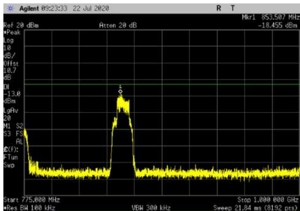
DL_769-775_ 775- 1000MHz_MC
