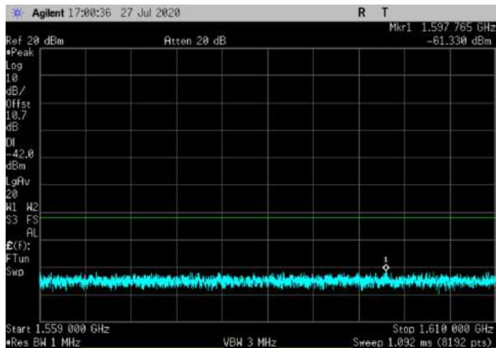
UL_799-805_1559-1610MHz_MC
