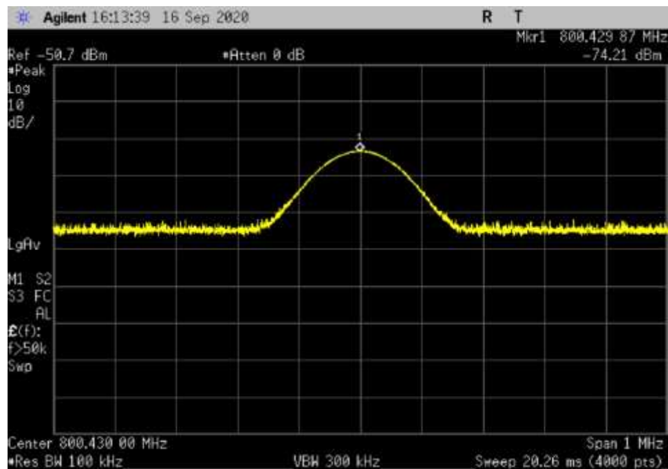
UL_799-805-CW-Input_ 800.43MHz
