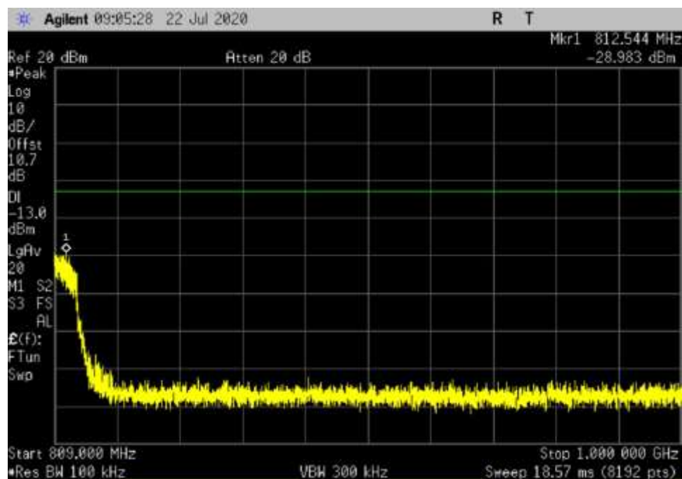
UL_806-809_ 809- 1000MHz_MC
