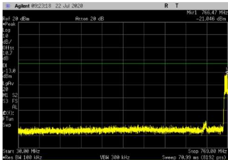
DL_769-775_ 30- 769MHz_MC
