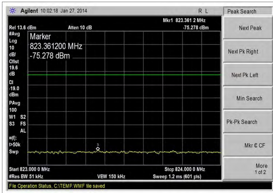
UL_824-849MHz_Low CH_CDMA_10dbm
