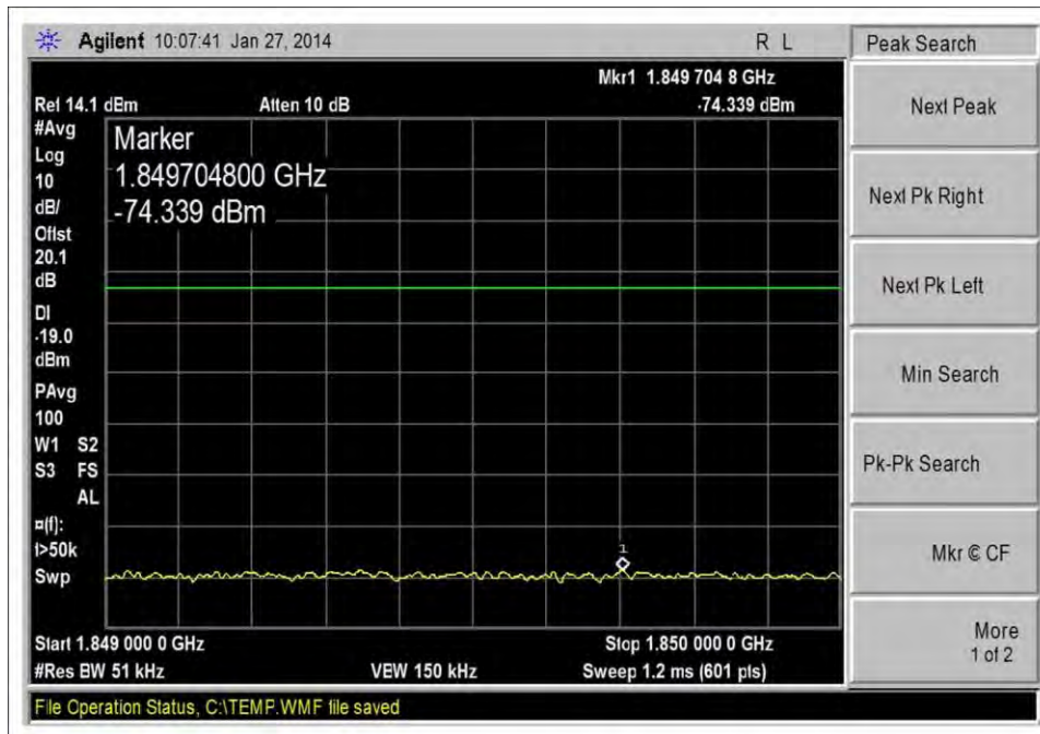
UL_1850-1910MHz_Low CH_CDMA_10dbm
