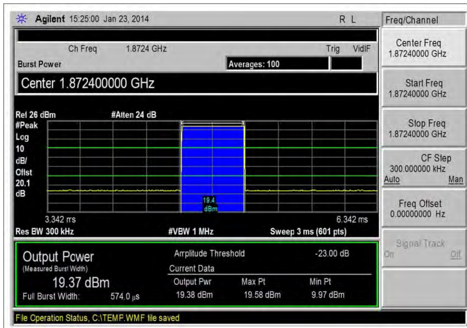
UL_1850-1910_GSM
