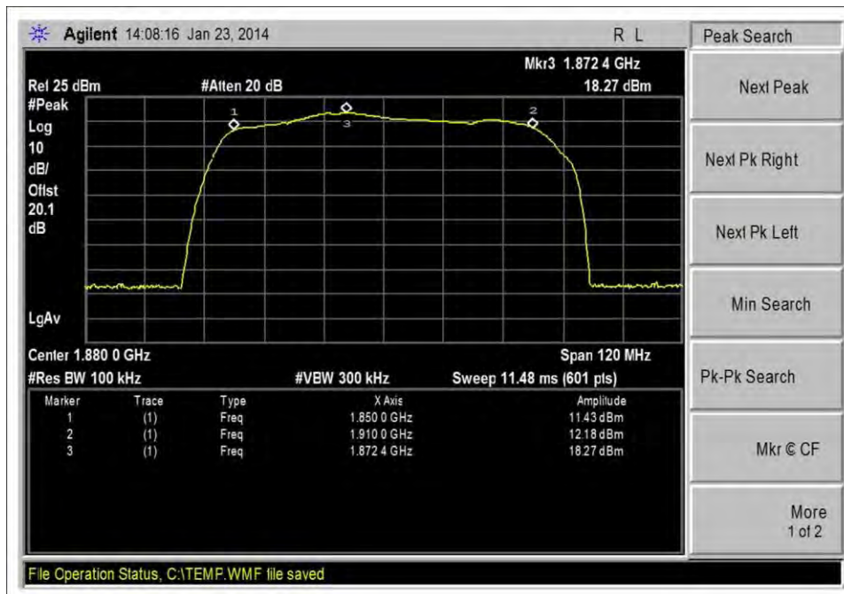
UL_1850-1910MHz
