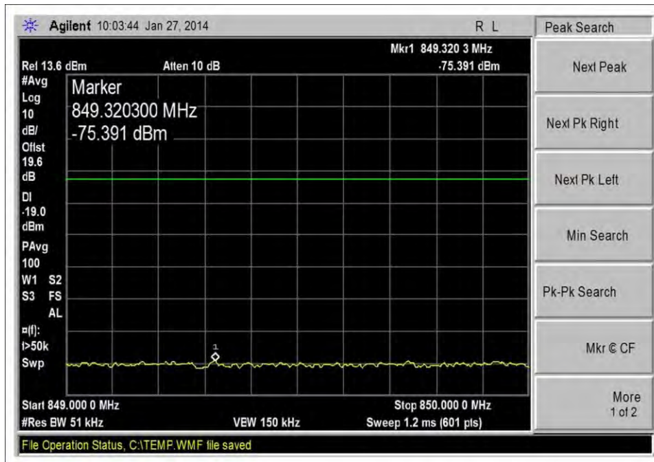
UL_824-849MHz_Hi CH_CDMA_10dbm
