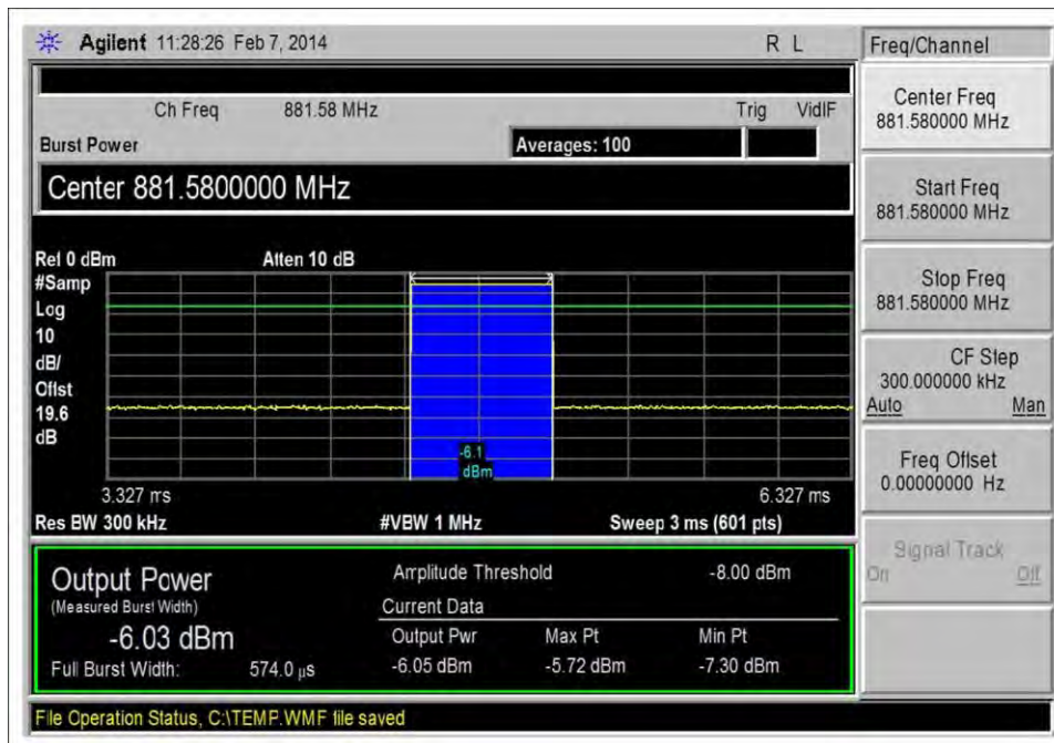
DL_869-894_GSM
