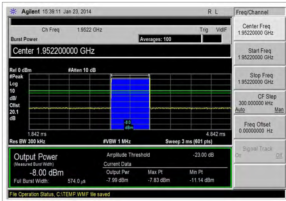
DL_1930-1990_GSM
