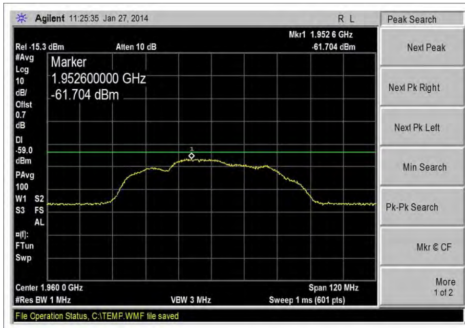
Max Noise_DL_1930-1990MHz
