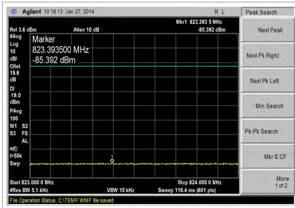
UL_824-849_Low CH_GSM_10dbm
