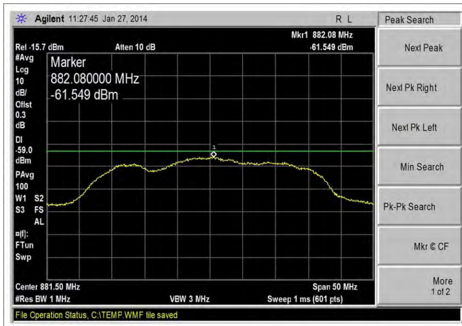
Max Noise_DL_869-894MHz
