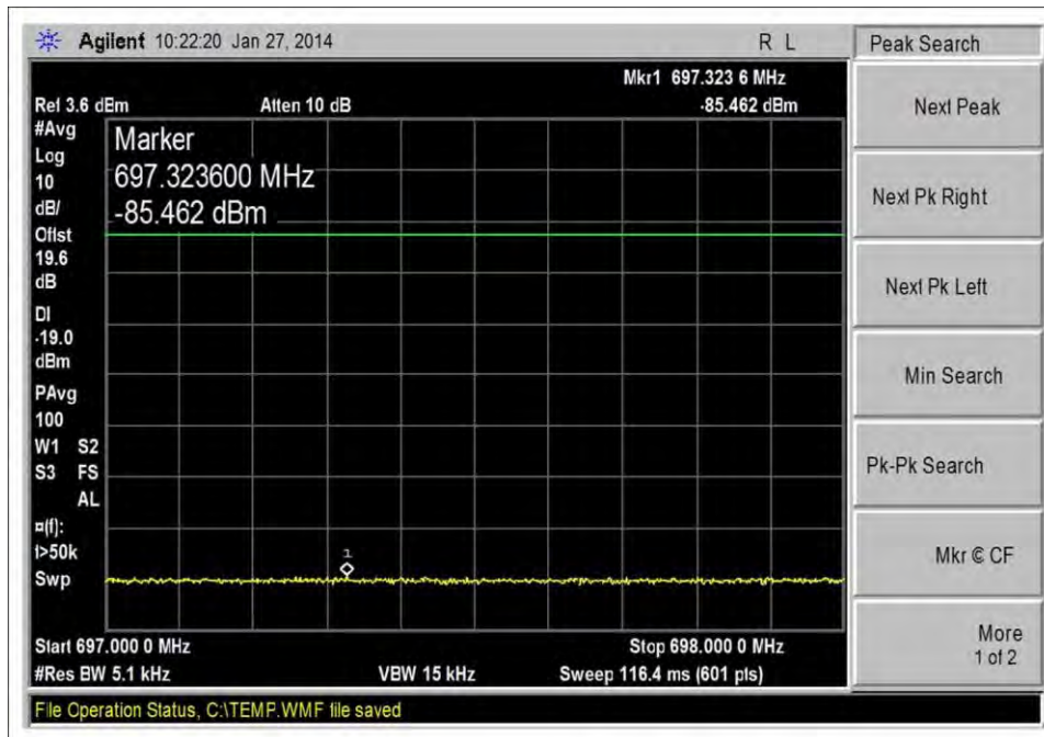
UL_698-716_Low CH_GSM_10dbm
