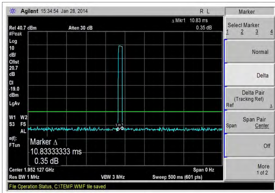
Oscillation Detectoin_DL_1930-1990MHz
