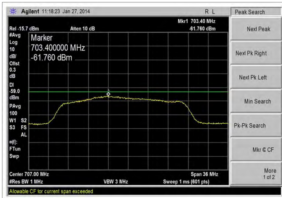
Max Noise_UL_698-716
