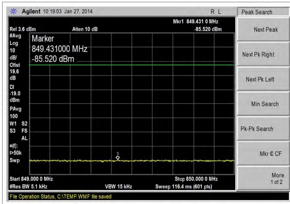
UL_824-849_Hi CH_GSM_10dbm
