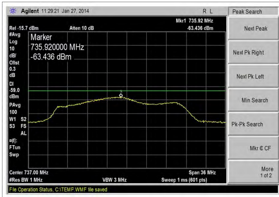
Max Noise_DL_728-746MHz
