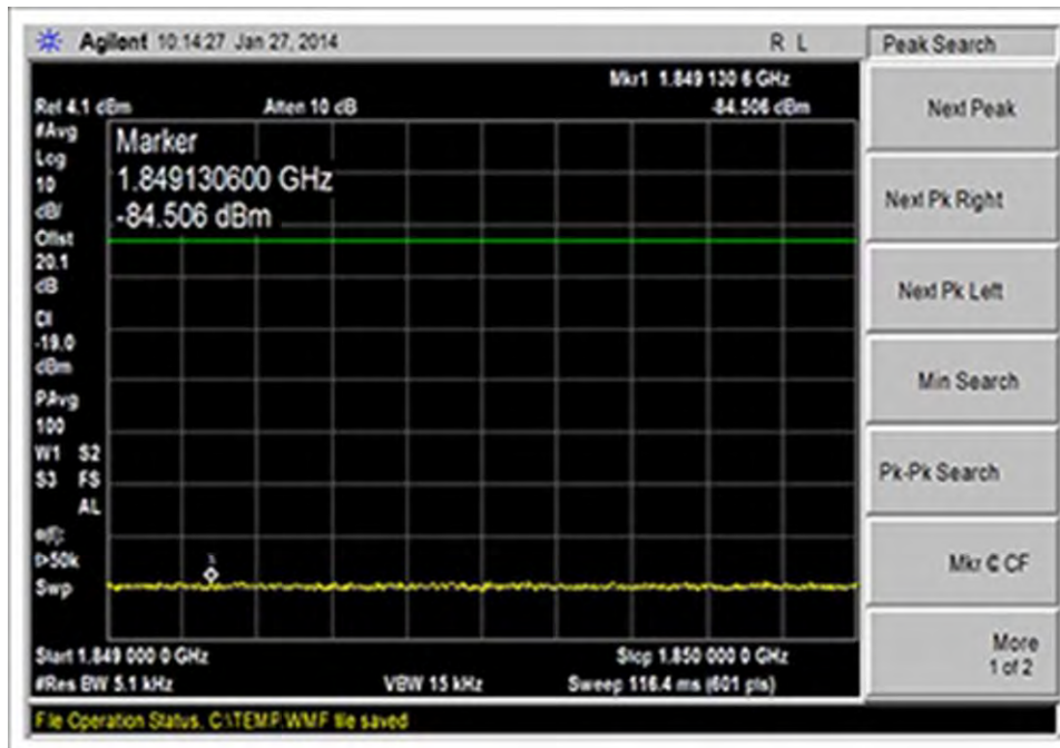
UL_1850-1910MHz_Low CH_GSM_10dbm
