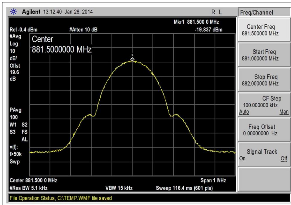
GSM_DL 869-894_Output
