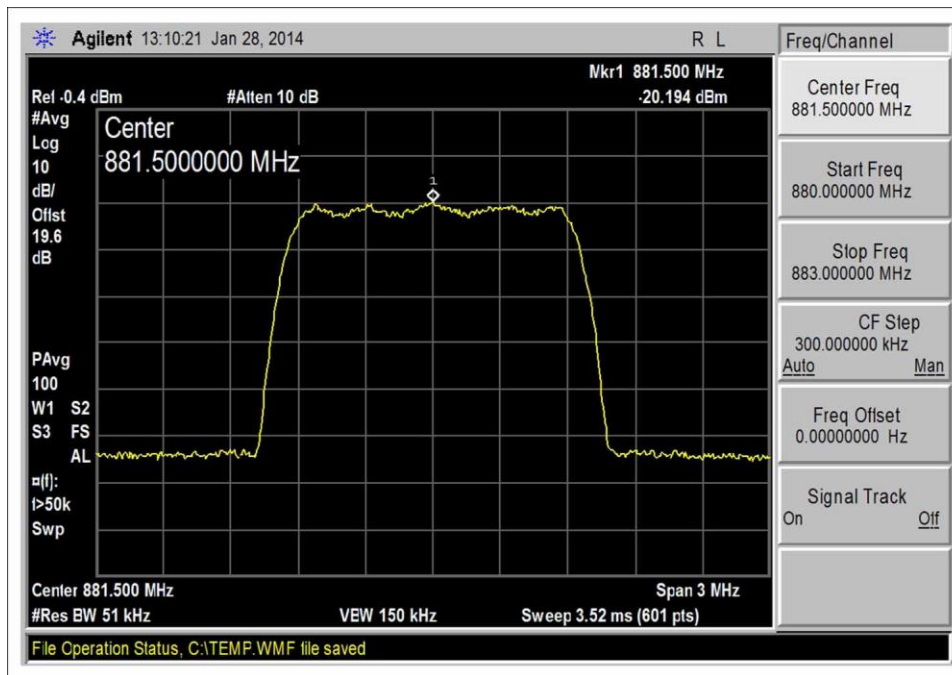
CDMA_DL 869-894_Output
