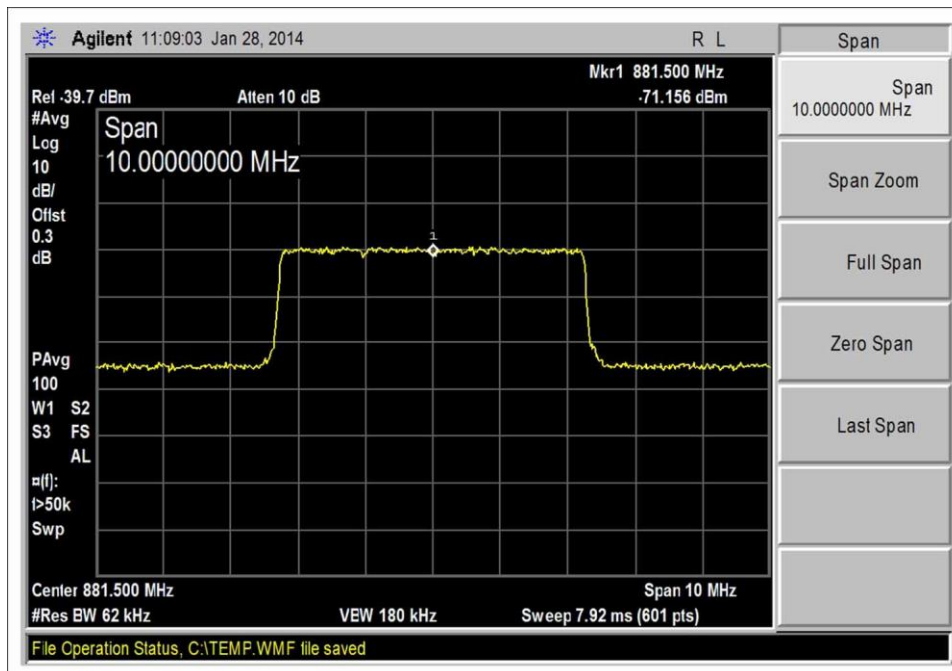
LTE_DL 869-894_Input
