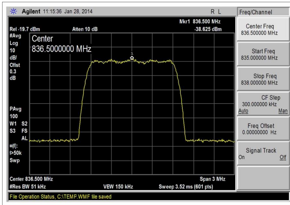
CDMA_UL 824-849_Input
