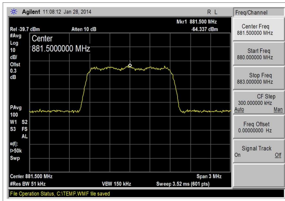
CDMA_DL 869-894_Input
