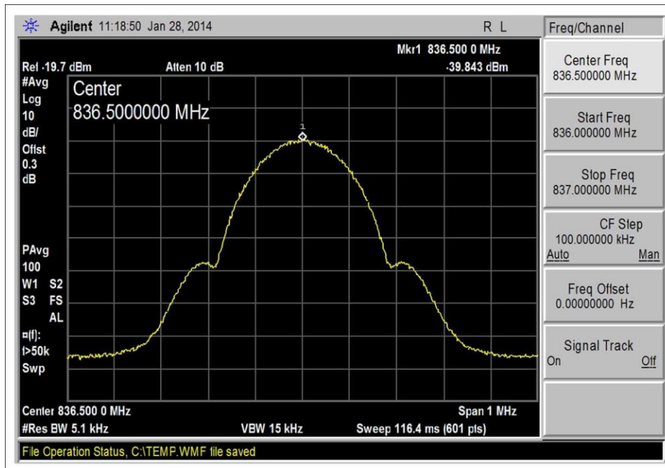
GSM_UL 824-849_Input
