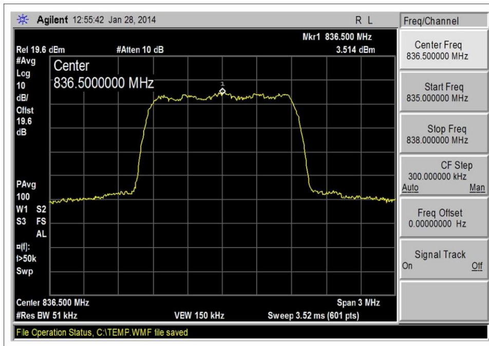
CDMA_UL 824-849_Output
