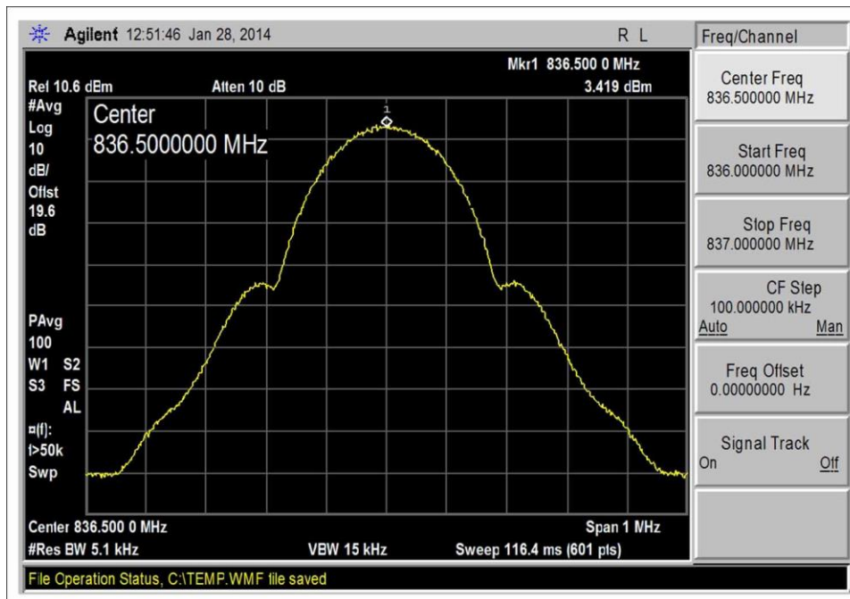
GSM_UL 824-849_Output
