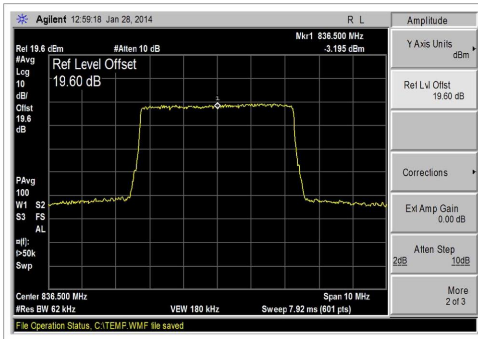
LTE_UL 824-849_Output
