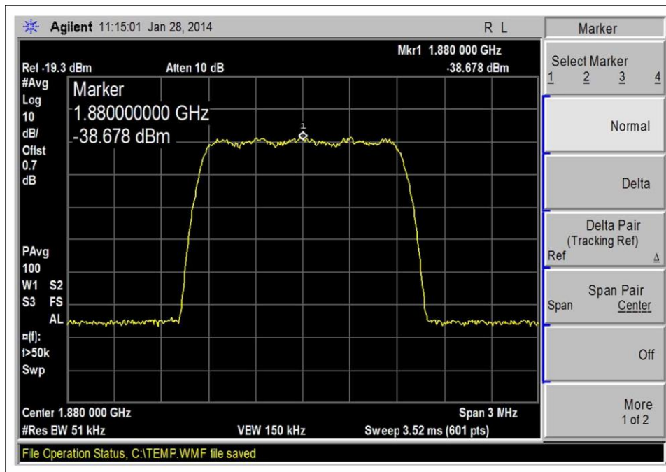
CDMA_UL 1850-1910_Input
