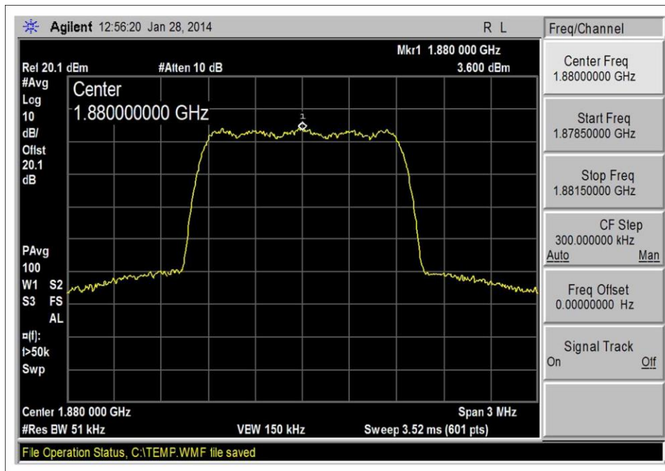
CDMA_UL 1850-1910_Output
