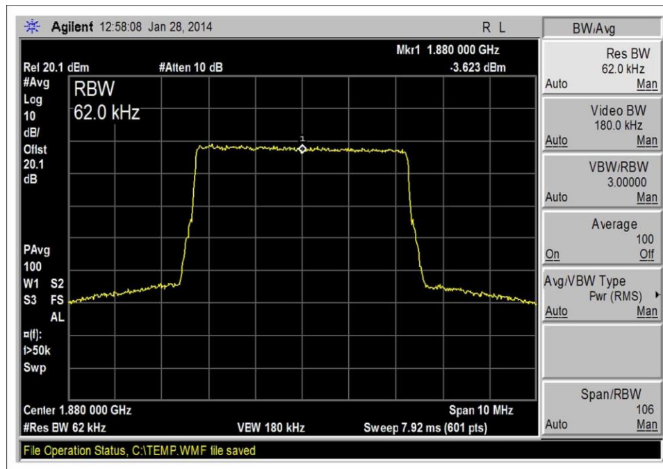
LTE_UL 1850-1910_Output
