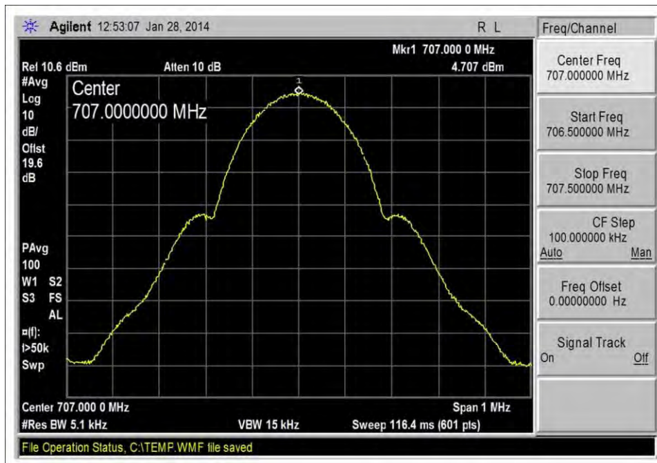
GSM_UL 698-716_Output
