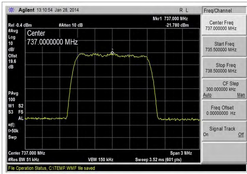
CDMA_DL 728-746_Output
