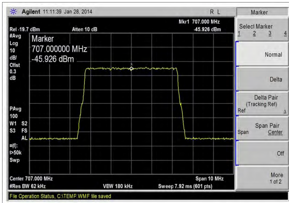
LTE_UL 698-716_Input
