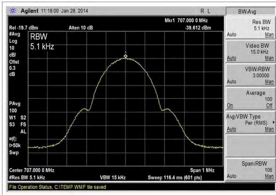
GSM_UL 698-716_Input
