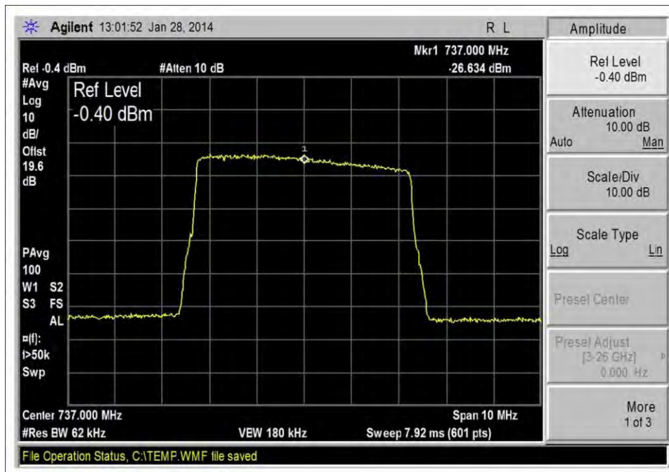
LTE_DL 728-746_Output
