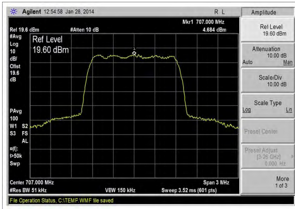
CDMA_UL 698-716_Output
