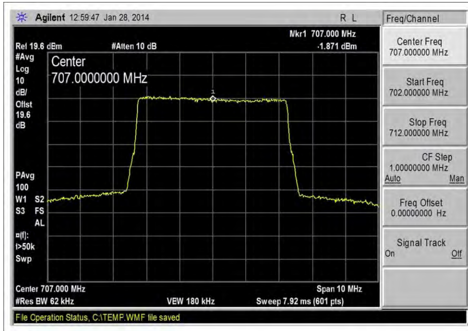
LTE_UL 698-716_Output
