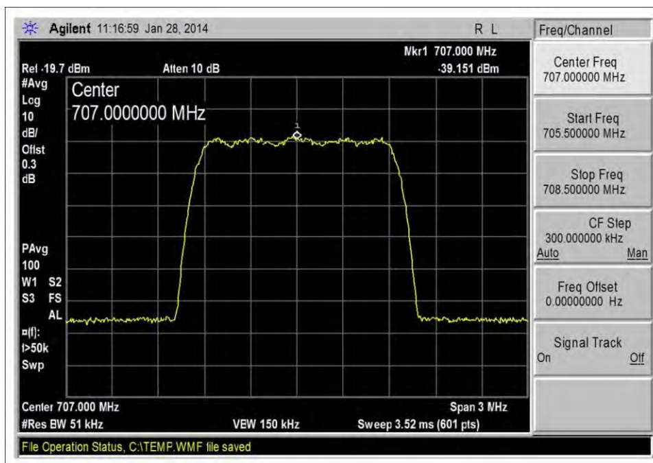
CDMA_UL 698-716_Input
