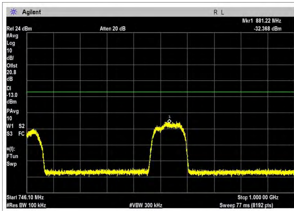
DL-728-746R-AWGN-L
