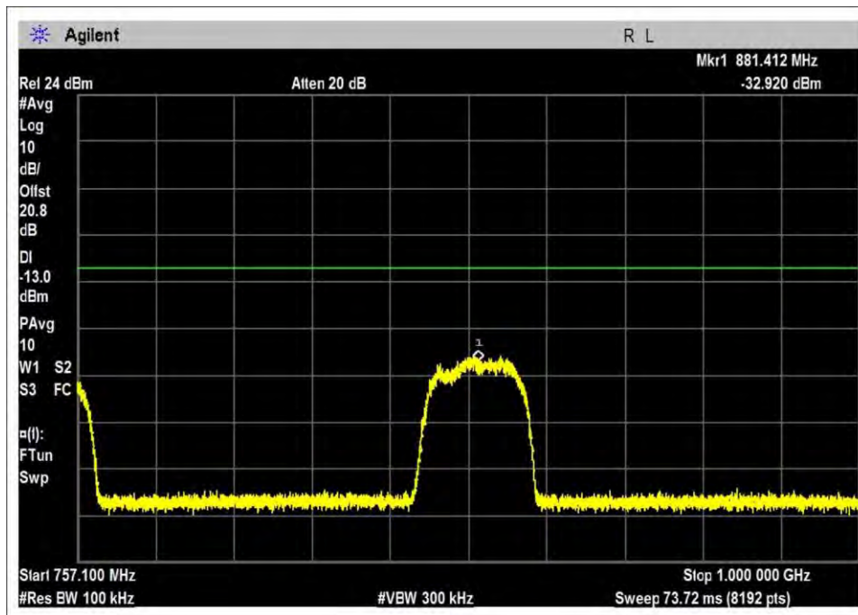
DL-746-757R-GSM-L
