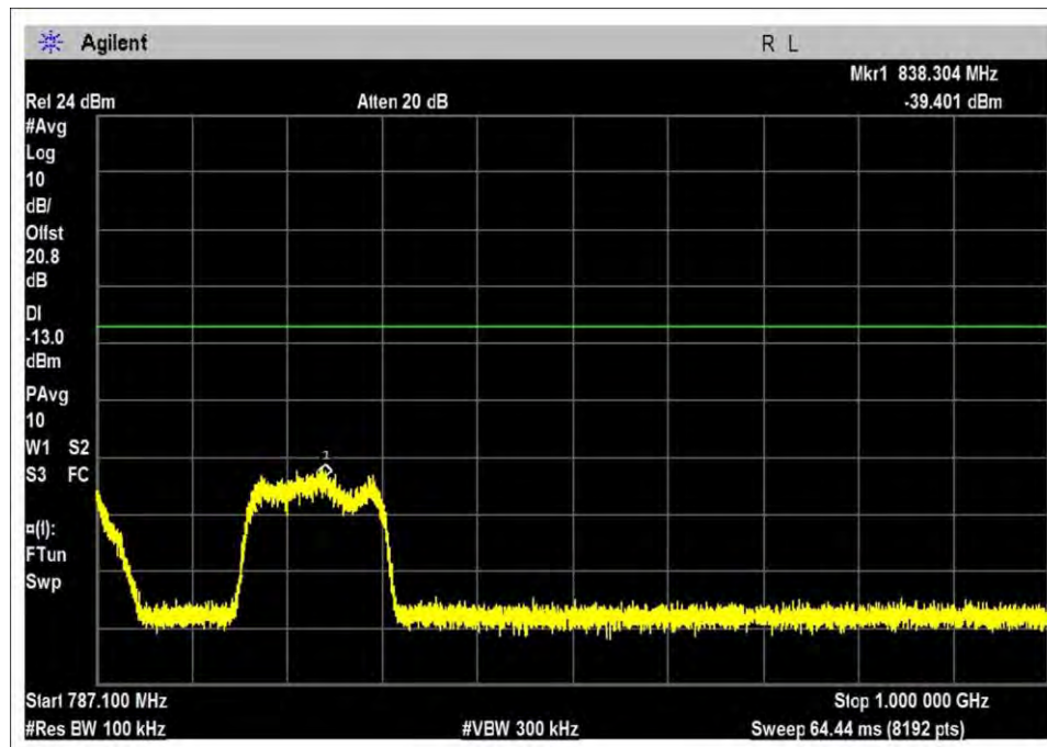
UL-776-787R-AWGN-L
