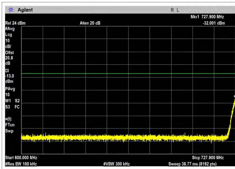
DL-728-746L-AWGN-L
