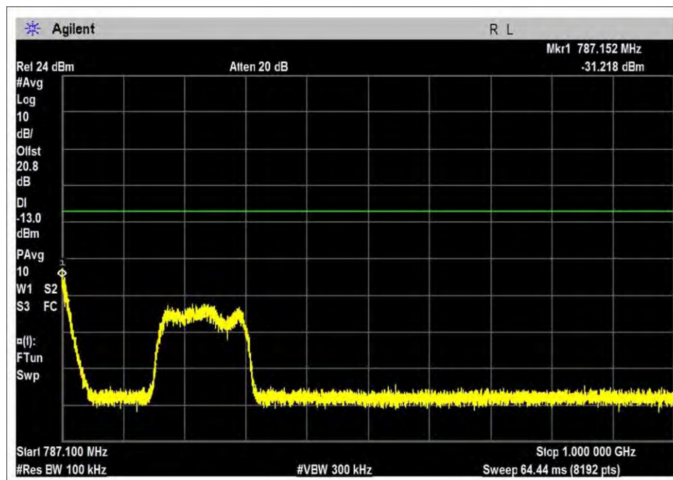
UL-776-787R-AWGN-H
