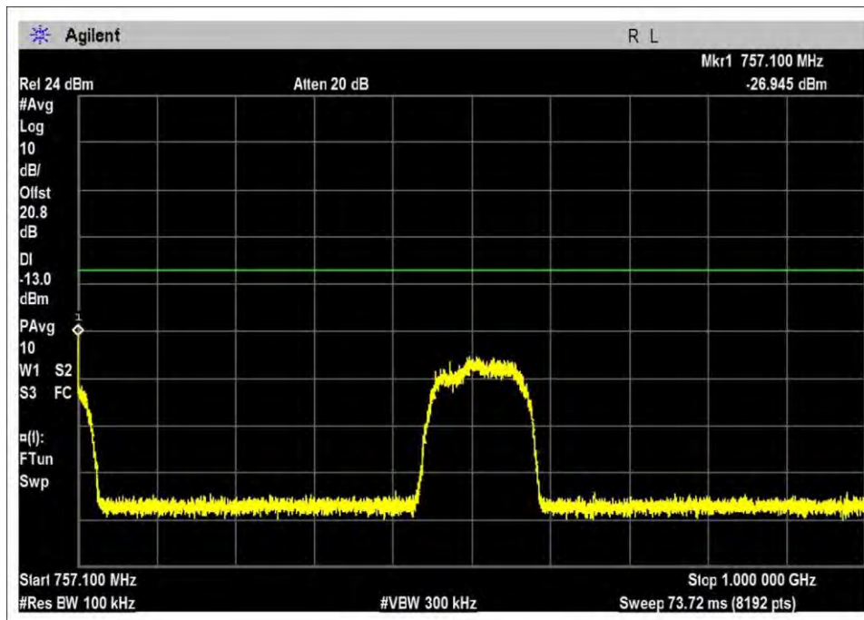
DL-746-757R-GSM-H
