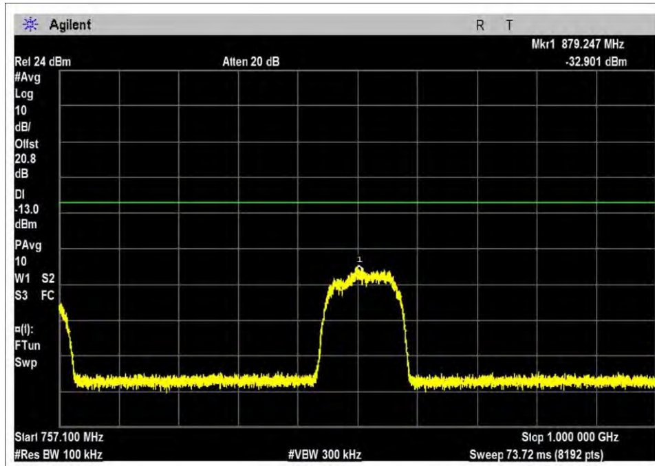
DL-746-757R-GSM-M
