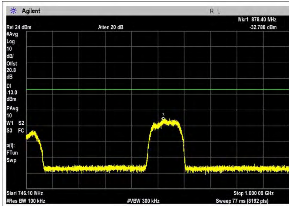
DL-728-746R-AWGN-M
