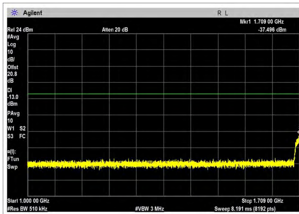
UL-1710-1755L-AWGN-M
