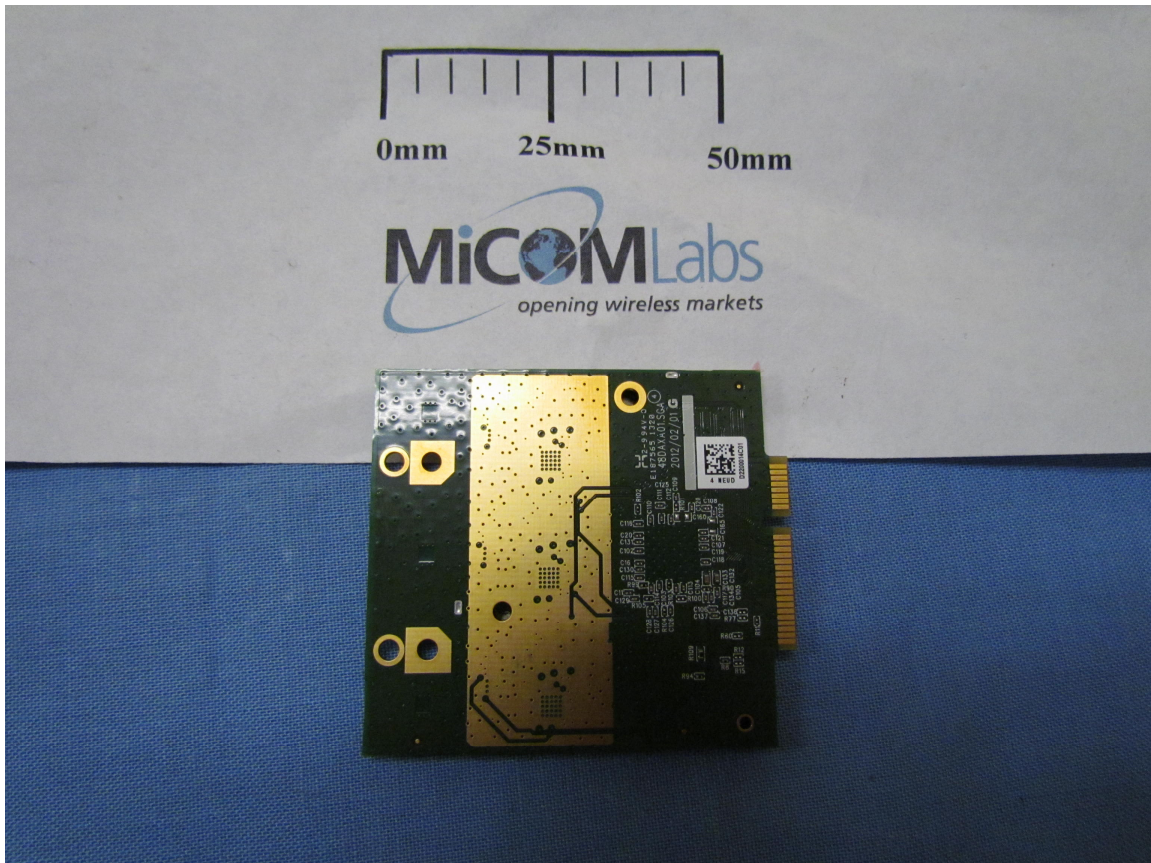
Module back
