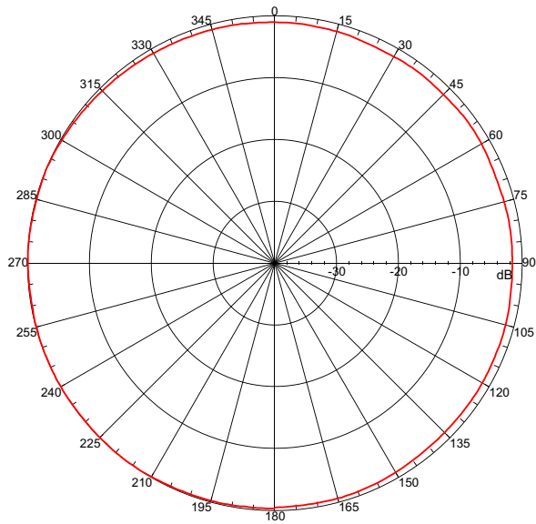
5.725 GHz H-Plane
