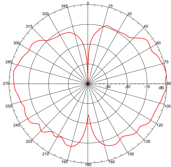
5.725 GHz E-Plane
