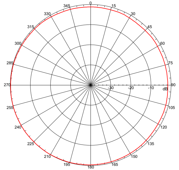
5.35 GHz H-Plane
