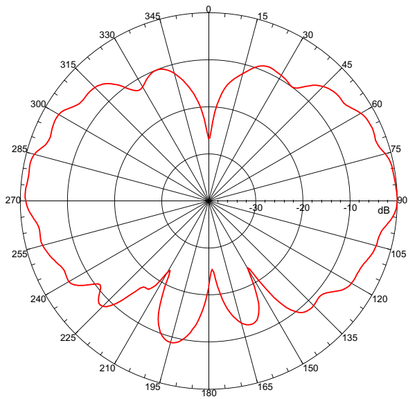
5.15 GHz E-Plane
