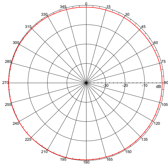
5.15 GHz H-Plane
