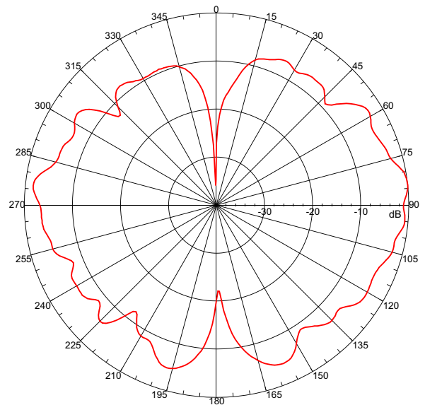
5.875 GHz E-Plane
