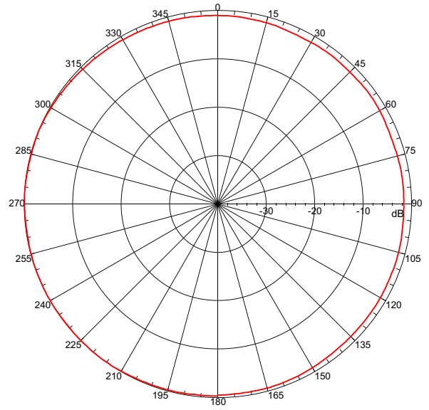
5.875 GHz H-Plane
