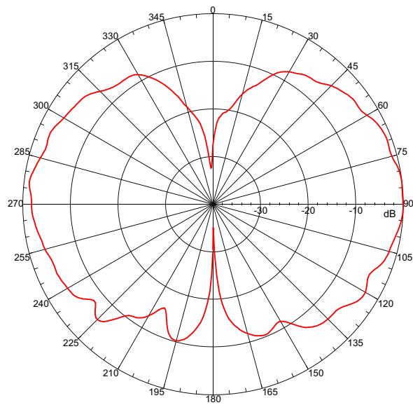
5.50 GHz E-Plane
