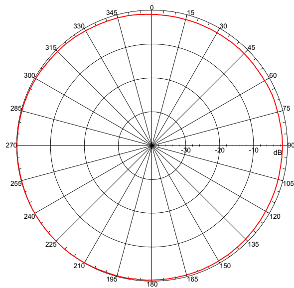
5.50 GHz H-Plane
