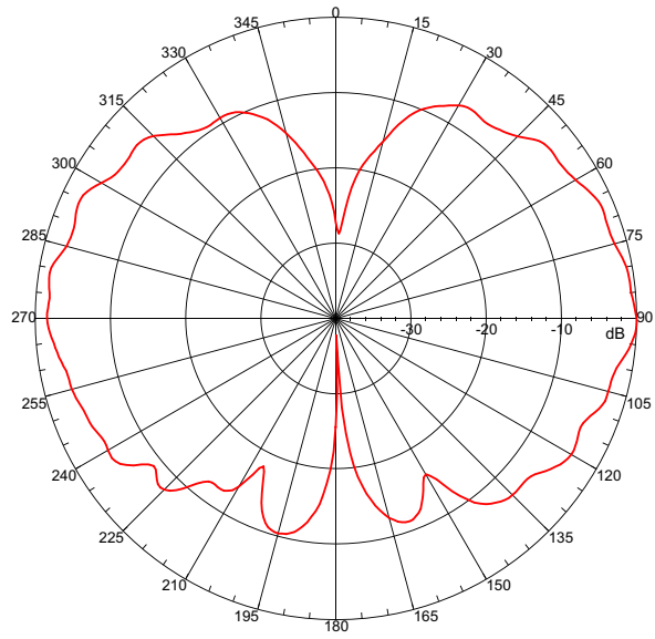
5.35 GHz E-Plane
