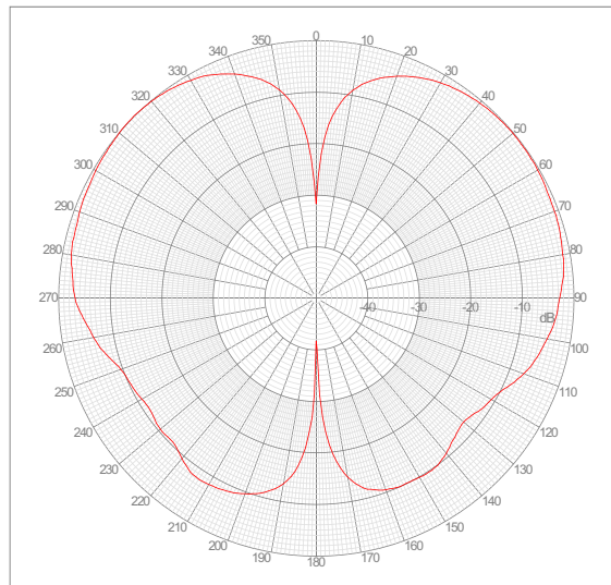
5.875 GHz E-Plane
