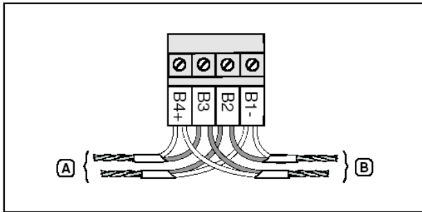
Fig. 5 : Wiring E-Bus
