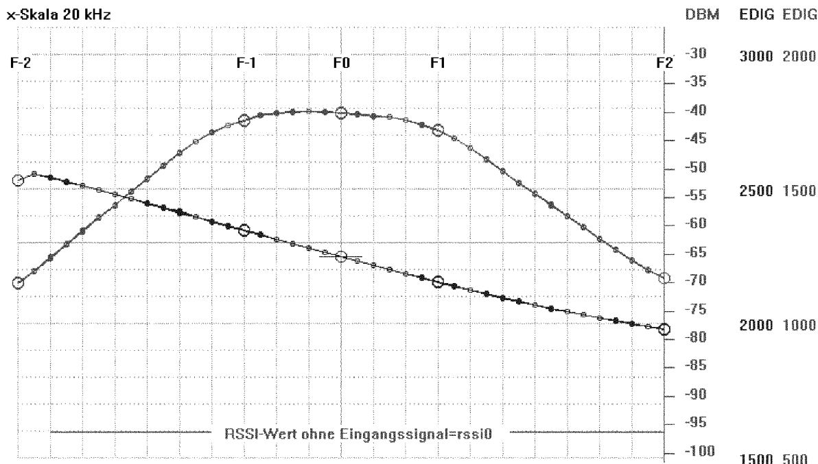
Bild 3: Selektions- und Diskriminatorkurve des Funkmodul-Empfängers
