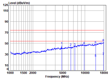
Right BT_DH5_TX_CH_39_Horizontal
