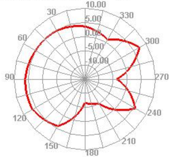
Bluetooth 39 TRP E1
