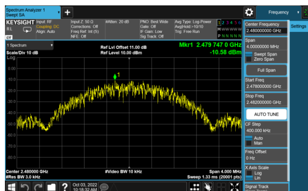
CH78 (2480MHz)
