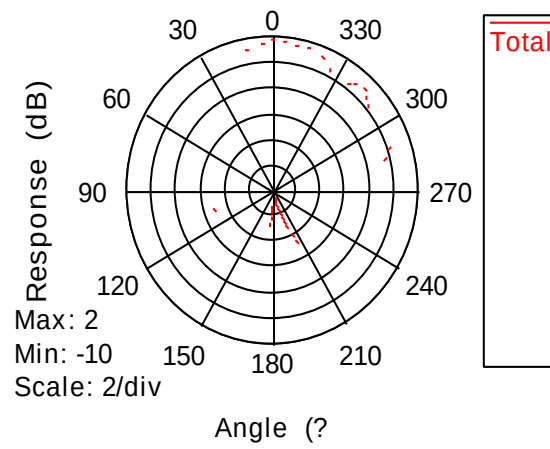
H-Plane
