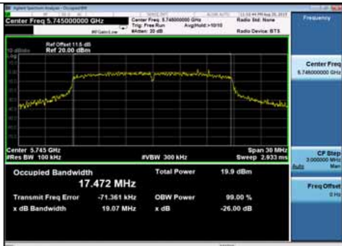
5745MHz
