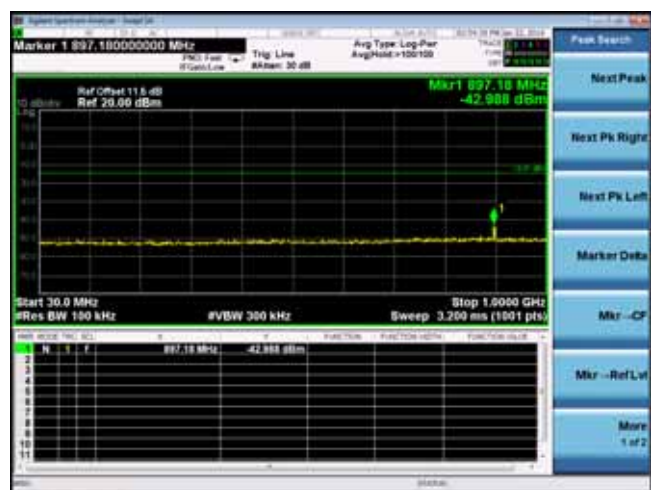
2402MHz(30MHz – 1GHz)
