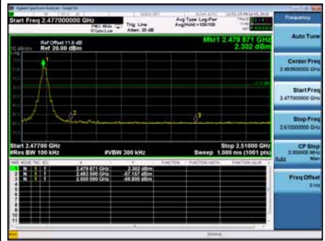
2480MHz(2.4GHz – 2.5GHz)
