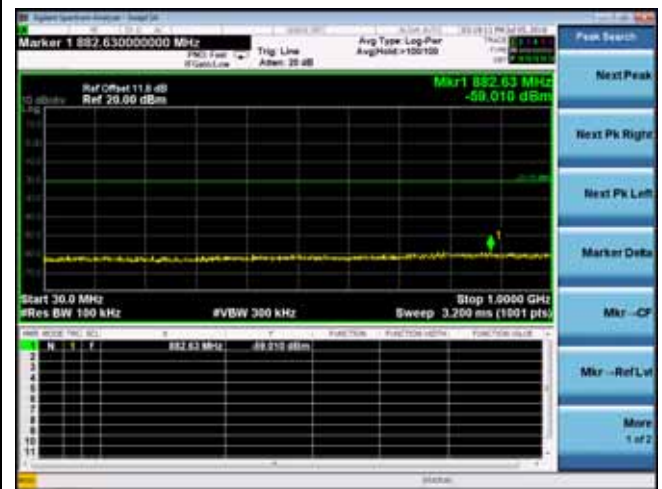
2402MHz(30MHz – 1GHz)
