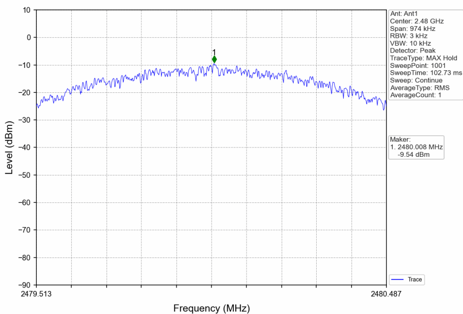
1M_HCH_2480MHz_DataRate=_Ant1_NTNV
