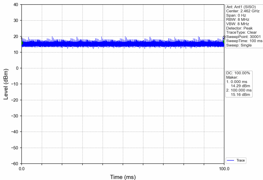
802.11g_HCH_2462MHz_Ant1 (SISO)_NTNV
