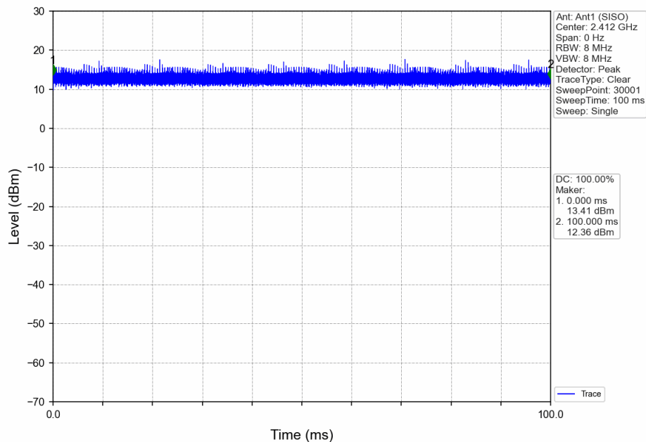
802.11g_LCH_2412MHz_Ant1 (SISO)_NTNV
