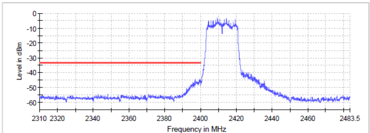
Band Edge
