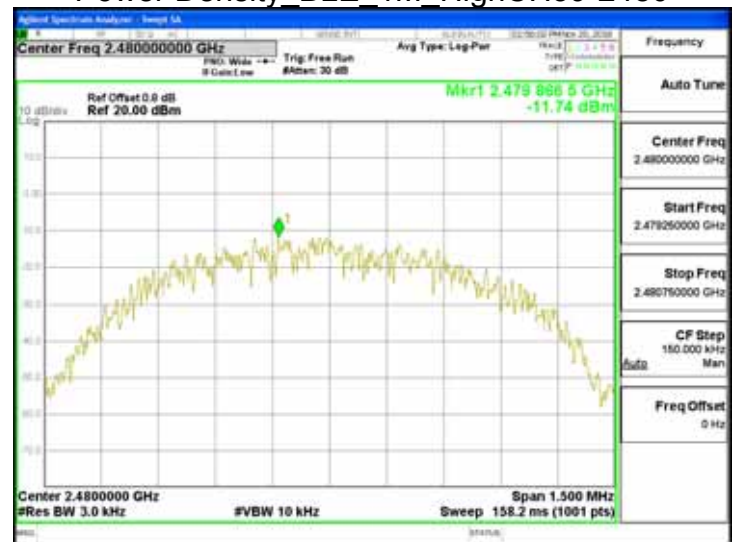
Power Density BLE 1M HighCH39-2480
