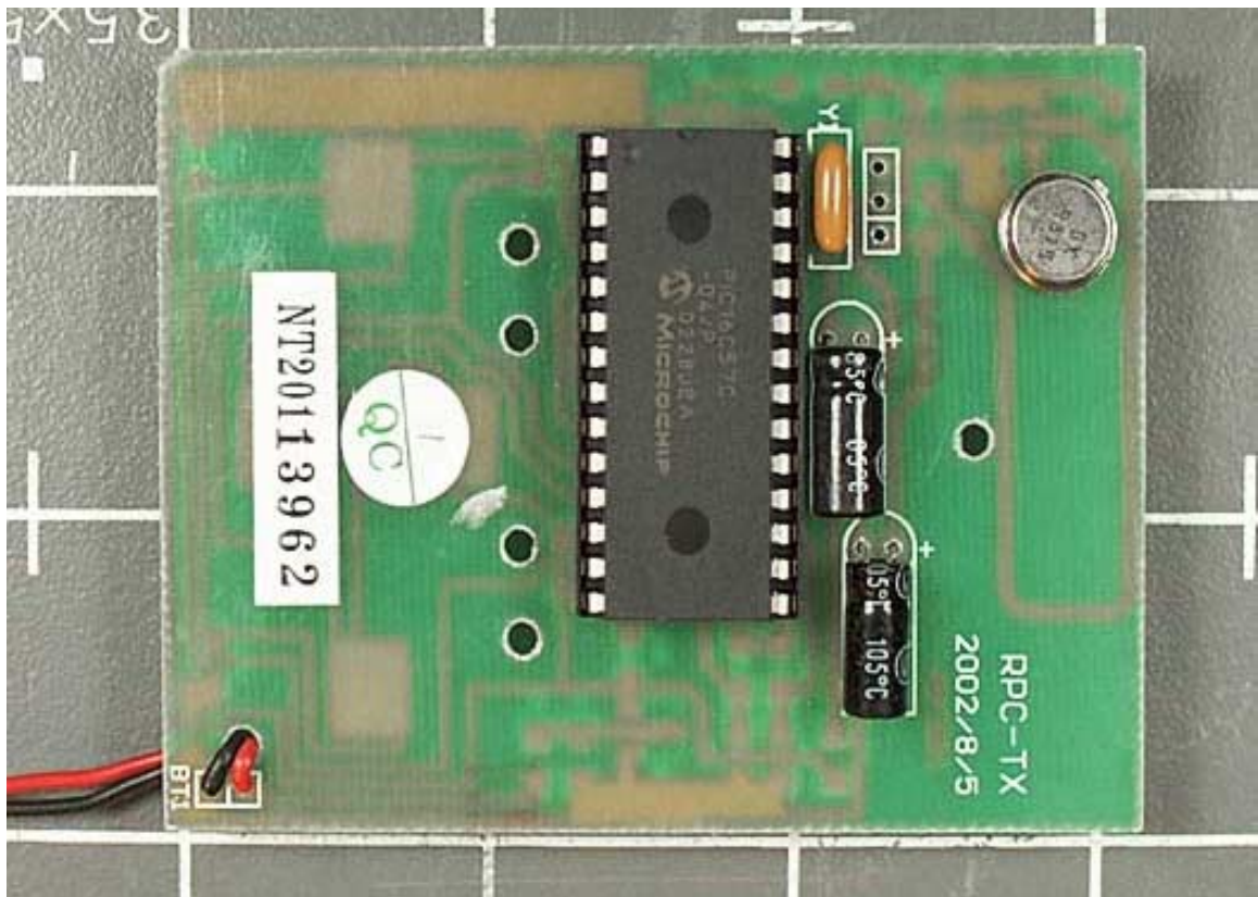
PCB Bottom
