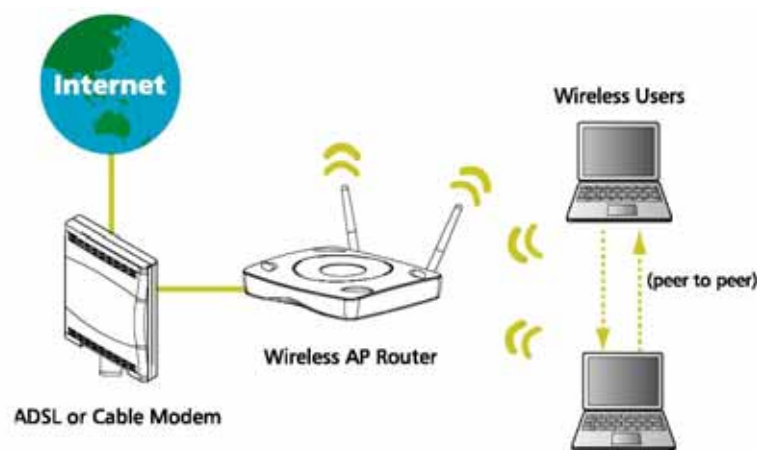
Ad-hoc Mode
