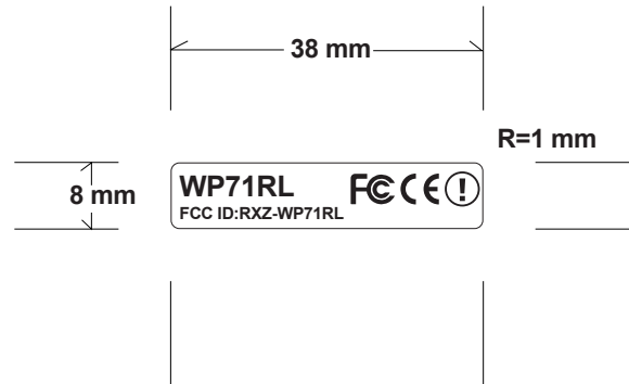
〈尺寸圖〉
