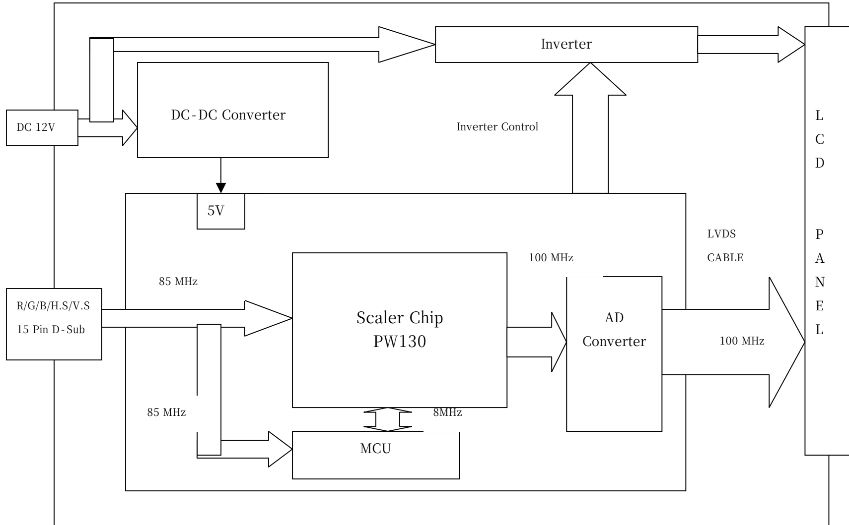
EFL-1903X Block Diagram
