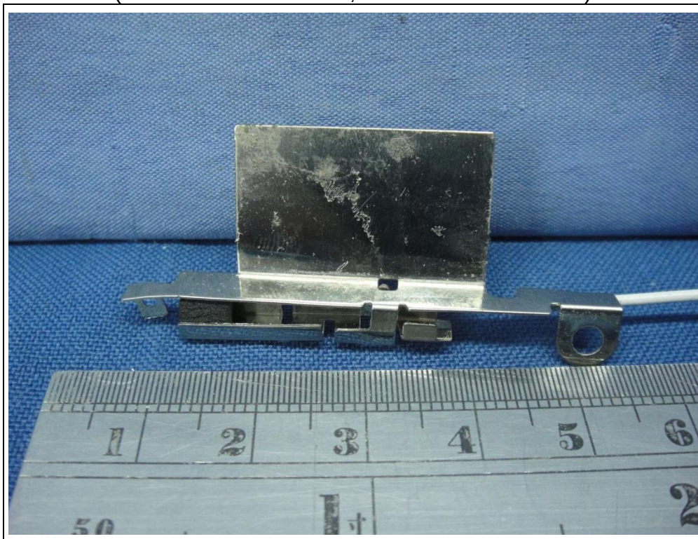
Antenna set 1 (Chain 1 / Brand : WNC, Model : 81-EBJ15.005)
