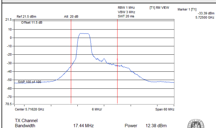
802.11ax (HE20) RU52 / Chain 1 : CH 144 (U-NII-2C)
