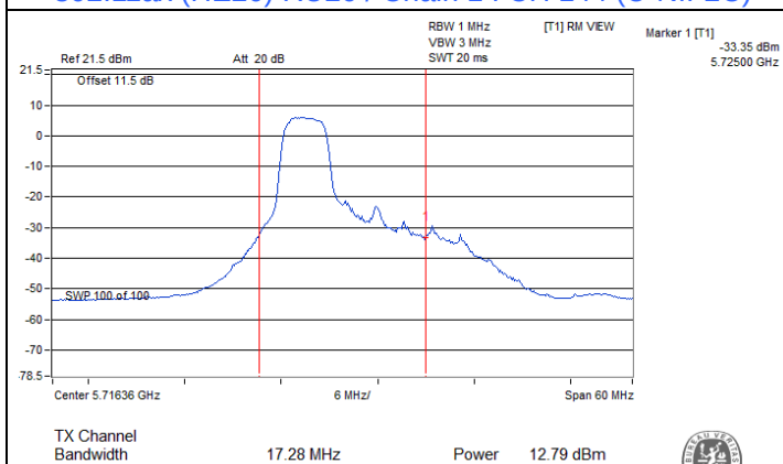
802.11ax (HE20) RU26 / Chain 1 : CH 144 (U-NII-2C)
