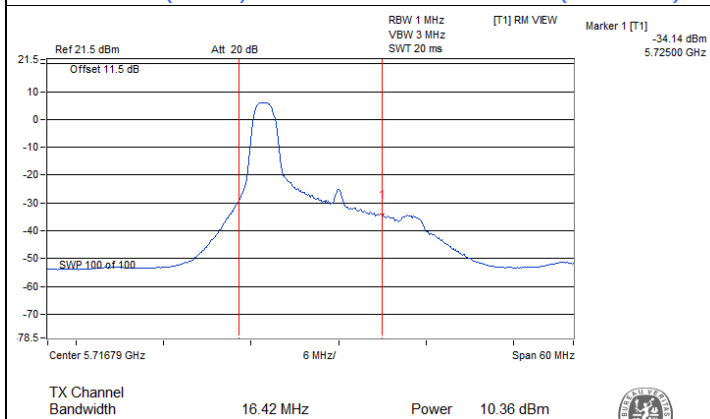
802.11ax (HE20) RU26 / Chain 0 : CH 144 (U-NII-2C)
