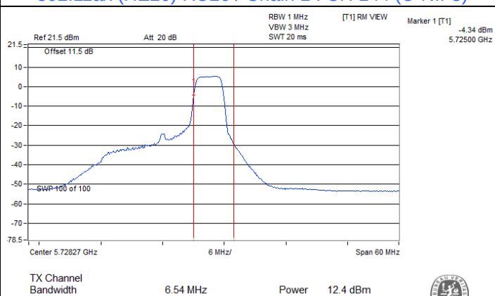
802.11ax (HE20) RU26 / Chain 1 : CH 144 (U-NII-3)
