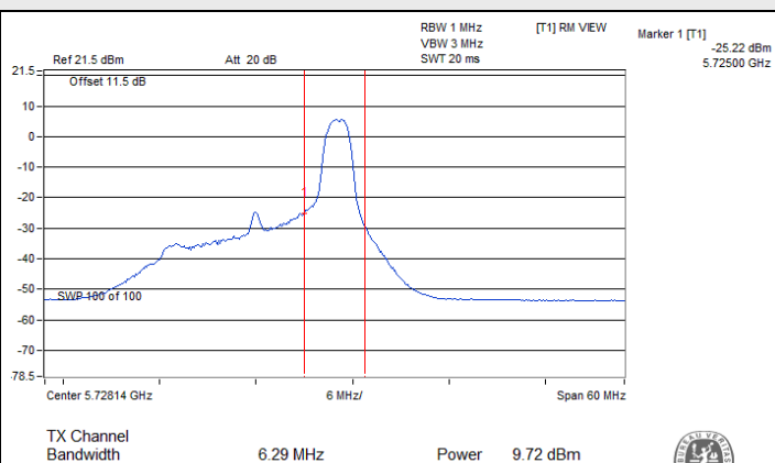
802.11ax (HE20) RU26 / Chain 0 : CH 144 (U-NII-3)
