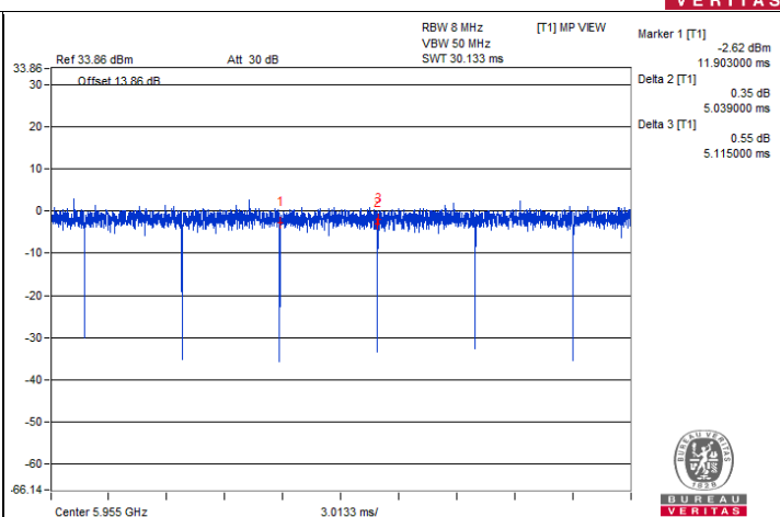
802.11be (EHT20) 52-tone RU
