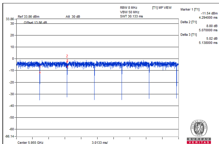
802.11be (EHT20) 26-tone RU
