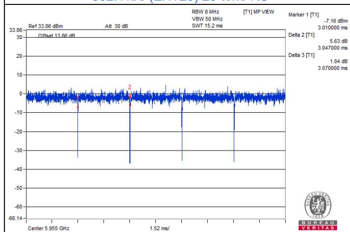
802.11be (EHT20) 106-tone RU
